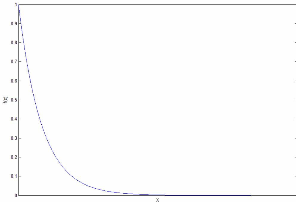
Figura 24 - Curva exponencial f(x)
