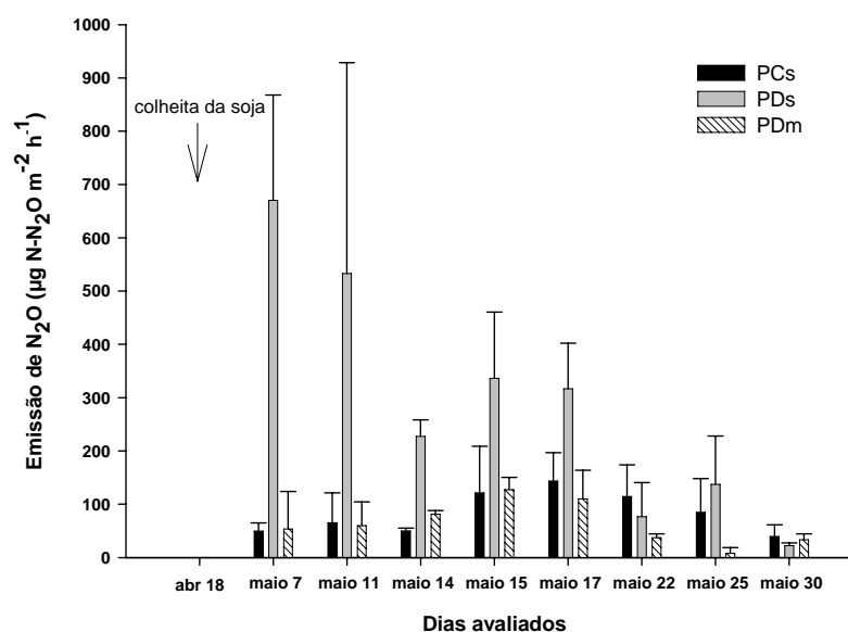
Figura 14. Emissões de N_2O nos sistemas de preparo do solo convencional e plantio direto em sistemas de rotação de culturas sob Latossolo Vermelho distrófico típico no período de 07/05/07 a 30/05/07. Rotação 1-3 (PCs e PDs): Aveia/soja/aveia+ervilhaca/milho/nabo/trigo/soja; Rotação 1-2 (PDm): Aveia+ervilhaca/milho/nabo/trigo/soja/aveia/soja. As barras verticais representam o desvio padrão da média.
