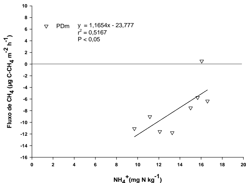
Figura 23. Relação entre o fluxo de CH 4 com a concentração de amônio (NH 4 + ) no plantio direto em sistema de rotação de culturas sob Latossolo Vermelho distrófico típico no período de 07/05/07 a 30/05/07. Rotação 1-2 (PDm): Aveia+ervilhaca/milho/nabo/trigo/soja/aveia/soja.
