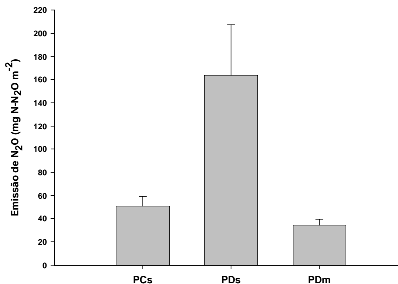
Figura 21. Emissões totais de N 2 O nos sistemas de preparo do solo convencional e plantio direto em sistemas de rotação de culturas sob Latossolo Vermelho distrófico típico no período de 07/05/07 a 30/05/07. Rotação 1-3 (PCs e PDs): Aveia/soja/aveia+ervilhaca/milho/nabo/trigo/soja; Rotação 1-2 (PDm): Aveia+ervilhaca/milho/nabo/trigo/soja/aveia/soja. As barras verticais representam o desvio padrão da média.
