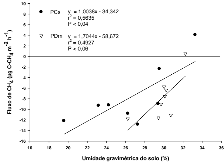
Figura 24. Relação entre o fluxo de CH 4 com umidade gravimétrica nos sistemas de preparo do solo convencional e plantio direto em sistemas de rotação de culturas sob Latossolo Vermelho distrófico típico no período de 07/05/07 a 30/05/07. Rotação 1-3 (PCs): Aveia/soja/aveia+ervilhaca/milho/nabo/trigo/soja; Rotação 1-2 (PDm): Aveia+ervilhaca/milho/nabo/trigo/soja /aveia/soja.
