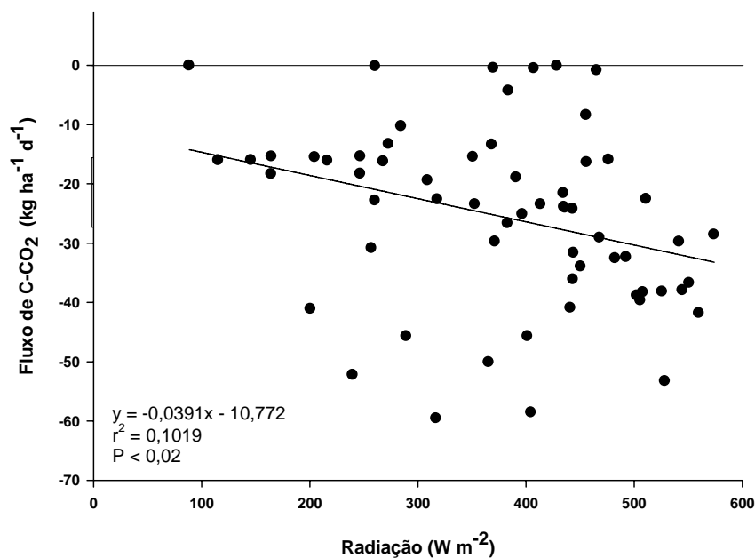
Figura 11. Relação entre o fluxo de C-CO 2 com a radiação solar no ciclo da cultura da soja.
