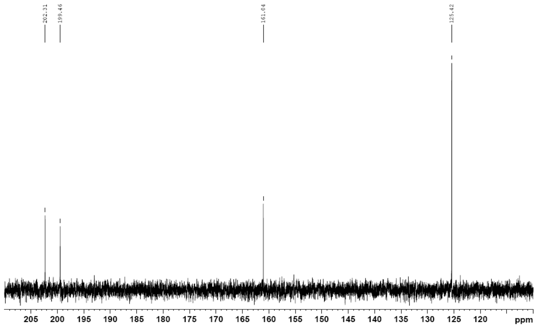
Espectro expandido de RMN ^{13}\text{C} da substância S1A em \text{CDCl}_3 , região entre 210 e 105 ppm.
