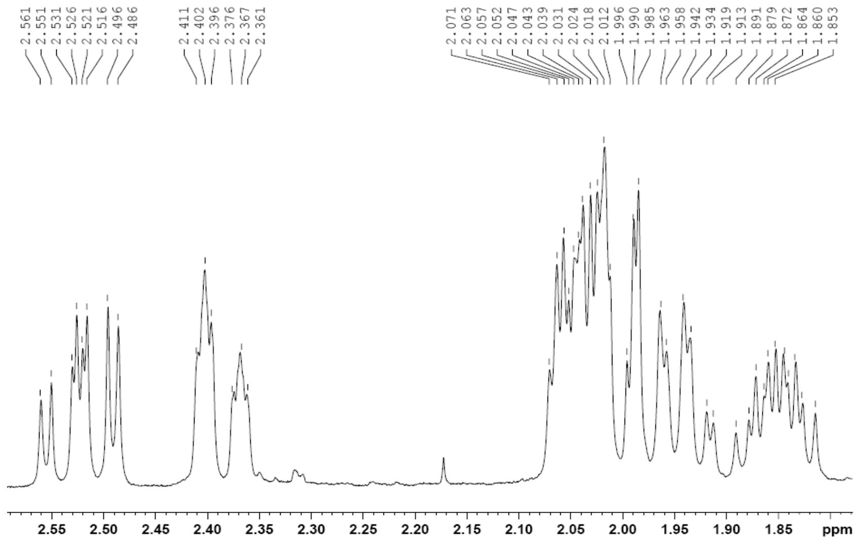
Espectro expandido de RMN ^1\text{H} da substância S2A em \text{CDCl}_3 , região entre 2,6 e 1,8 ppm.
