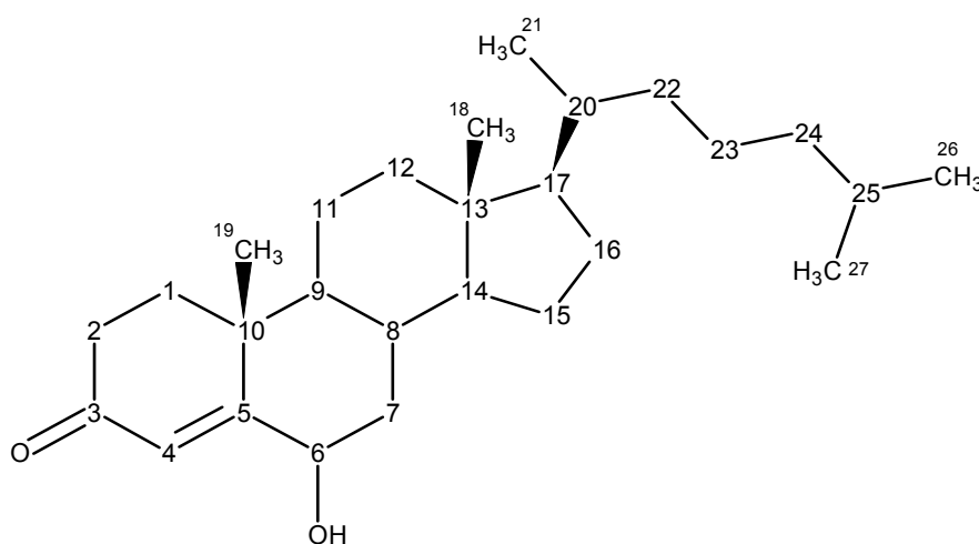
Figura 27: Estrutura proposta para a substância S2A, 6 \beta -hidroxi-colest-4-en-3-ona.
