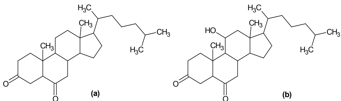
Figura 8: Estrutura da 5\alpha -colestano-3,6-diona e da 11\alpha -hidroxi- 5\alpha -colestano-3,6-diona.
