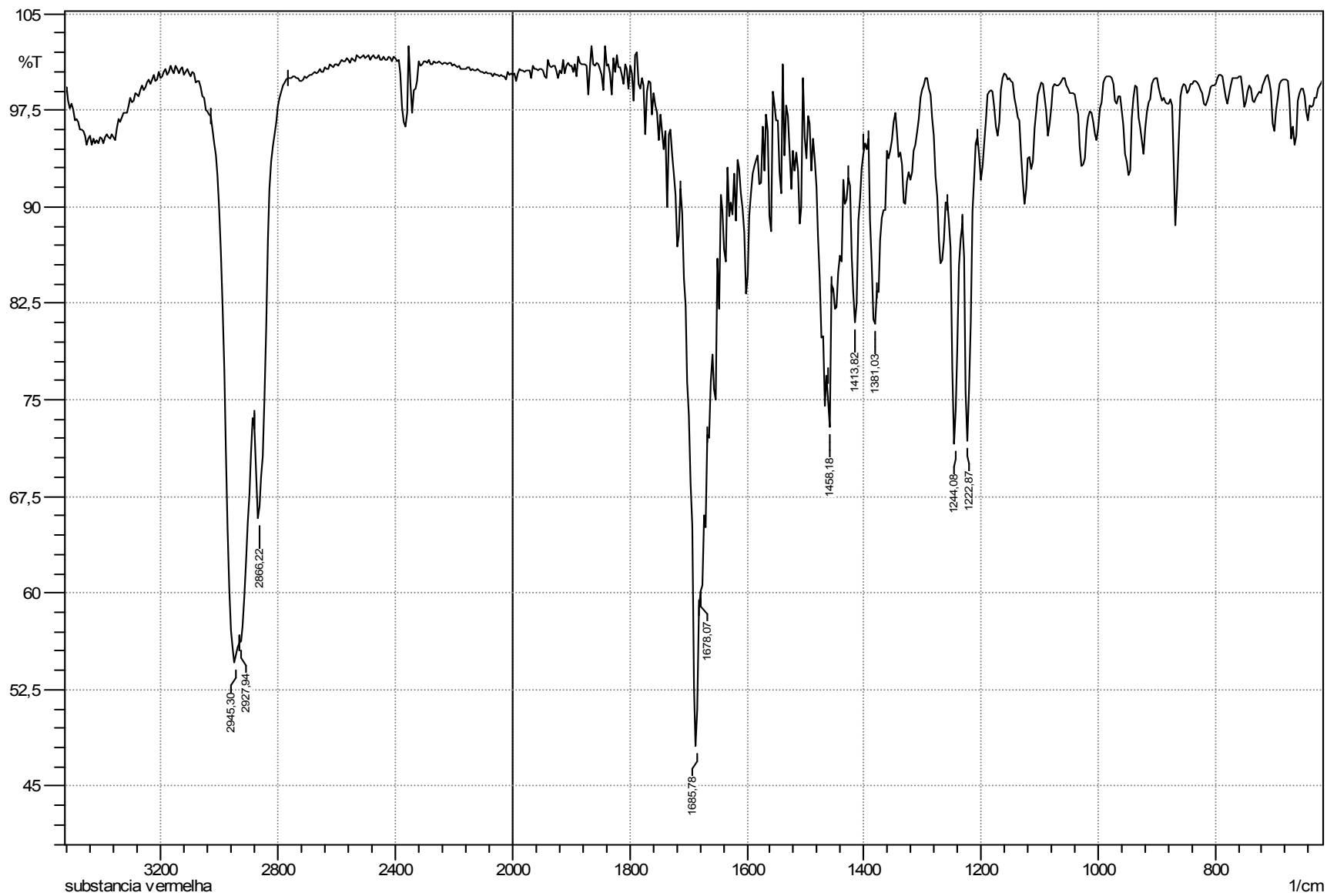
Espectro de IR da substância S1A, em pastilhas de KBr.
