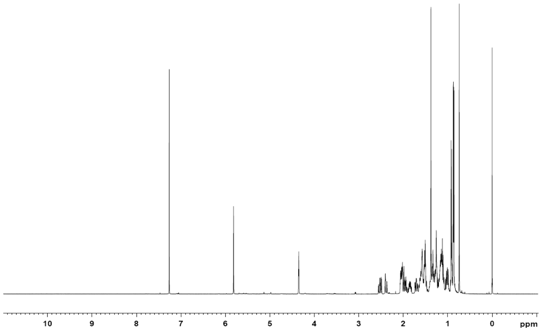
Espectro RMN ^1\text{H} da substância S2A em \text{CDCl}_3 .
