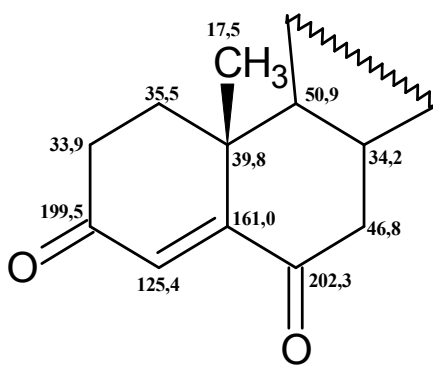
Figura 21: Estrutura parcial de S1A: atribuições dos deslocamentos químicos de ^{13}\text{C} para os carbonos dos anéis A e B.
