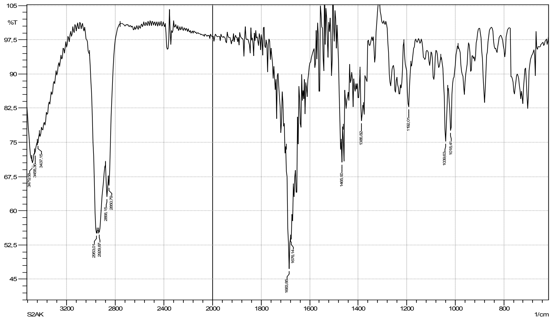
Espectro de IR da substância S2A, em pastilhas de KBr.
