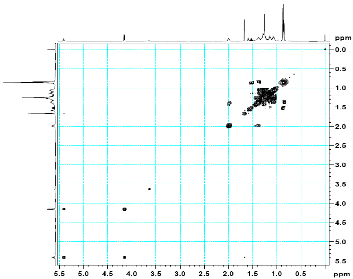
Espectro ^1\text{H} ^1\text{H} -COSY da substância S5A em \text{CDCl}_3
