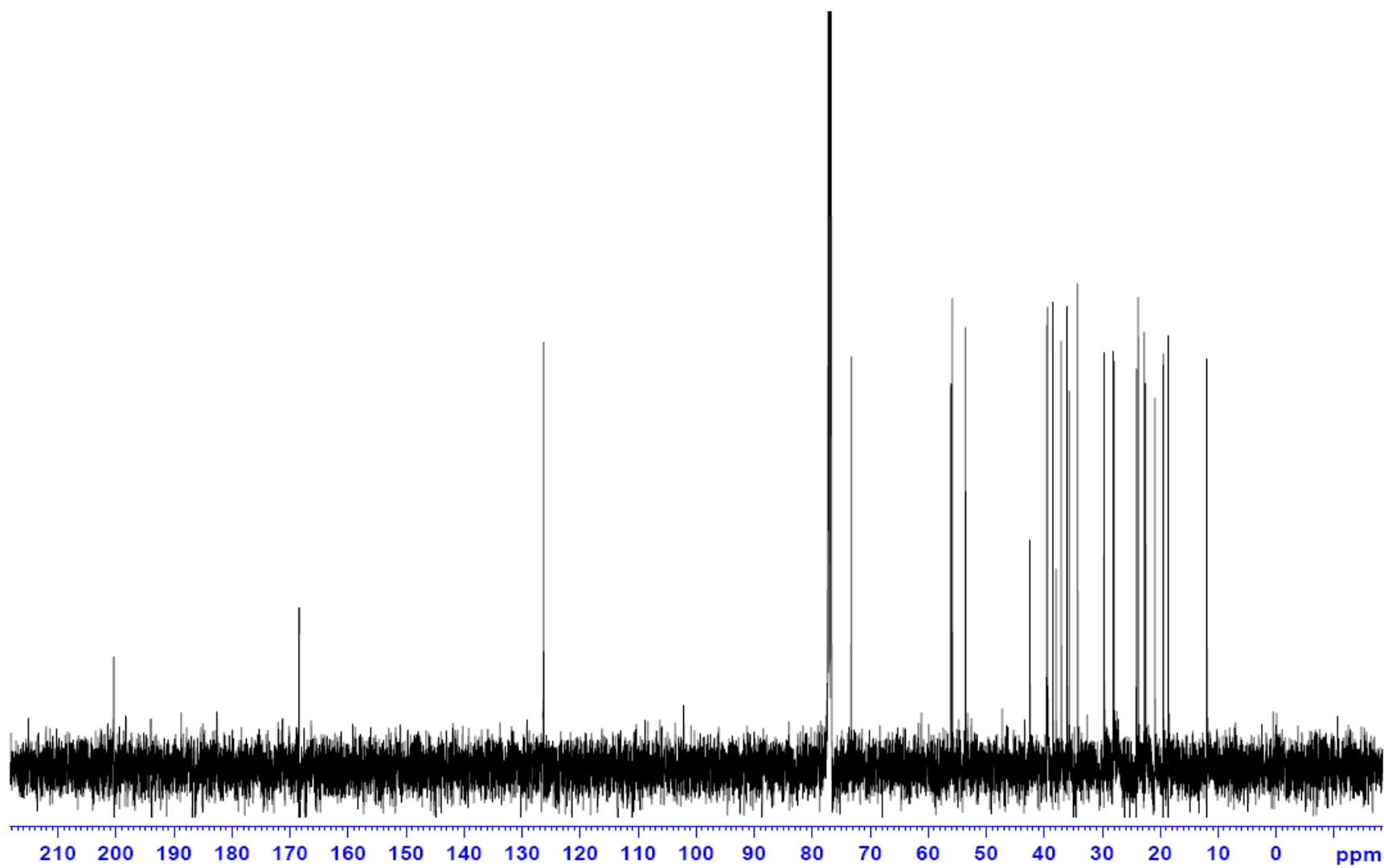
Espectro de RMN ^{13}\text{C} da substância S2A em \text{CDCl}_3 .
