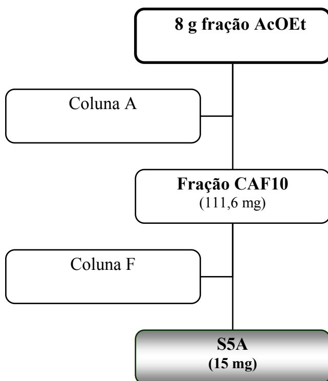
Figura 12: Representação esquemática do isolamento da substância S5A de A. spicifera .
