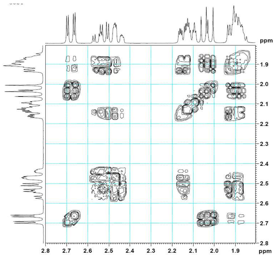
Espectro expandido ^1\text{H} - ^1\text{H} -COSY da substância S1A em \text{CDCl}_3 , região entre 2,8 e 1,8 ppm.
