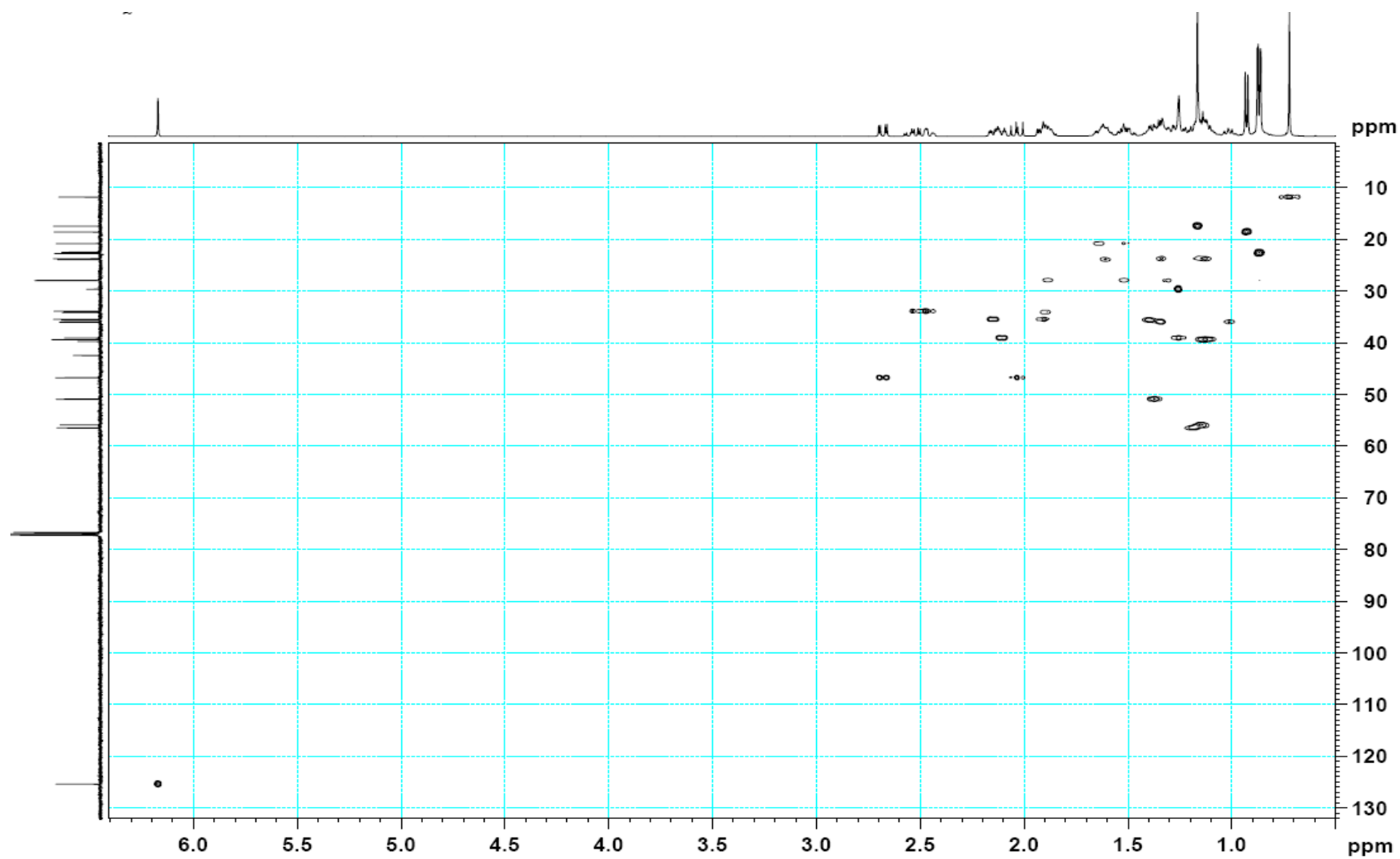
Espectro HSQC da substância S1A em CDCl 3
