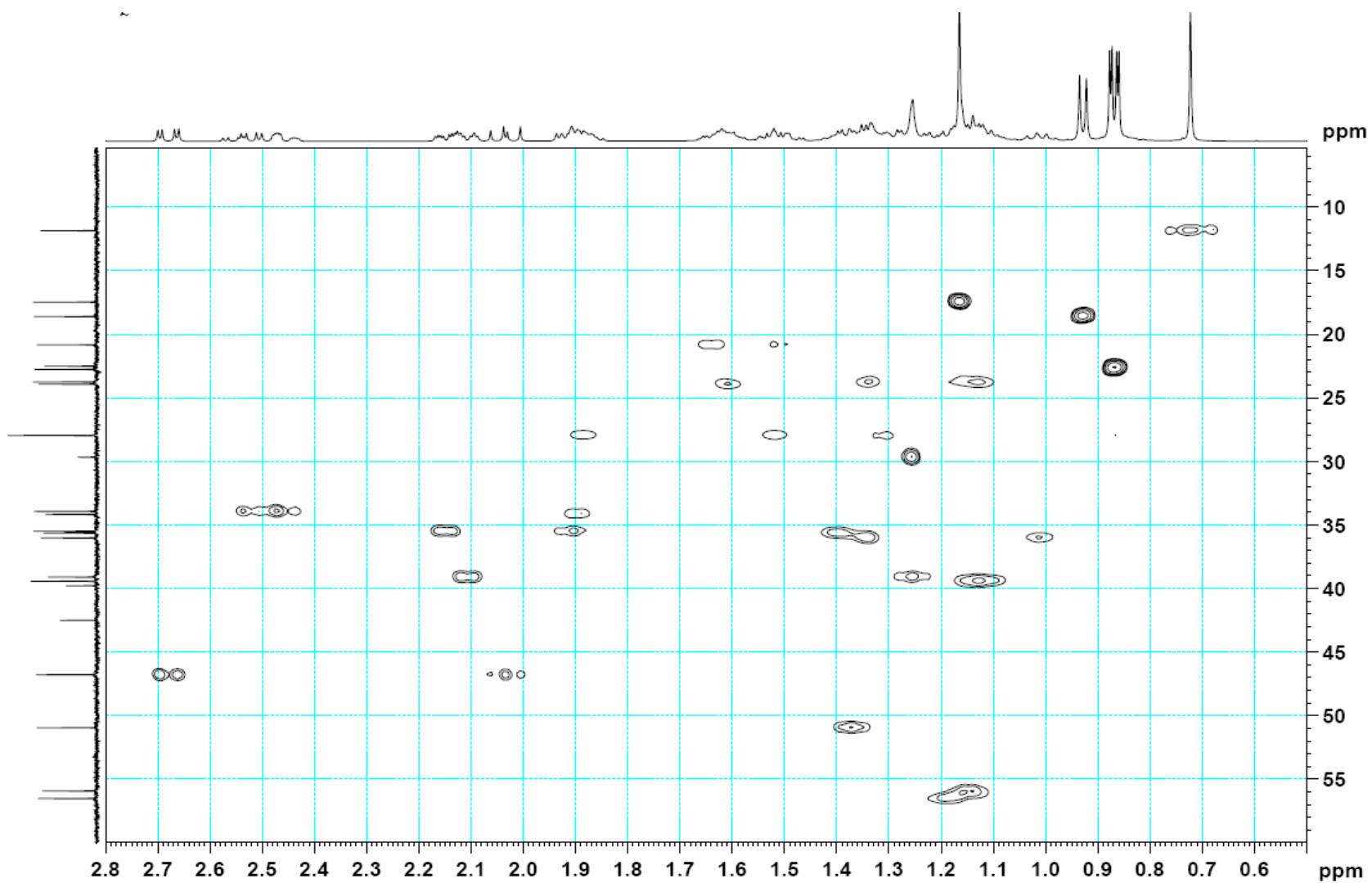
Espectro expandido HSQC da substância S1A em CDCl 3 , região entre 2,8 e 0,5 ppm.
