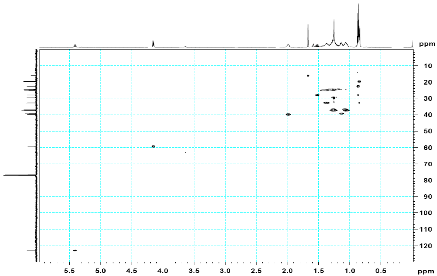
Espectro HSQC da substância S5A em \text{CDCl}_3
