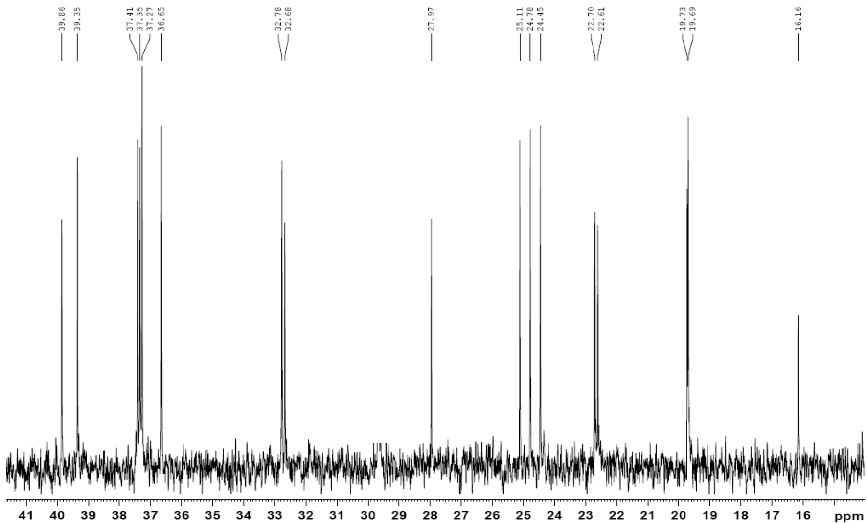
Espectro expandido de RMN ^{13}\text{C} da substância S5A em \text{CDCl}_3 , região entre 42 e 14 ppm.
