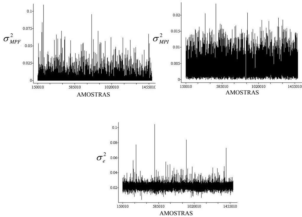
FIGURA 20A – Diagnóstico de convergência para as variâncias genéticas oligogênicas e poligênicas ( \sigma_{MPF}^2 e \sigma_{MPI}^2 ) e da variância do erro ( \sigma_e^2 ), para a característica relação carne:gordura (RCG), quando ajustado o modelo combinado (MPF + MPI).
