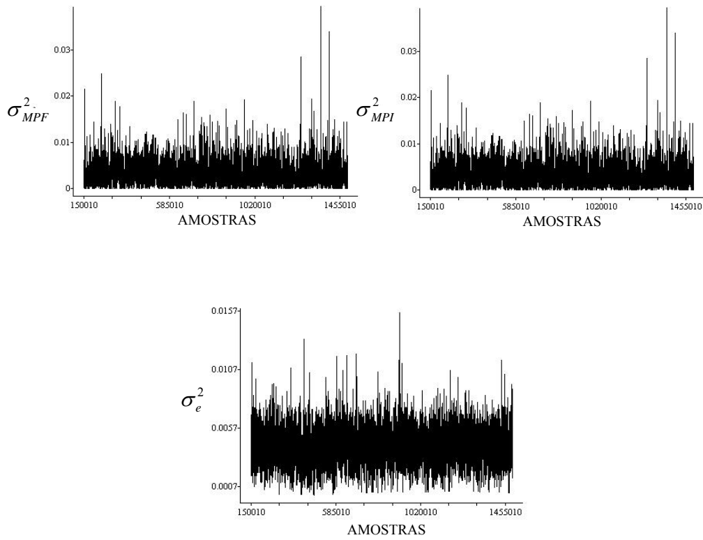
FIGURA 22A – Diagnóstico de convergência para as variâncias genéticas oligogênicas e poligênicas ( \sigma_{MPF}^2 e \sigma_{MPI}^2 ) e da variância do erro ( \sigma_e^2 ), para a característica relação peso da gordura/peso da carne (RGC), quando ajustado o modelo combinado (MPF + MPI).
