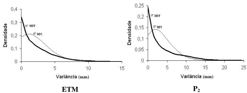
FIGURA 4 – Distribuição marginal a posteriori para as variâncias genéticas estimadas no MPF ( \sigma_{MPF}^2 ) e no MPI ( \sigma_{MPI}^2 ) para as características espessura de toucinho média (ETM) e espessura de toucinho a 6,5cm da linha do dorso (P 2 ).
