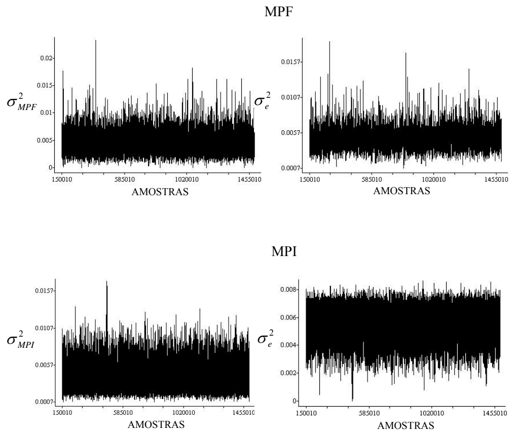
FIGURA 21A – Diagnóstico de convergência para as variâncias genéticas oligogênicas e poligênicas ( \sigma^2_{MPF} e \sigma^2_{MPI} ) e da variância do erro ( \sigma_e^2 ), para a característica relação peso da gordura/peso da carne (RGC), quando ajustado o modelo poligênico finito (MPF) e modelo poligênico infinitesimal (MPI).
