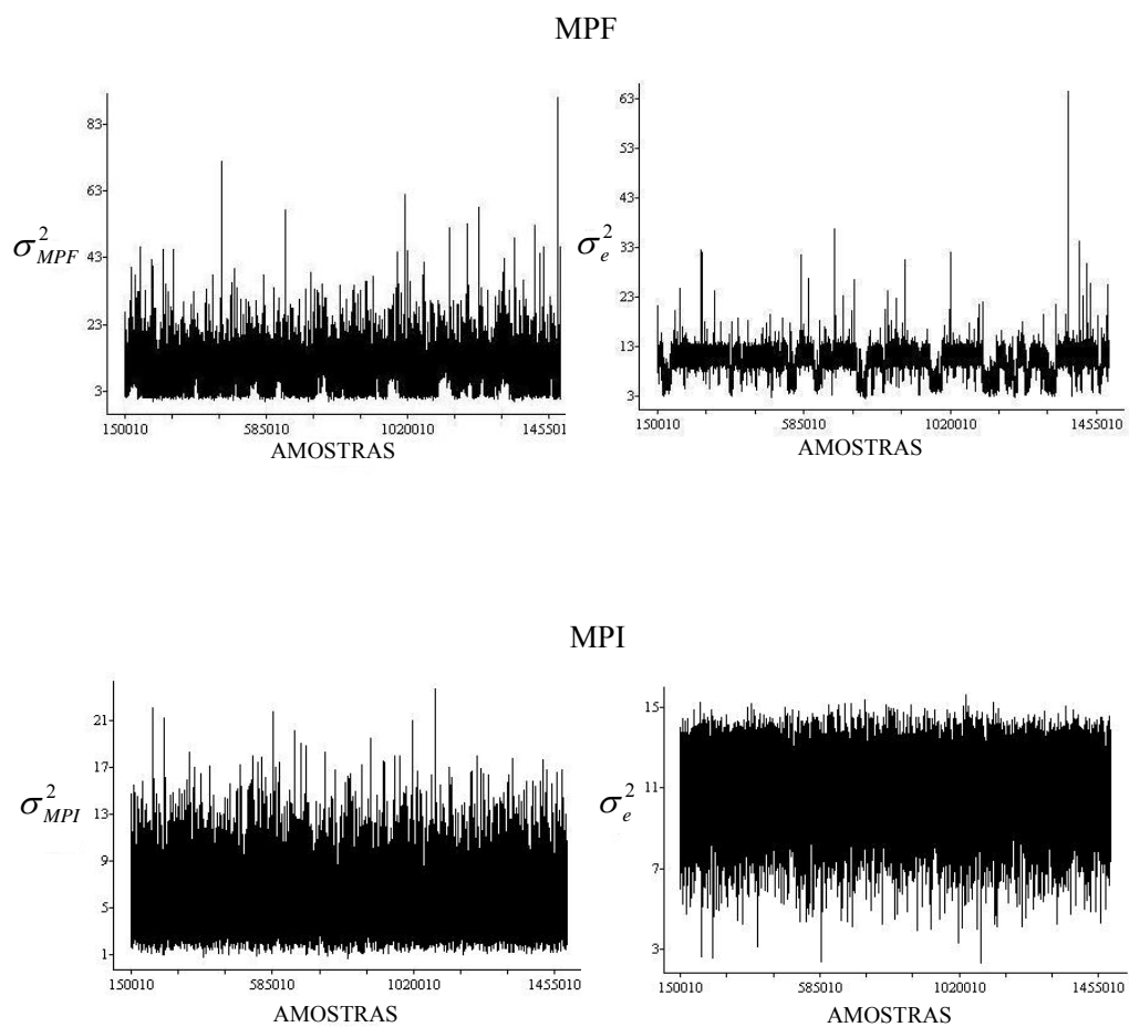
FIGURA 1A – Diagnóstico de convergência para as variâncias genéticas oligogênicas e poligênicas ( \sigma_{MPF}^2 e \sigma_{MPI}^2 ) e da variância do erro ( \sigma_e^2 ), para a característica área de olho de lombo (AOL), quando ajustado o modelo poligênico finito (MPF) e o modelo poligênico infinitesimal (MPI).
