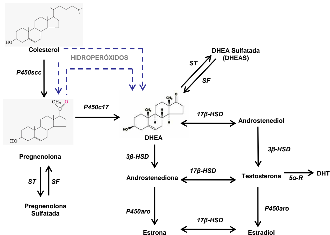
Figura 2: Síntese e metabolização da DHEA no sistema nervoso.
