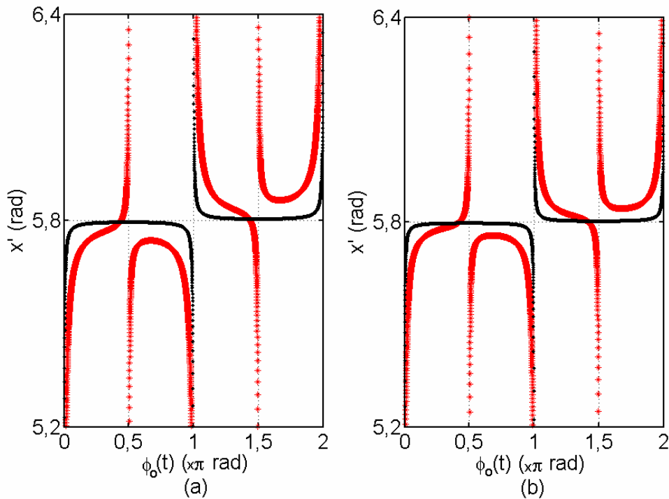
Figura 5.9 - Índice de modulação de fase x' em função da fase \phi_0(t) para o valor esperado x = 5,8 rad, calculado usando os métodos (*) J_1...J_6 -pos e (●) J_1...J_3 , considerando o fator de ruído K . (a) Ruído 1/f^2 com K=0,0011 . (b) Ruído branco com K=0,0004 .
