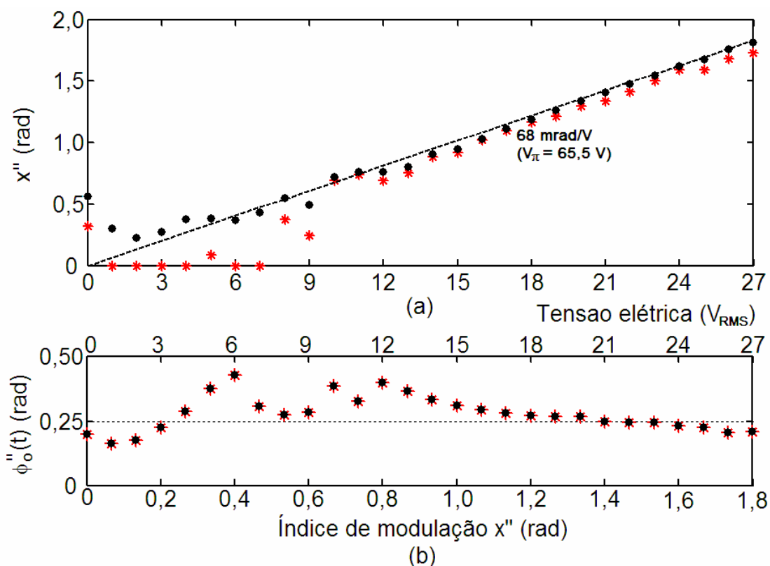
Figura 7.7 – Cálculos realizados para o SOT excitado por uma tensão senoidal variando de 0 a 27 V. (a) Profundidade de modulação de fase estimada usando-se os métodos: (*) J_1...J_6 -neg, e (●) J_1/J_3A . (b) Fase \phi_0(t) calculada pelo: (*) método desenvolvido por Sudarshanam e (●) novo método proposto nesta tese.
