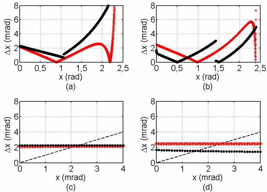
Figura 5.17 – Erro absoluto \Delta x em função de x usando os métodos (*) J_0 \dots J_2 e (•) J_0 \dots J_3 , considerando x_a = 2,7 rad e \phi_0(t) = \pi/4 rad. (a) Ruído 1/f^2 com K=0,0011 . (b) Ruído branco com K=0,0004 . (c) Ruído 1/f^2 com K=0,0011 (região de baixos índices). (d) Ruído branco com K=0,0004 (região de baixos índices).
