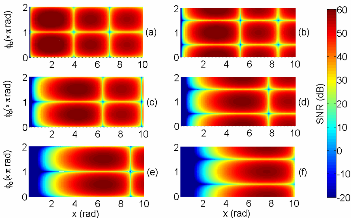
Figura 3.10 – SNR para ruído branco com K=0,0004 . (a) componente fundamental. (b)-(f) segunda a sexta harmônicas, respectivamente.
