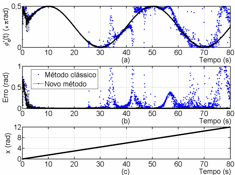
Figura 6.31 – Respostas do subsistema de cálculo de \phi'_o(t) em função do tempo, para x e \phi_o(t) variando. (a) (●) Cálculo pelo método desenvolvido por Sudarshanam (clássico) e (●) cálculo pelo novo método. (b) Erro absoluto no cálculo de \phi'_o(t) usando (●) o método desenvolvido por Sudarshanam (clássico) e (●) o novo método. (c) Índice de modulação x .
