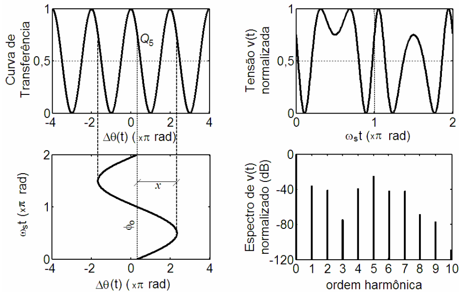
Figura 3.8 – Tensão fotodetectada v(t) e seu espectro de magnitude em dB (até a décima harmônica), normalizados, para uma excitação \Delta\phi = x \text{ sen}(\omega_s t) , considerando visibilidade unitária, e regime multifranjas, com índice de modulação x = 2\pi rad e ponto quiescente Q_5 , [ \phi_0(t) = \pi/3 rad].
