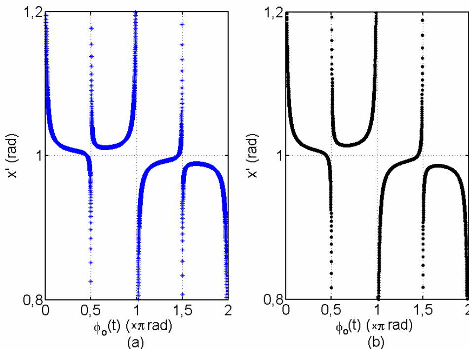
Figura 4.3 - Fase estimada x' em função da fase \phi_0(t) para o valor esperado x = 1 rad, pela aplicação do método J_1...J_4 . (a) Simulação para ruído 1/f^2 com K=0,0011 . (b) Simulação para ruído branco com K=0,0004 .
