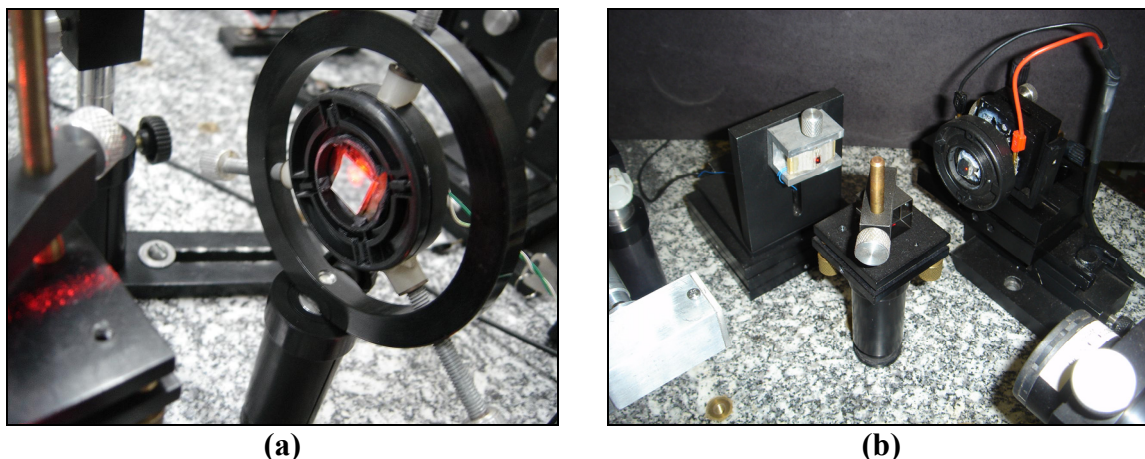
Figura 8.16 – (a) Detalhe do tweeter usado no interferômetro para uso específico dos métodos J_0\dots J_2 e J_0\dots J_3 . (b) Interferômetro de Michelson modificado em seu braço de referência, pelo uso do tweeter .
