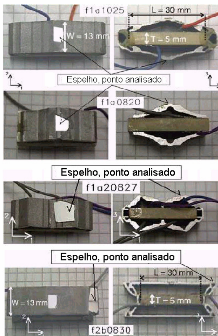
Figura 2.7 – Piezoatuadores flexensionais com diferentes topologias, dependendo do ponto em que se deseja amplificar a vibração [143].
