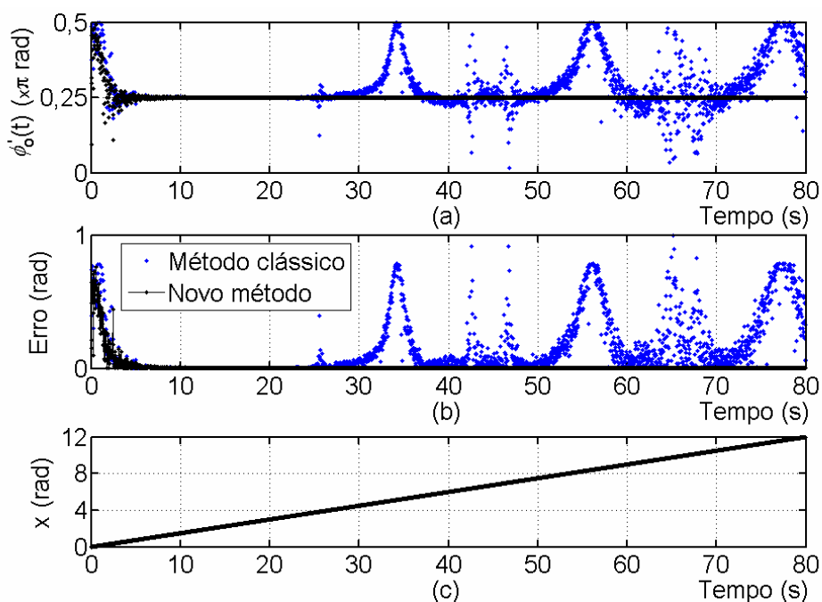
Figura 6.30 – Respostas do subsistema de cálculo de \phi'_o(t) em função do tempo, para x variando e \phi_o(t) = \pi/4 rad. (a) (●) Cálculo pelo método desenvolvido por Sudarshanam (clássico) e (●) cálculo pelo novo método. (b) Erro absoluto no cálculo de \phi'_o(t) usando (●) o método desenvolvido por Sudarshanam (clássico) e (●) o novo método. (c) Índice de modulação x .
