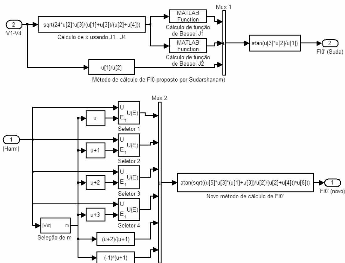
Figura 6.11 – Subsistema de cálculo de \phi_0(t) usando os métodos espectrais.
