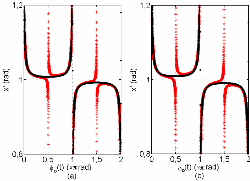
Figura 5.3 – Índice de modulação de fase estimado x' em função da fase \phi_0(t) para o valor esperado x=1 rad, pela aplicação dos métodos (*) J_1\dots J_4 e (•) J_1/J_3A , considerando o fator de ruído K . (a) Ruído 1/f^2 com K=0,0011 . (b) Ruído branco com K=0,0004 .
