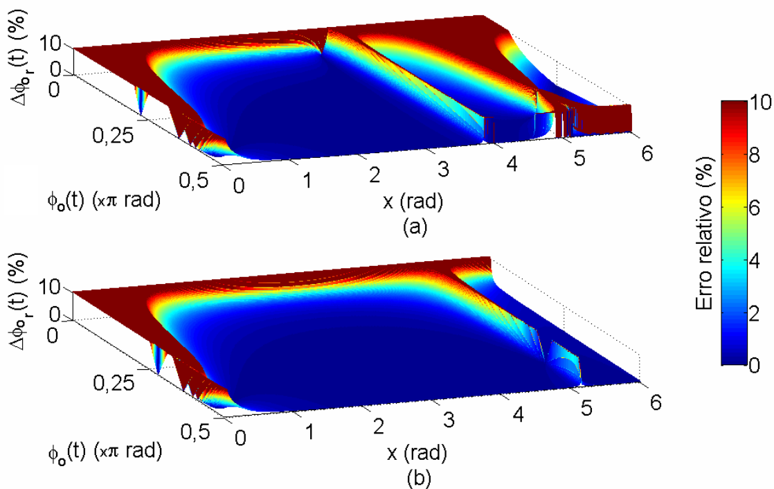
Figura 5.23 – Erro percentual relativo \Delta\phi_0(t)_r , em função de x e \phi_0(t) , simulado com ruído branco e K=0,0004 , para: (a) o método proposto por Sudarshanam e (b) o novo método direto de medição de \phi_0(t) , calculado usando (5.49).
