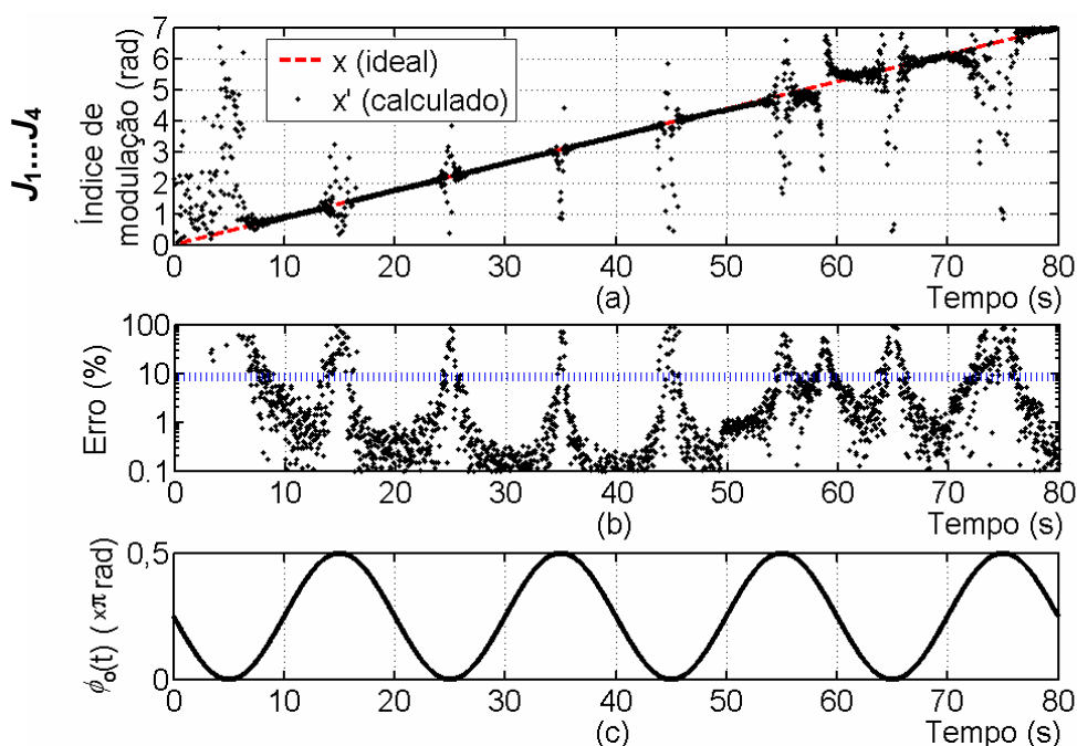
Figura 6.25 – Resposta do subsistema de cálculo de x pelo método J_1...J_4 , para x e \phi_0(t) variando. (a) Índice estimado x' . (b) Erro \Delta x , na estimativa de x . (c) Fase \phi_0(t) .
