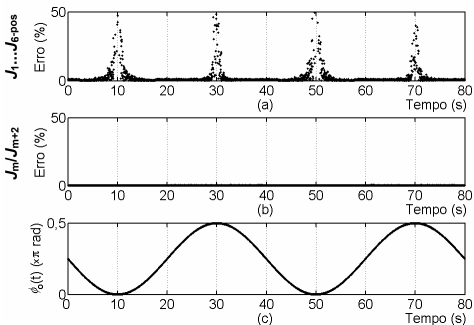
Figura 6.21 – Respostas dos subsistemas de cálculo de x' em função do tempo, para x=5,5 rad e \phi_0(t) variando. (a) Erro \Delta x_r pelo método J_1...J_6 -pos. (b) Erro \Delta x_r pelo método J_m/J_{m+2} . (c) Fase \phi_0(t) .
