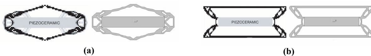
Figura 2.6 - Resultados de otimização topológica e a interpretação correspondente [155]. a) Deslocamento máximo no centro do encapsulamento metálico. b) Deslocamento máximo na extremidade do encapsulamento.
