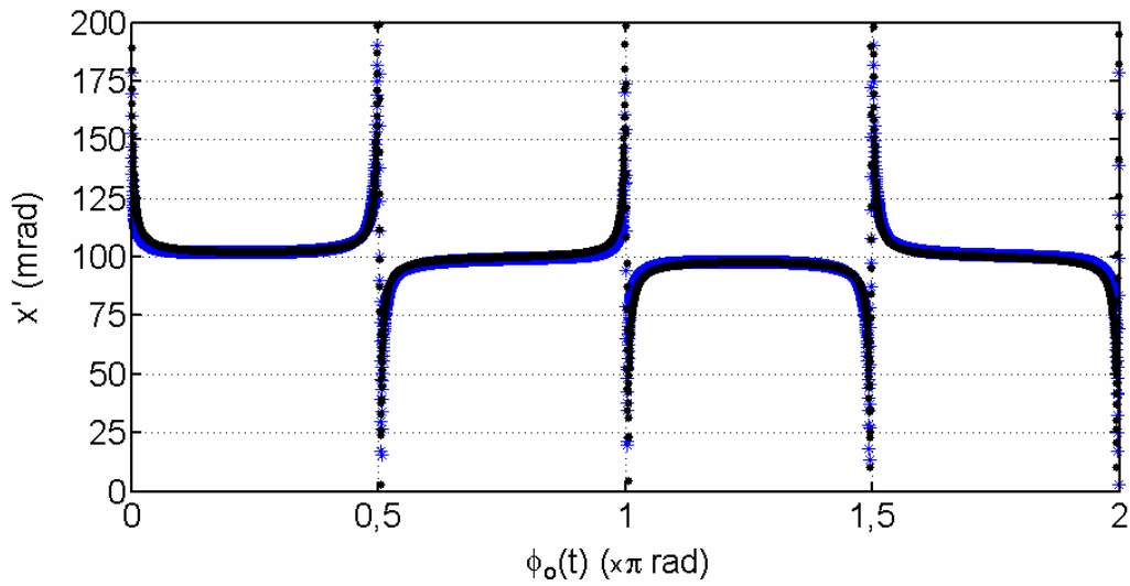
Figura 4.12 - Fase estimada x' em função da fase \phi_0(t) para o valor esperado x = 100 mrad, pela aplicação do método J_0...J_2 , considerando (*) ruído 1/f^2 com K=0,0011 e (o) ruído branco com K=0,0004 .
