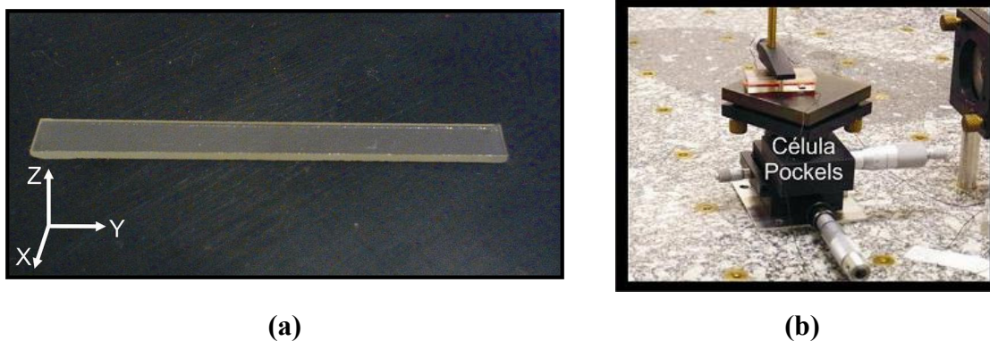
Figura 7.1 - Célula Pockels de \text{LiNbO}_3 empregada no SOT. (a) Cristal de \text{LiNbO}_3 utilizado como elemento sensor. (b) Célula Pockels transversal montada com o cristal num suporte.
