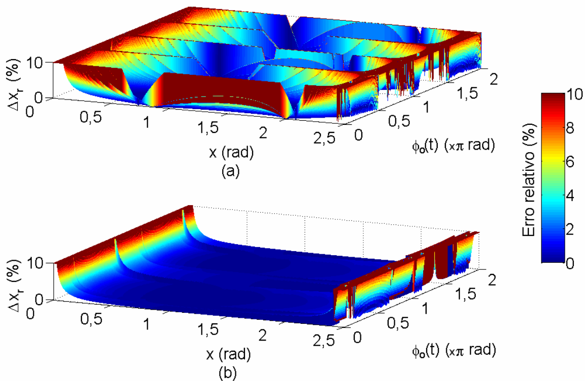
Figura 5.18 – Erro relativo de fase \Delta x_r , em função de x e \phi_0(t) , obtido em simulação com ruído branco e K=0,0004 , x_a = 2,5 rad. (a) Cálculo pelo método J_0...J_2 . (b) Cálculo pelo método J_0...J_3 .
