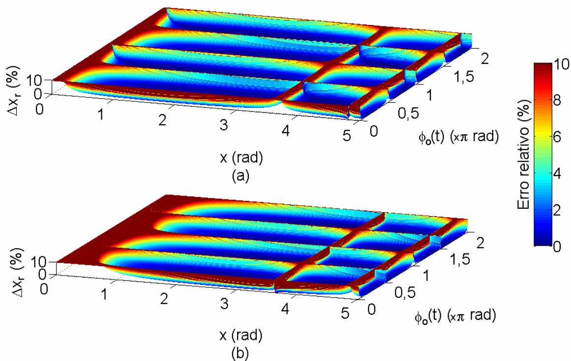
Figura 4.9 – Erro relativo de fase \Delta x_r como uma função de x e de \phi_0(t) , para o método J_1\dots J_6 -neg. (a) simulação para ruído 1/f^2 com K=0,0011 (b) simulação para ruído branco com K=0,0004 .
