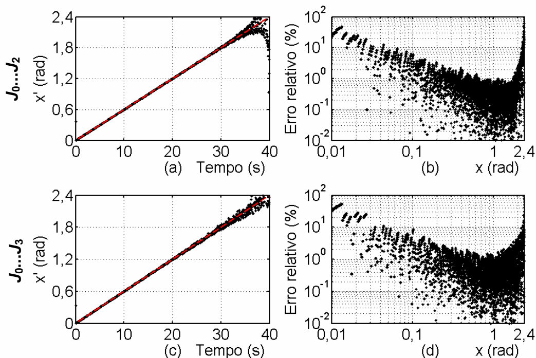
Figura 6.19 – Respostas dos subsistemas de cálculo de x' em função do valor esperado de x , para \phi_o(t)=\pi/4 rad. (a) \bullet x' pelo método J_0 \dots J_2 e -- valor esperado x . (b) Erro \Delta x_r , pelo método J_0 \dots J_2 . (c) \bullet x' pelo método J_0 \dots J_3 e -- valor esperado x . (d) Erro \Delta x_r , pelo método J_0 \dots J_3 .
