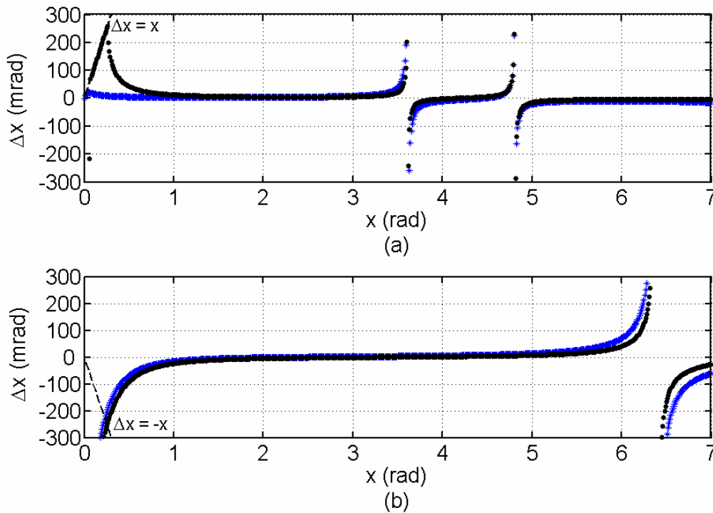
Figura 4.7 – Erro absoluto de fase \Delta x em função do valor esperado x para (*) ruído 1/f^2 com K=0,0011 e (●) ruído branco com K=0,0004 , onde a linha tracejada \pm x é utilizada para a identificação do MDPS; o valor de x correspondente a \Delta x = -x . (a) Método J_1 \dots J_6 -neg. (b) Método J_1 \dots J_6 -pos.
