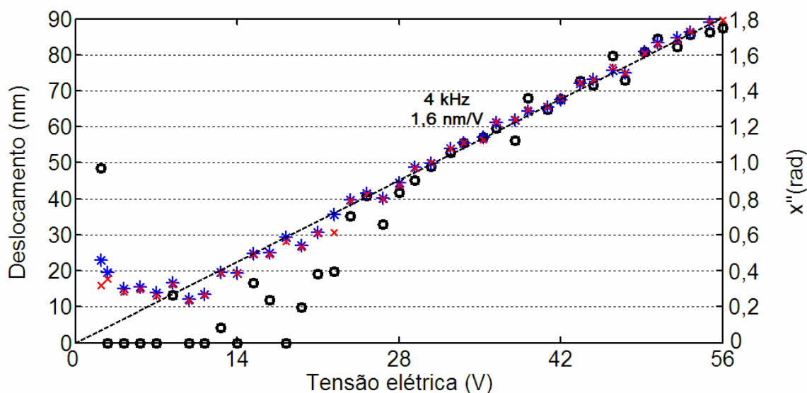
Figura 8.8 – Deslocamento \Delta l_s do APF obtido em análise harmônica, em 4 kHz, na região de baixo índice de modulação, calculado usando os métodos: (○) J_1...J_6 -neg, (×) J_1...J_4 e (*) J_1/J_3A .
