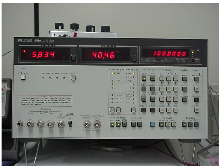
Figura 8.13 – Analisador de impedâncias HP 4192A utilizado na obtenção do módulo e fase da admitância elétrica do atuador.
