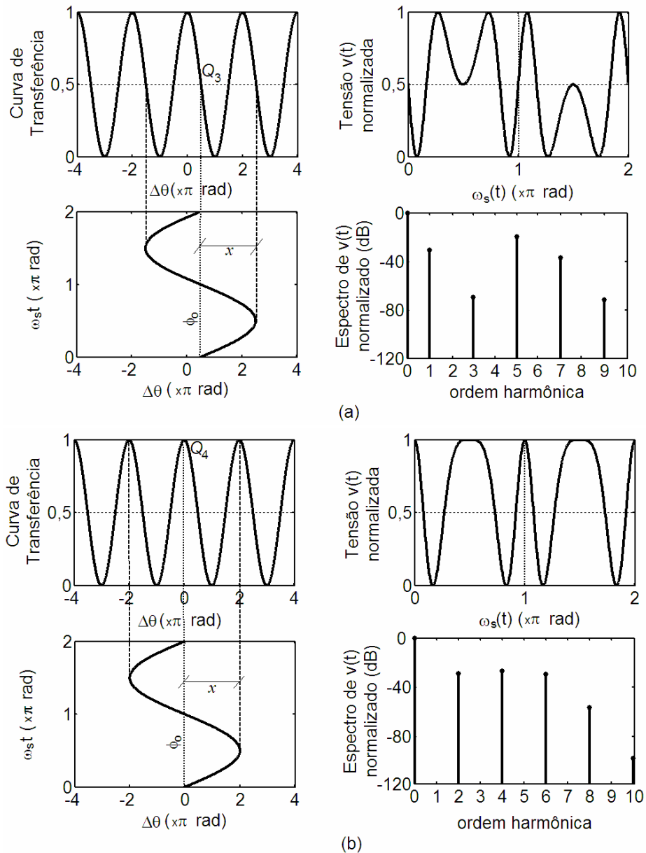
Figura 3.7 – Tensão fotodetectada v(t) e seu espectro de magnitude em dB (até a décima harmônica), normalizados, para uma excitação do tipo \Delta\phi = xsen(\omega_s t) , considerando visibilidade unitária, e regime multi-franjas, com índice de modulação x = 2\pi rad. (a) ponto quiescente Q_3 [ \phi_0(t) = \pi/2 rad]. (b) Ponto quiescente Q_4 [ \phi_0(t) = 0 ].
