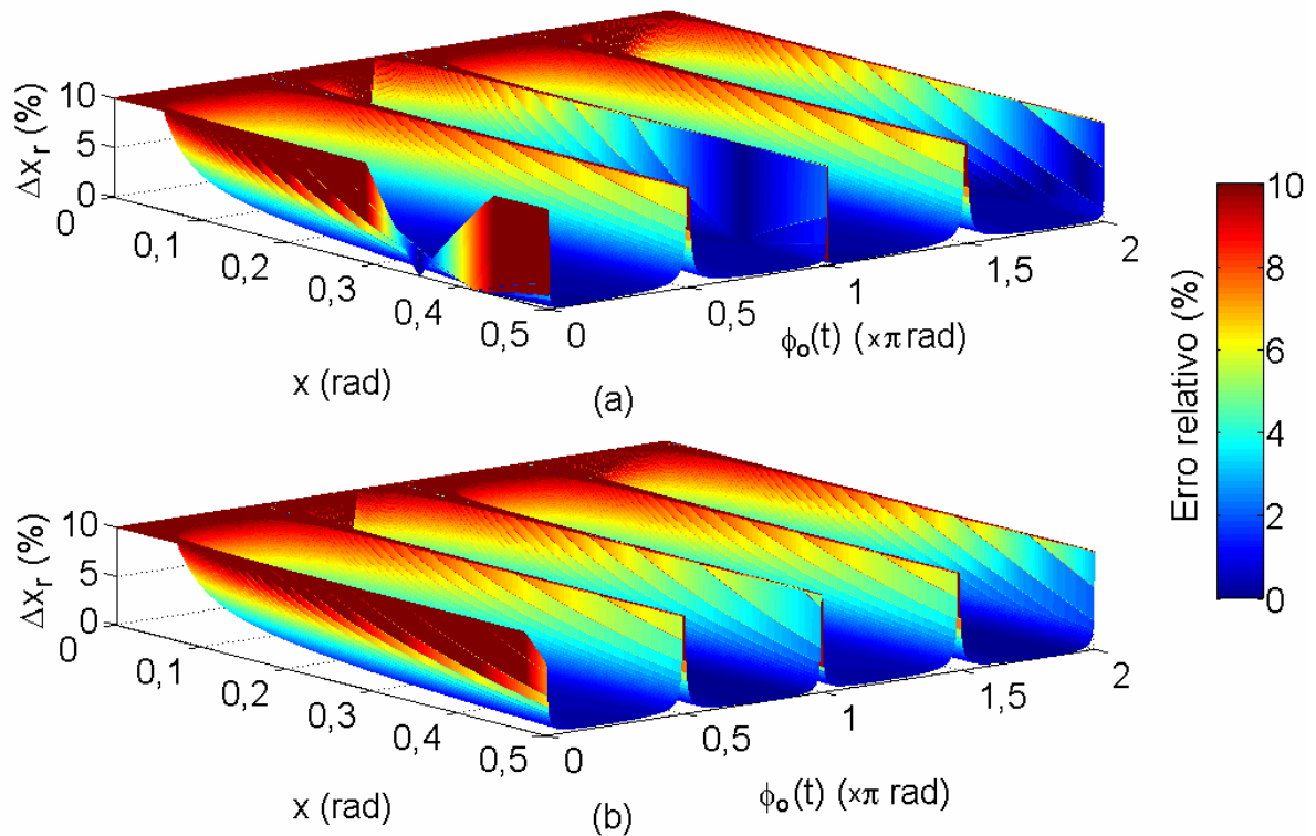
Figura 4.13 – Erro \Delta x_r em função de x e \phi_0(t) , para o método J_0...J_2 . (a) Cálculo para ruído 1/f^2 com K=0,0011 e (b) Cálculo para ruído branco com K=0,0004 .
