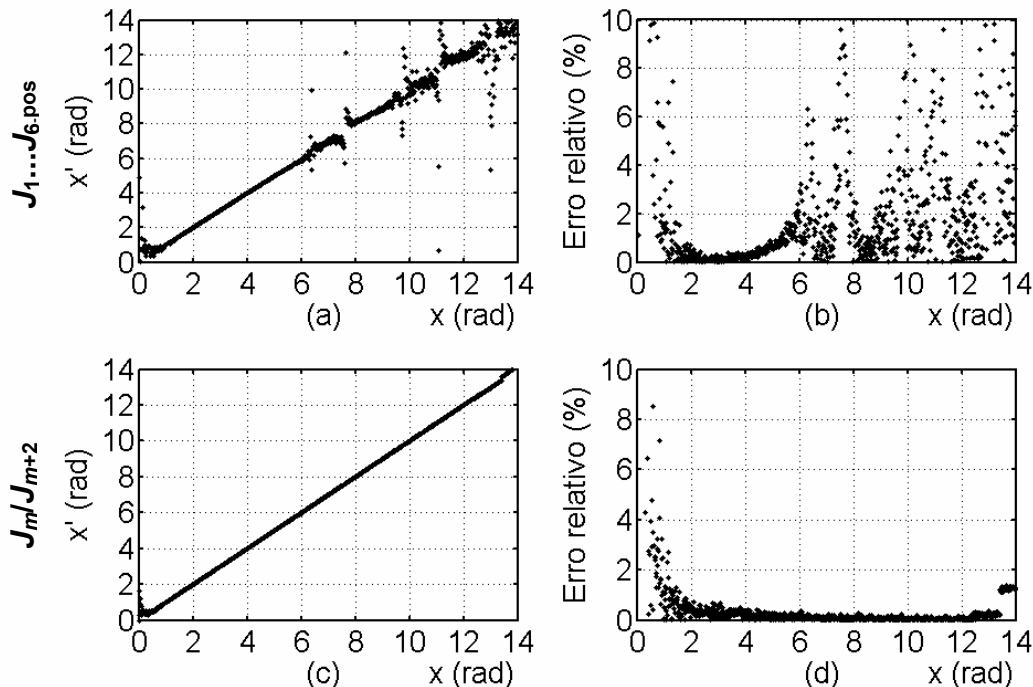
Figura 6.18 – Respostas dos subsistemas de cálculo de x' em função do valor esperado de x , para \phi_o(t)=\pi/4 rad. (a) Método J_1 \dots J_6\text{-pos} . (b) Erro relativo \Delta x_r , pelo método J_1 \dots J_6\text{-pos} . (c) Método J_m/J_{m+2} . (d) Erro relativo \Delta x_r , pelo método J_m/J_{m+2} .
