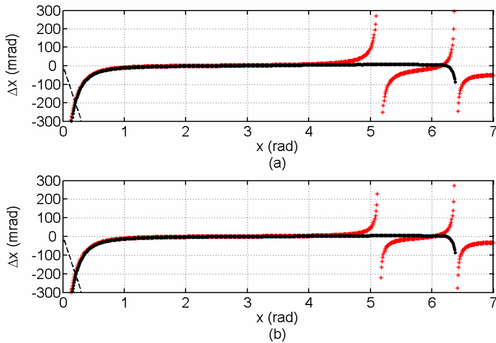
Figura 5.8 – Erro de fase \Delta x em função de x para os métodos (*) J_1...J_4 Modificado e (●) J_1...J_3 , considerando o fator de ruído K . (a) Ruído 1/f^2 com K=0,0011 . (b) Ruído branco com K=0,0004 .
