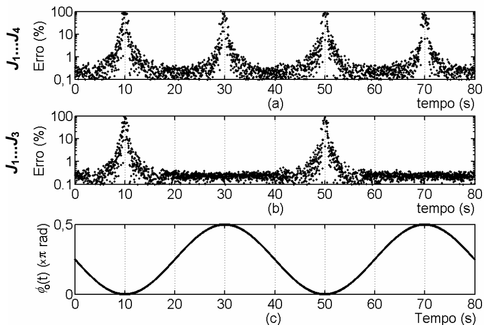
Figura 6.20 – Respostas dos subsistemas de cálculo de x' em função do tempo de simulação, para x=2,6 rad e \phi_0(t) variando. (a) Erro \Delta x_r pelo método J_1...J_4 . (b) Erro \Delta x_r pelo método J_1...J_3 . (c) Fase \phi_0(t) .
