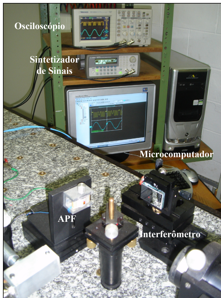
Figura 8.4 – Montagem experimental para caracterização do APF, composto basicamente pelo interferômetro de Michelson, o sintetizador de sinais Agilent 33220A, o osciloscópio digital Tektronix TDS2022 e o microcomputador para aquisição e processamento digital da tensão fotodectada.
