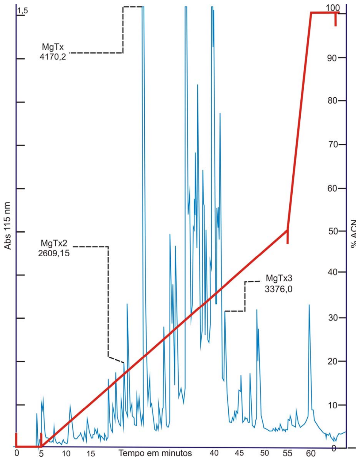
Figura 13: Perfil cromatográfico típico do fracionamento da peçonha de C. margaritatus em coluna de fase reversa C 8 . A peçonha bruta (5 mg) foi dissolvida em 250 µL de TFA 0,1% (v/v) em água Milli-Q e submetida à centrifugação por 15 min a 14.000 rpm. O sobrenadante foi aplicado em uma coluna de fase reversa C 8 (Vydac 208TP54, 4,6 x 250 mm) previamente equilibrada em TFA 0,1% (v/v) em água Milli-Q. As frações foram eluídas com gradiente linear de TFA 0,1% (v/v) em acetonitrila, com fluxo constante de 1,0 mL/min, monitoramento em 215 nm, sendo coletadas manualmente, liofilizadas e armazenadas a -20°C.
