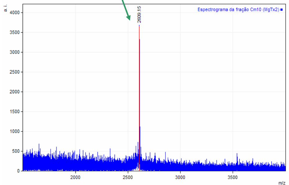
Figura 17. (A) Recromatografia por RP-HPLC da fração Cm10 em coluna C 18 (Vydac 4,6 x 250 mm). (B). Espectrograma de massa (MALDI-TOF) da margatoxina 2 (MgTx2) nativa.
