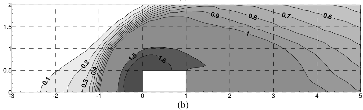
Figura 36 – Distribuição de concentração no chão sob condições atmosféricas estáveis, com a fonte localizada a 10H_b barlavento do prédio. (a) \kappa - \epsilon Padrão e (b) \omega .
