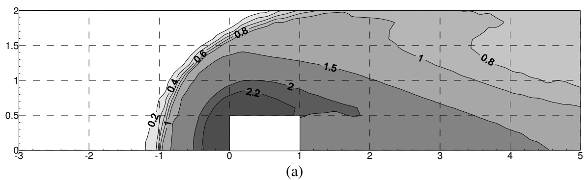
Figura 35 – Distribuição de concentração no plano central sob condições atmosféricas estáveis, com a fonte localizada a 10H_b barlavento do prédio. (a) \kappa - \epsilon Padrão e (b) \omega .
