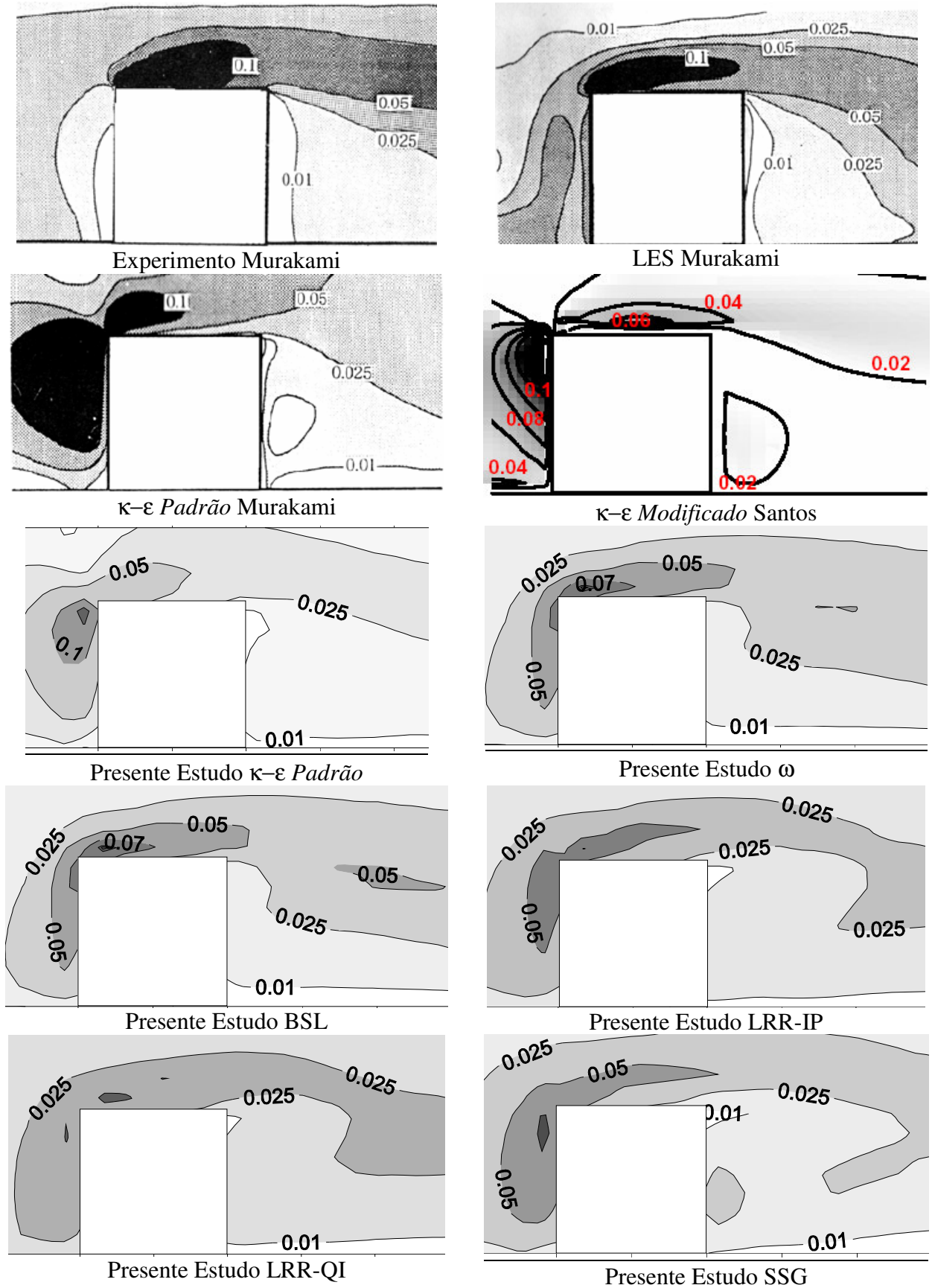
Figura 16 – Distribuição de \overline{u_1 u_1} normalizado por W_{Hb}^2 .
