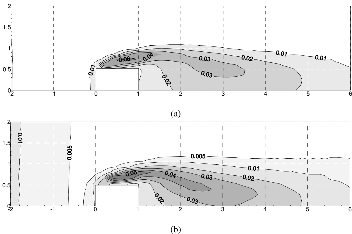
Figura 43 - Distribuição de ECT à metade da altura do prédio sob condições atmosféricas instáveis. (a) \kappa - \epsilon Padrão e (b) \omega .
