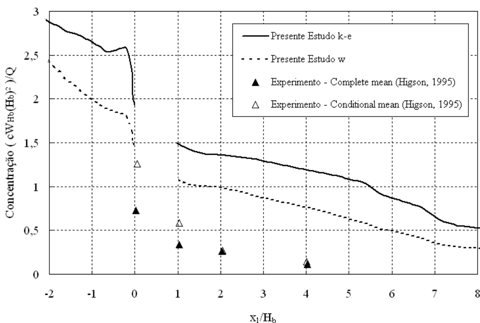
Figura 38 - Perfil de concentração no plano central à metade da altura do prédio sob condições atmosféricas estáveis, com a fonte localizada a 10H_b barlavento do prédio a uma altura de 0,5H_b .
