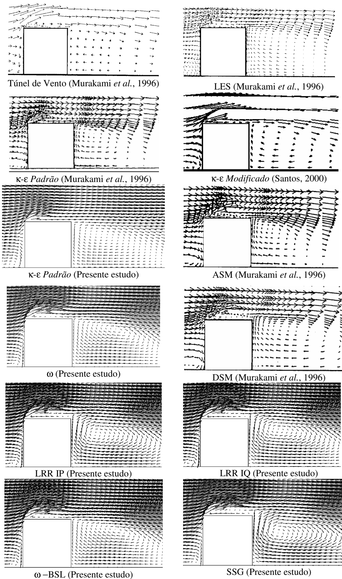
Figura 14 - Campo de Velocidade no plano central do prédio para os diferentes modelos de turbulência.
