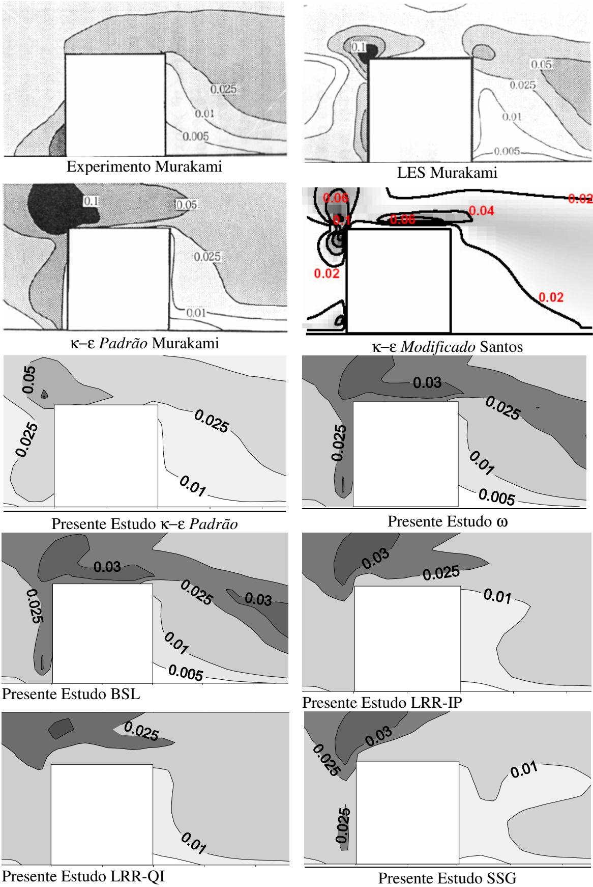
Figura 18 - Distribuição de \overline{u_3 u_3} normalizado por W_{Hb}^2 .
