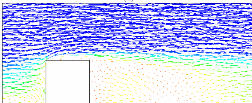
Figura 30 – Vista do plano central do campo de velocidades sob condições atmosféricas estáveis. (a) \kappa - \epsilon Padrão e (b) \omega .
