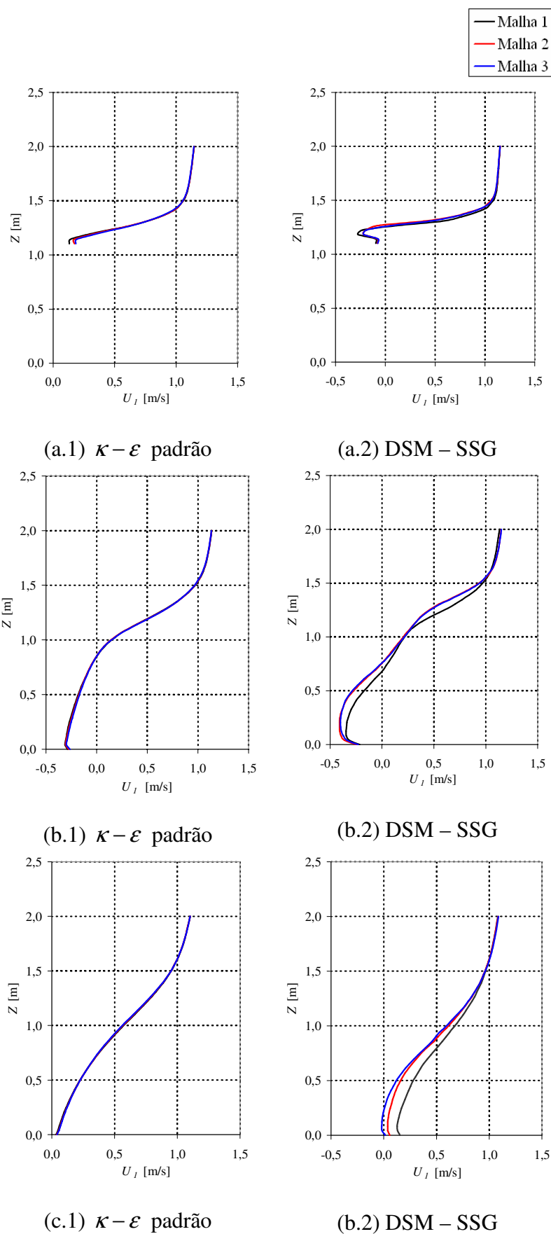
Figura A.4 – Perfil Vertical de Velocidade no plano de simetria para (a.1) e (a.2) centro do prédio, (b.1) e (b.2) 1H_b e (c.1) e (c.2) 3H_b a montante do centro do prédio.
