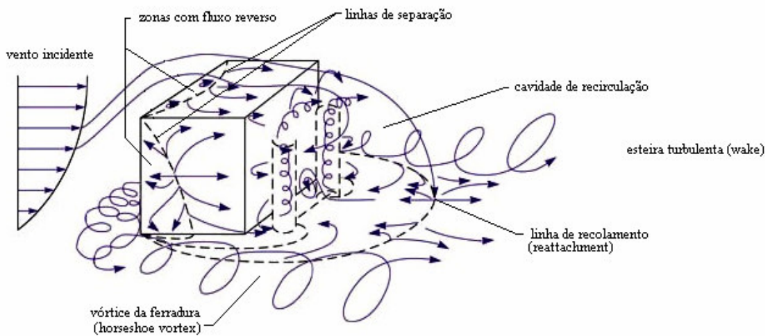
Figura 5 - Estruturas típicas do escoamento ao redor de um obstáculo cúbico – perspectiva tridimensional. Fonte: Hosker (1980).
