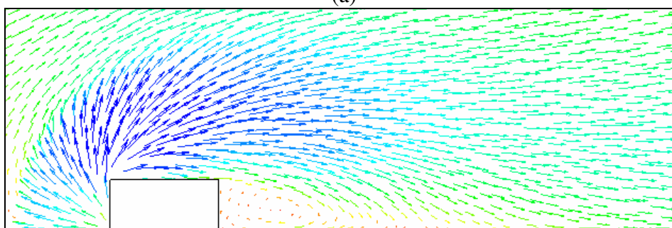
Figura 31 – Vista do plano próximo do chão do campo de velocidades sob condições atmosféricas estáveis. (a) \kappa - \epsilon Padrão e (b) \omega .
