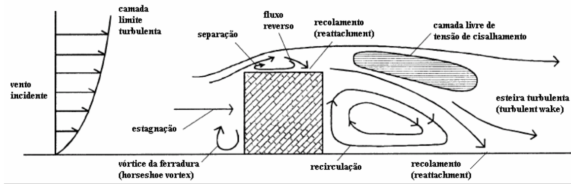
Figura 4 – Representação esquemática do escoamento ao redor de um prédio cúbico – vista do plano central. Fonte: Adaptado de Murakami (1993).
