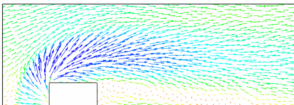
Figura 30 – Vista do plano central do campo de velocidades sob condições atmosféricas estáveis. (a) \kappa - \epsilon Padrão e (b) \omega .
