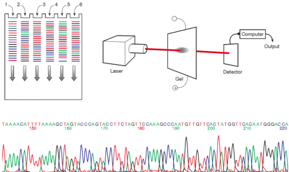
Figura 1. Exemplo do processo de seqüenciamento automatizado com marcadores fluorescentes e detecção a laser. Durante a corrida de um gel de eletroforese com as amostras marcadas, um mecanismo a laser detecta a fluorescência em cada canaleta do gel e gera um fluorograma ou cromatograma. A parte inferior mostra um cromatograma típico, resultado de um seqüenciador ABI PRISM 377. O gel mostrado na figura foi substituído por géis capilares ultrafinos em versões mais modernas de seqüenciadores comerciais. Retirado de (Strachan e Read, 1999).
