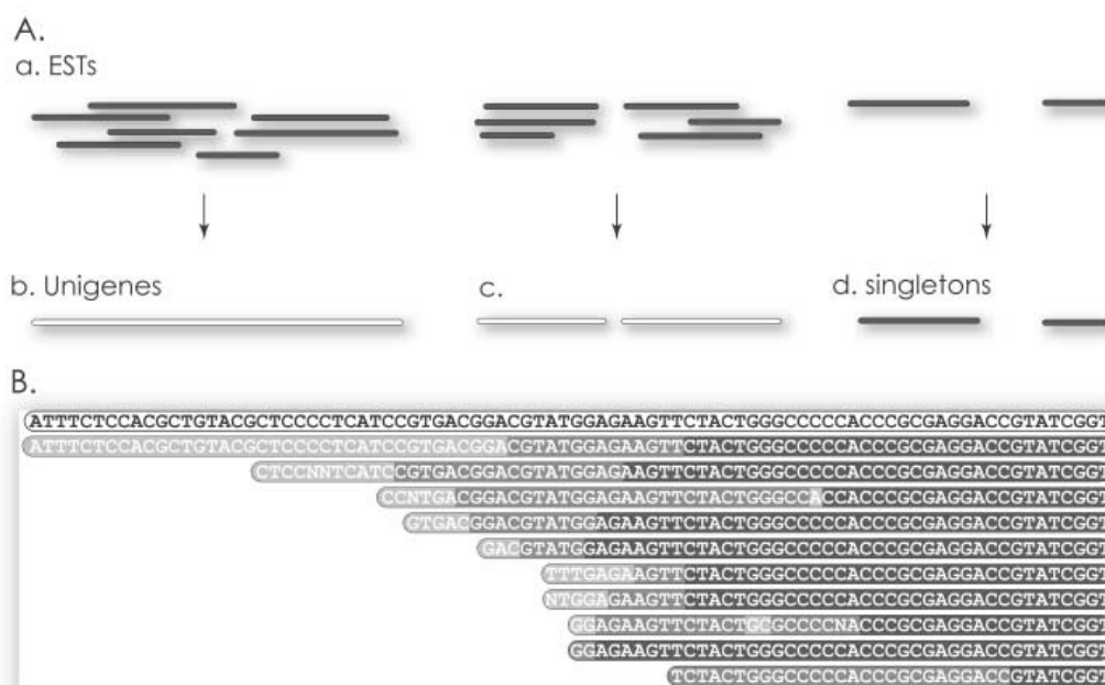
Figura 7. Montagem de Unigenes ou Uniques. A. Formação dos consensos, também chamados Unigenes ou Uniques (b e c) pelas EST (a); seqüências singleton (d) são EST órfãs. B. Exemplo de seqüência consenso (em branco, parte superior), e as seqüências que a representam (tons de cinza). Retirado de (Bouck e Vision, 2007).
