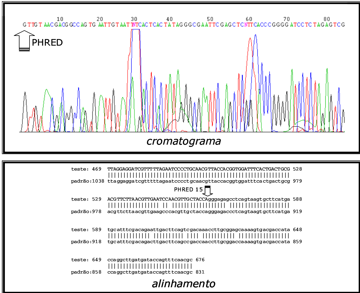
Figura 2: Cromatograma gerado a partir da leitura dos dados brutos do seqüenciador MegaBACE por um programa nomeador de bases (PHRED). Na parte inferior vemos, em letras maiúsculas, as bases que apresentam valor de qualidade acima de 15 e, em letras minúsculas, as que apresentam valor inferior. Tais bases minúsculas, apresentando informação (como visto no alinhamento com o padrão), são frequentemente descartadas em projetos genoma.
