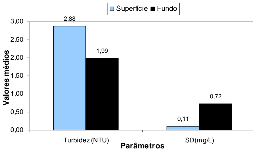
Figura 5.1 . Valores médios dos parâmetros de turbidez e sólidos dissolvidos da superfície e do fundo do reservatório.
