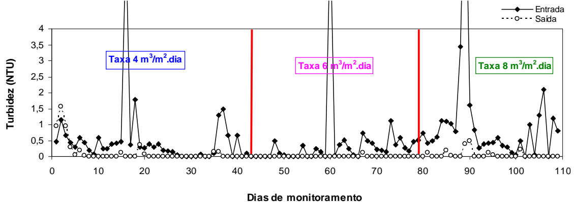
Figura 5.25: Monitoramento da turbidez durante as três taxas de filtração analisadas.
