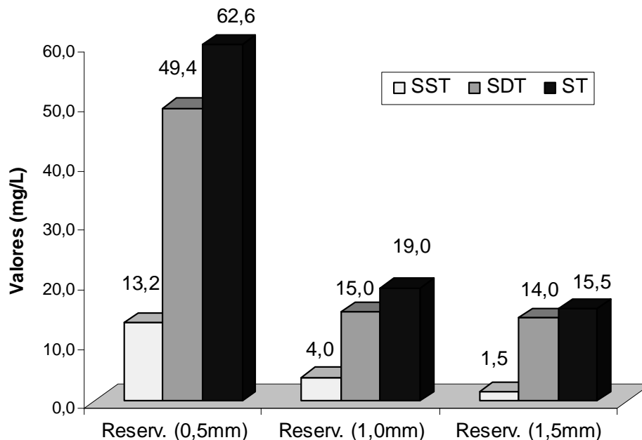
Figura 59 – Concentração de sólidos nas amostras coletadas nas 2ª, 3ª e 4ª etapas
