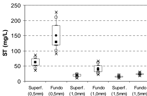
Figura 63 – Comparação dos resultados de ST da chuva da superfície com a chuva do fundo do reservatório
