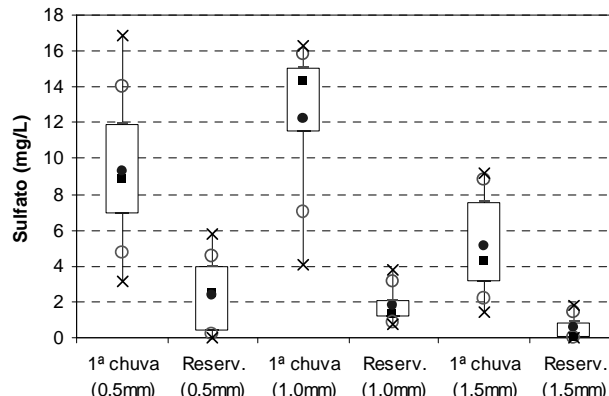
Figura 57 – Concentração de sulfatos nas amostras coletadas nas 2ª, 3ª e 4ª etapas
