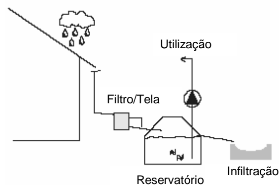
Figura 11 – Sistema com derivação
