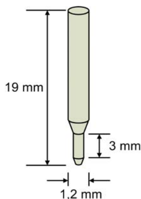
FIGURA 5 - Dimensões do pino Aestheti Plus #2.
