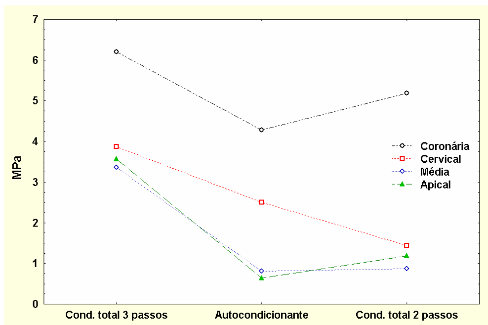
FIGURA 11 - Efeito Região: gráfico de médias dos valores de resistência adesiva (MPa) estabelecidas pelas variáveis região e adesivo.
