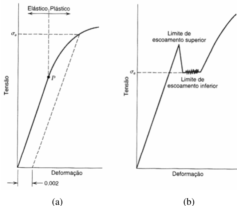
Figura 11 - Comportamento de escoamento (47)
