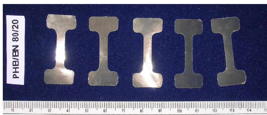
Figura 17 - Corpos de prova para o ensaio de tensão-deformação: PHB/BN 80/20
