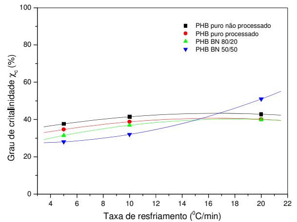
Figura 28 - Grau de cristalinidade \chi_c em função da taxa de resfriamento.
