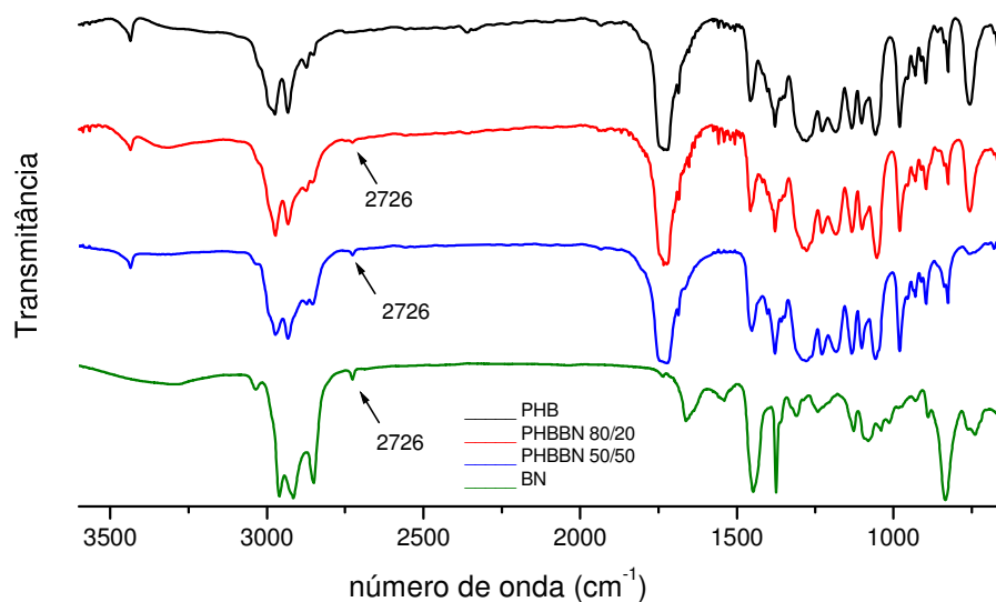
Figura 21 - Espectros de FT-IR para materiais obtidos por casting
