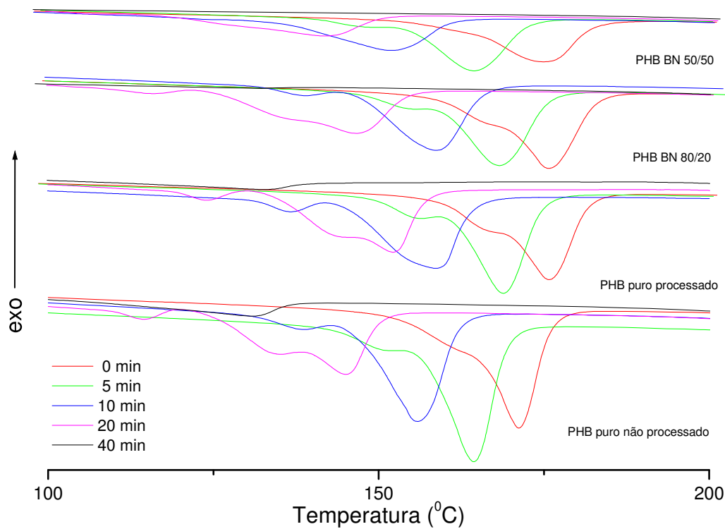
Figura 25 - Influência do tempo de recozimento (isotermas em 190°C)
