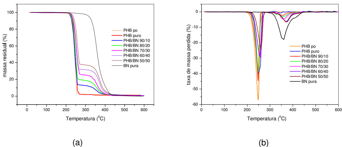
Figura 29 - (a)TGA e (b)DTGA
