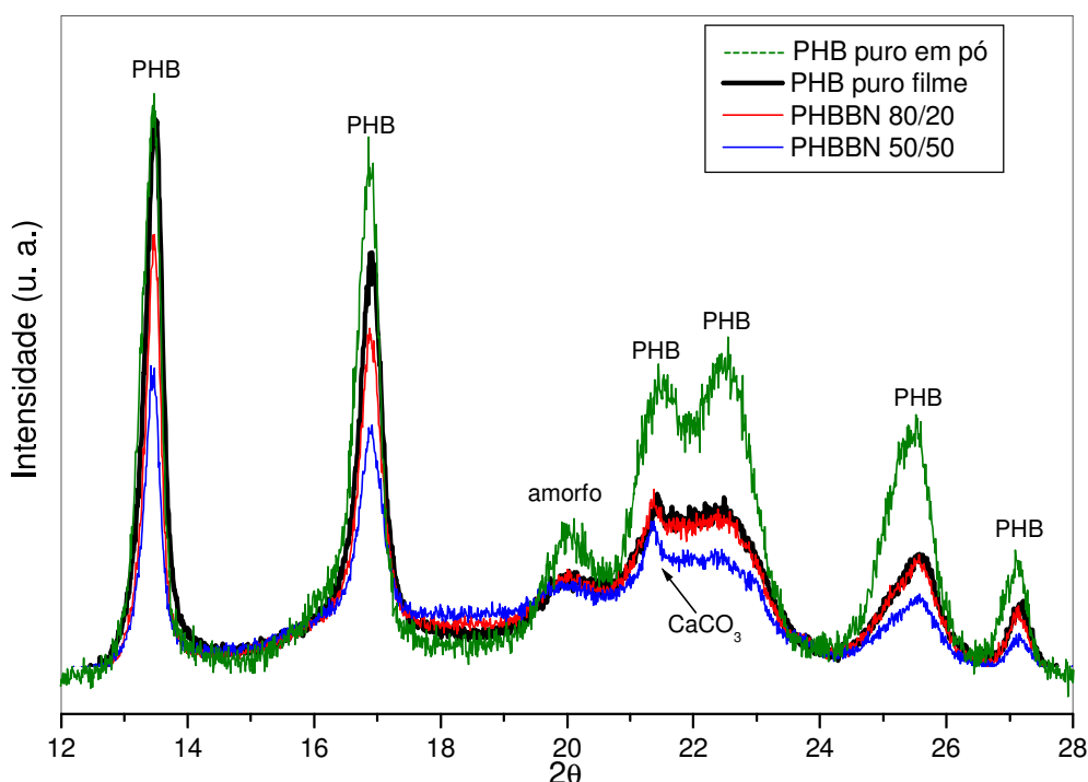
Figura 22 – Difratograma de Raio-X. Filmes de PHB puro, PHBBN 80/20 e PHBBN 50/50, obtidos por prensagem.
