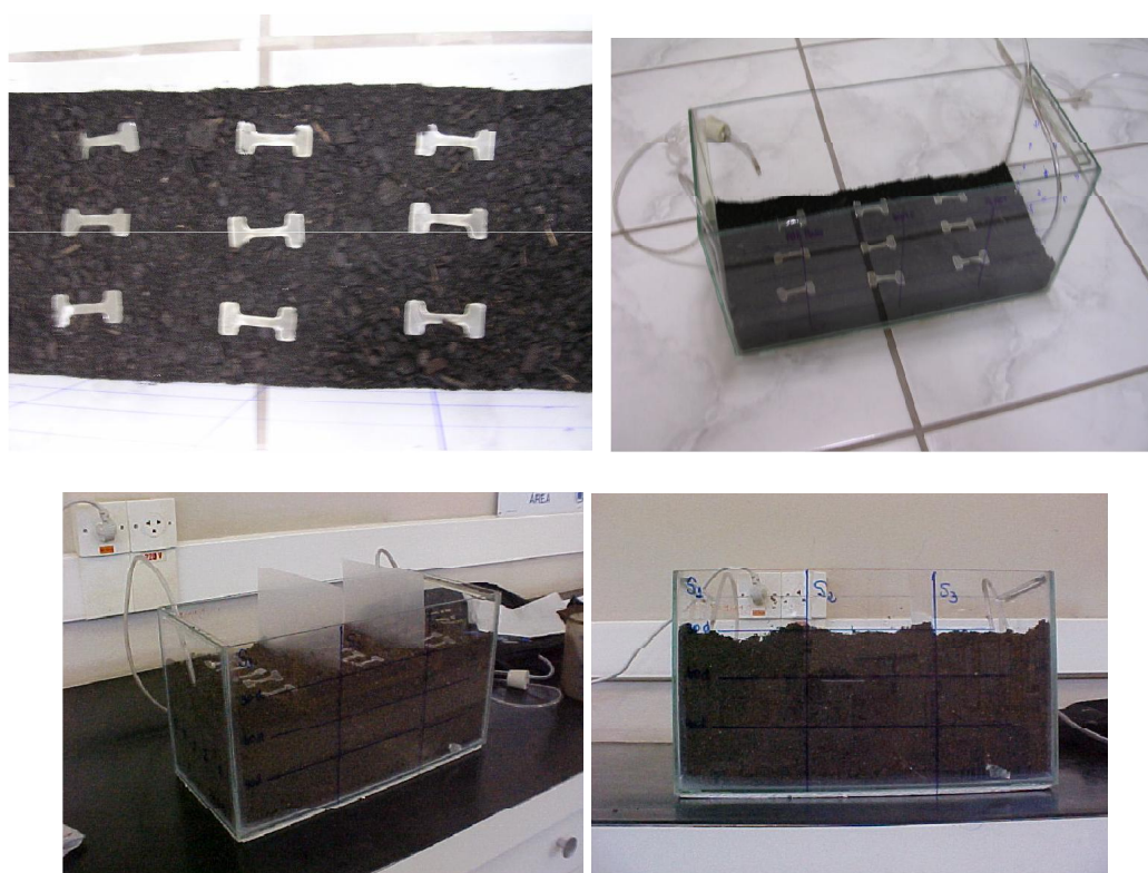
Figura 18 - Sistema empregado no teste de biodegradação (Norma ASTM D-6003 e ASTM G160)
