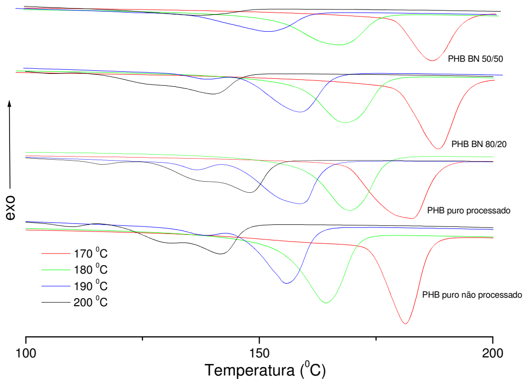
Figura 24 - Influência da temperatura de recozimento (isotermas por 10 minutos)
