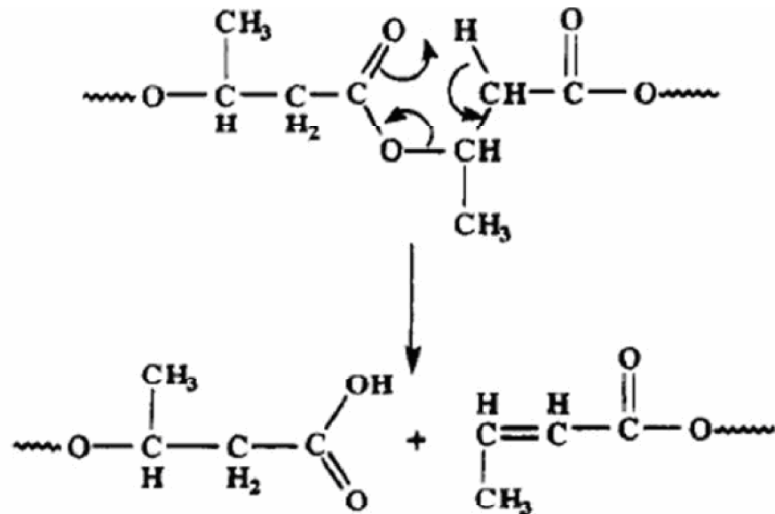
Figura 2 - Processo de degradação térmica do PHB
