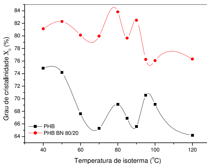
Figura 23 – Graus de cristalinidade do PHB puro e PHBBN 80/20 preparados por prensagem
