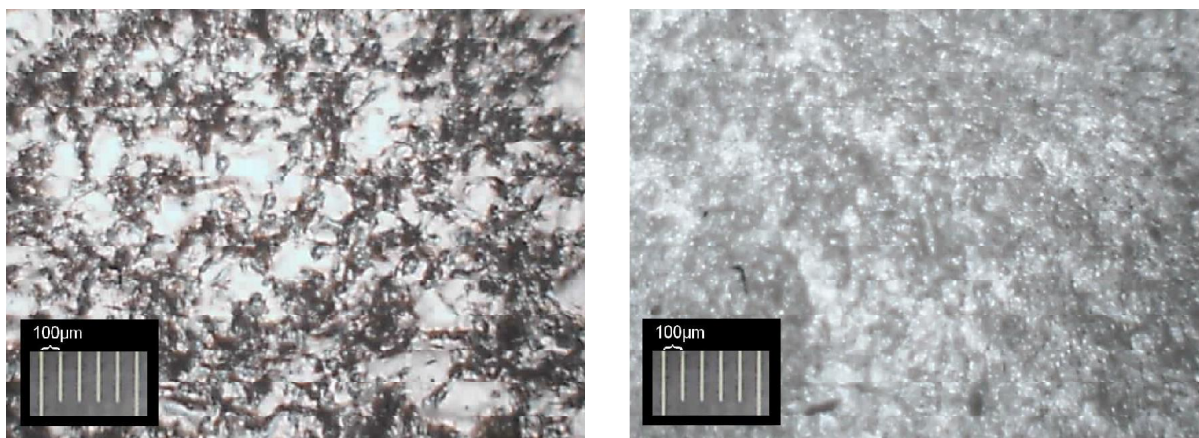
Figura 20 - Micrografias ópticas das blendas PHB/Borracha na proporção 50/50 obtidas por refração. A esquerda preparada por “casting” e a direita por prensagem.
