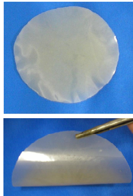
Figura 14 - Filmes de blendas de PHB/BN 80/20 preparadas por prensagem
