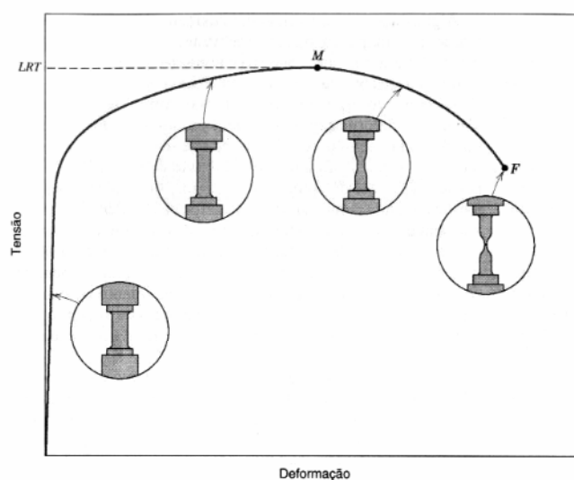
Figura 10 - Tensão-deformação: Comportamento da curva e de formação de pescoço (47)
