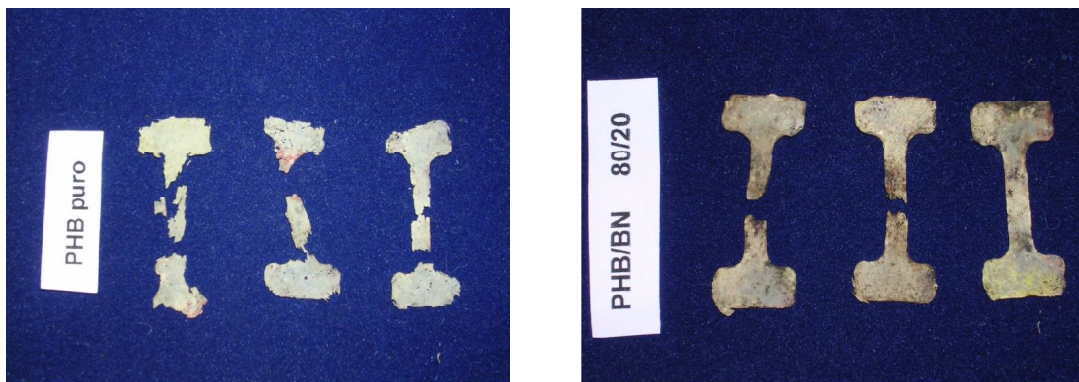
Figura 32 - Corpos de prova após 45 dias. À esquerda o PHB puro e a direita a blenda PHBBN 80/20.
