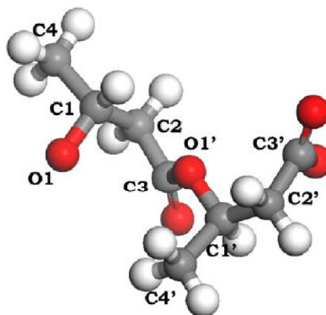
Figura 3 - Estrutura molecular do PHB (23)
