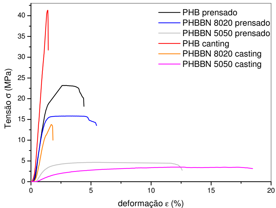
Figura 30 - Gráfico Tensão- deformação
