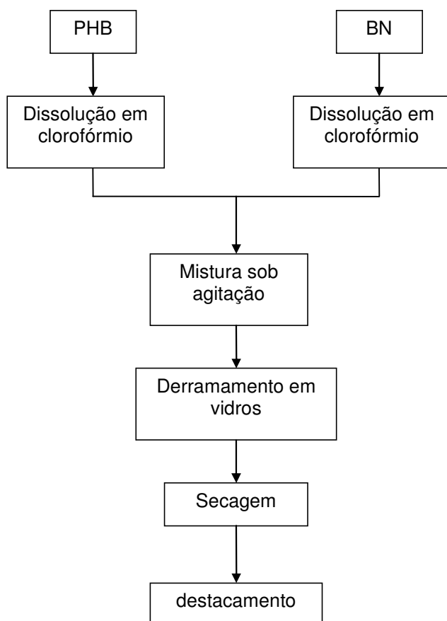
Figura 15 - Diagrama do método de preparação por casting
