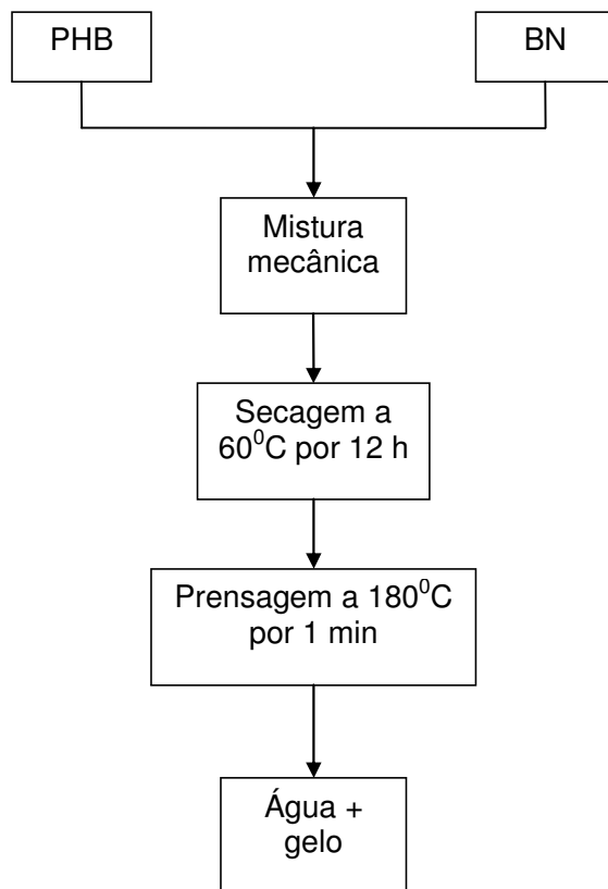
Figura 13 - Diagrama do método de preparação por prensagem
