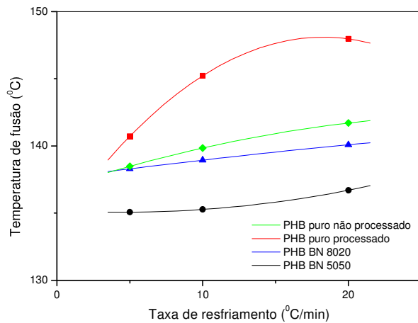
Figura 27 - Temperatura de fusão em função da taxa de resfriamento.
