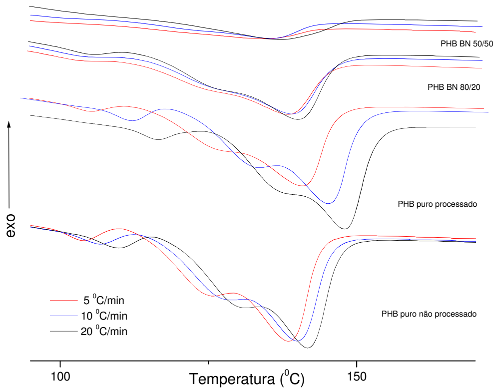
Figura 26 - Influência da taxa de resfriamento (isotermas em 200°C por 10 minutos)
