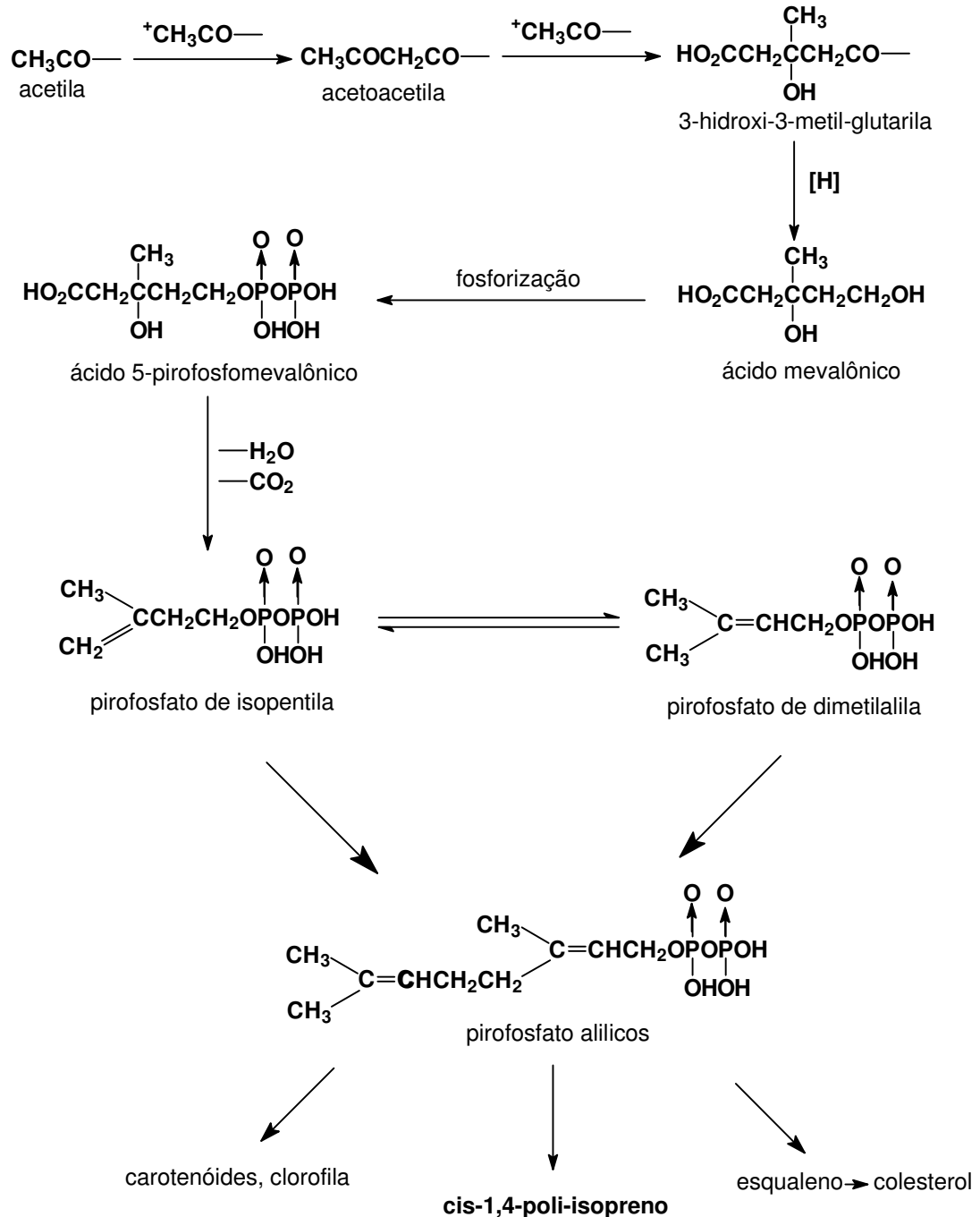
Figura 9 - Principais etapas da biossíntese da borracha natural (41)
