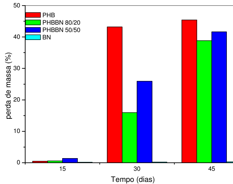
Figura 31 - Ensaio de biodegradação do PHB puro, PHBBN 80/20, PHBBN 50/50 e borracha pura.
