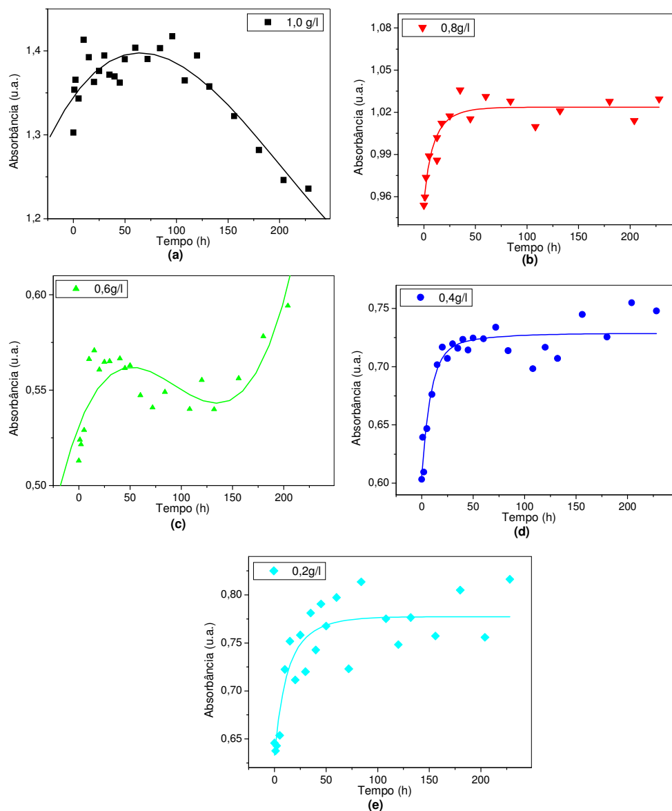
Figura 27: Estudo da cinética de desorção dos filmes formados sob diferentes concentrações de BN com \text{pH}=7,0 . (a) 1,0g/L; (b) 0,8g/L; (c) 0,6g/L; (d) 0,4g/L; (e) 0,2g/L.
