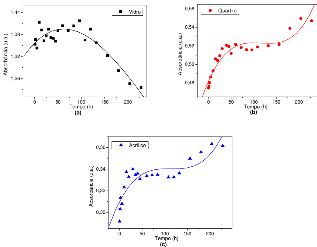
Figura 32: Cinética de dessorção de filmes Pani/BN formados sobre diferentes substratos. Com pH 5,0 e concentração de 0,8g/L para a Pani e pH=7,0 e concentração de 1,0g/L para a BN.
