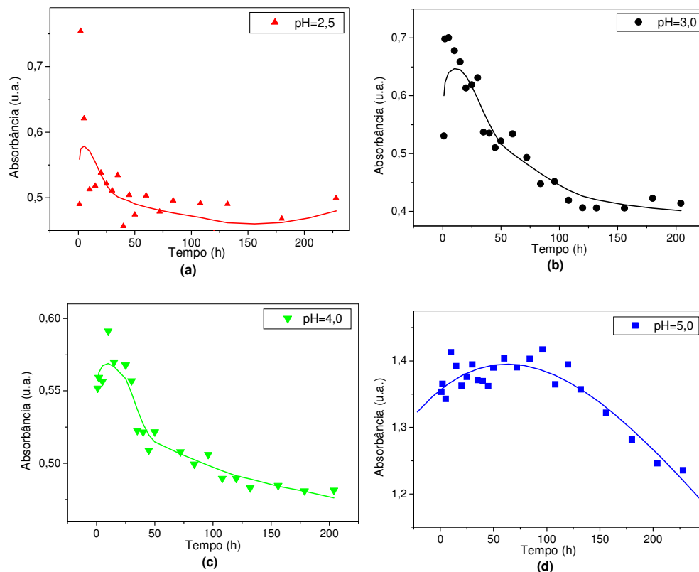
Figura 28: Estudo da cinética de dessorção dos filmes de Pani/BN formados sob diferentes pHs de Pani, com concentrações de 0,8g/L para a Pani e pH=7,0 e concentração de 1,0g/L para a BN.
