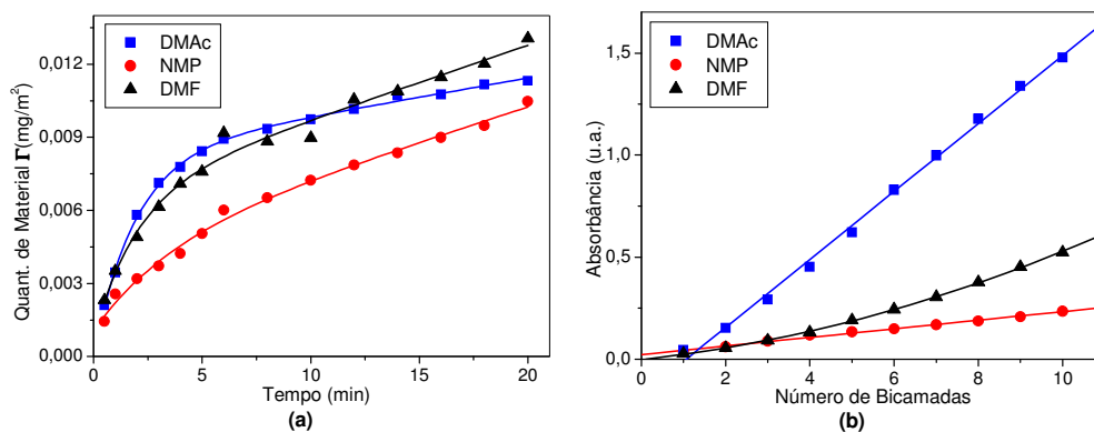
Figura 23: Cinética de adsorção (a) em função do tempo e (b) de formação do filme, para diferentes solventes. Pani com \text{pH}=5,0 e concentração de 0,8\text{g/L} e BN com \text{pH}=7,0 e concentração de 1,0\text{g/L} .
