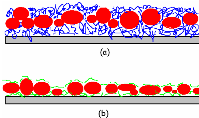
Figura 42: Esquema de adsorção de cadeias de Pani sobre camada de BN (a) Pani desdopada configuração compacta (b) Pani dopada configuração estendida.
