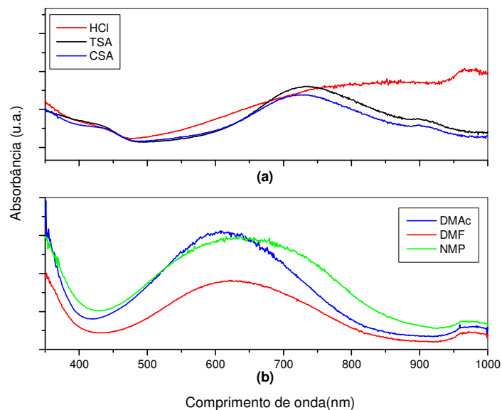
Figura 10: Influência do tipo de dopante e solvente utilizado na solução de polianilina com mesmas concentrações sobre o espectro de absorção no UV-vis (a) três diferentes dopantes em água/DMAc à \text{pH}=2,5 (b) três diferentes solventes sem uso de dopante e com \text{pH}=5,0 .
