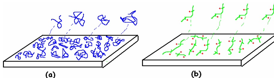
Figura 20: Esquema ilustrativo das cadeias de Pani adsorvendo sobre o substrato em diferentes conformações, de acordo com seu grau de dopagem em (a) enovelada em pHs acima de 3,0 e (b) estendida em pHs abaixo de 3,0.
