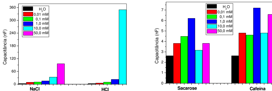
Figura 47: Variação da capacitância em 1kHz para diferentes analitos.
