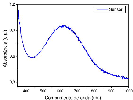
Figura 45: Espectro de absorção no UV-vis do sensor utilizado.
