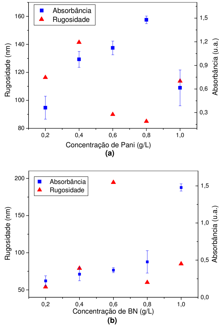
Figura 40: Comportamento da rugosidade e absorbância do filme em função da concentração de (a) Pani e (b) BN. Pani adsorvida a pH=5,0 e BN com pH=7,0.
