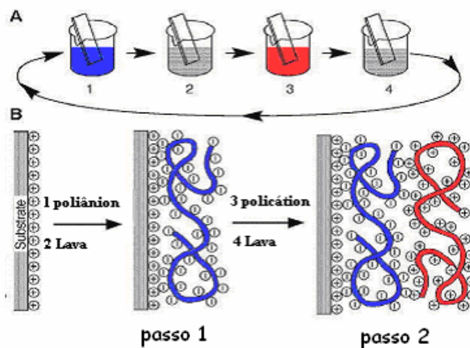
Figura 1: Diagrama esquemático de obtenção de um filme nanoestruturado pelo do método de automontagem 11 .
