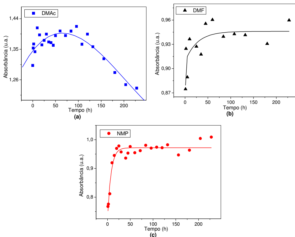
Figura 31: Cinética de dessorção de filmes Pani/BN formados em diferentes solventes. Com pH 5,0 e concentração de 0,8g/L para a Pani e pH=7,0 e concentração de 1,0g/L para a BN.
