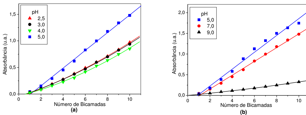
Figura 19: Estudo da cinética de adsorção do filme de Pani/BN: (a) em diferentes pHs de Pani e pH=7,0 da BN e (b) em diferentes pHs de BN e pH=5,0 da Pani. A Pani adsorvendo com concentração de 0,8g/L e a BN de 1,0g/L.
