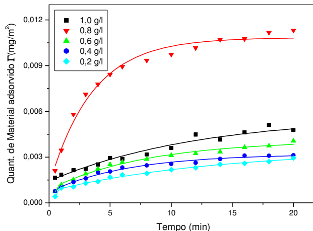
Figura 16: Estudo da cinética de adsorção em função do tempo de imersão da 1ª camada de Pani. Sobre substrato de vidro para diferentes concentrações de Pani com pH=5,0.
