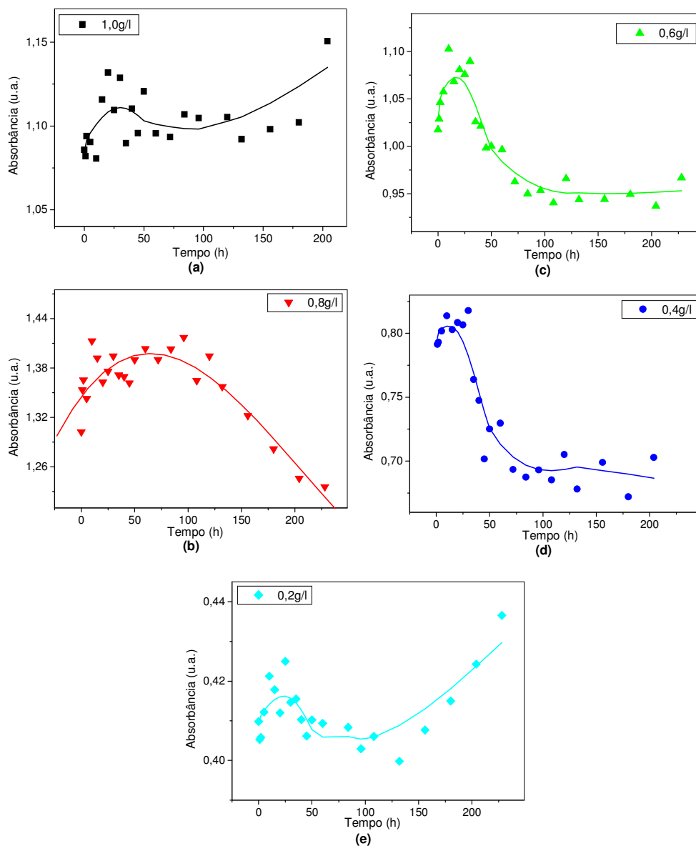
Figura 25: Estudo da cinética de dessorção dos filmes Pani/BN sob diferentes concentrações de Pani com pH=5,0. (a) 1,0g/L; (b) 0,8g/L; (c) 0,6g/L; (d) 0,4g/L; (e) 0,2g/L.
