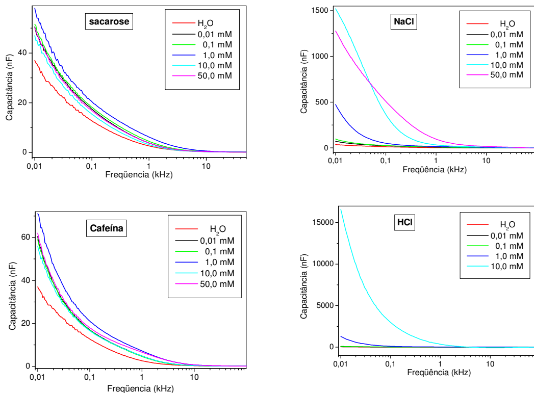
Figura 46: Resultados de espectroscopia de impedância para o sensor em diferentes analitos.
