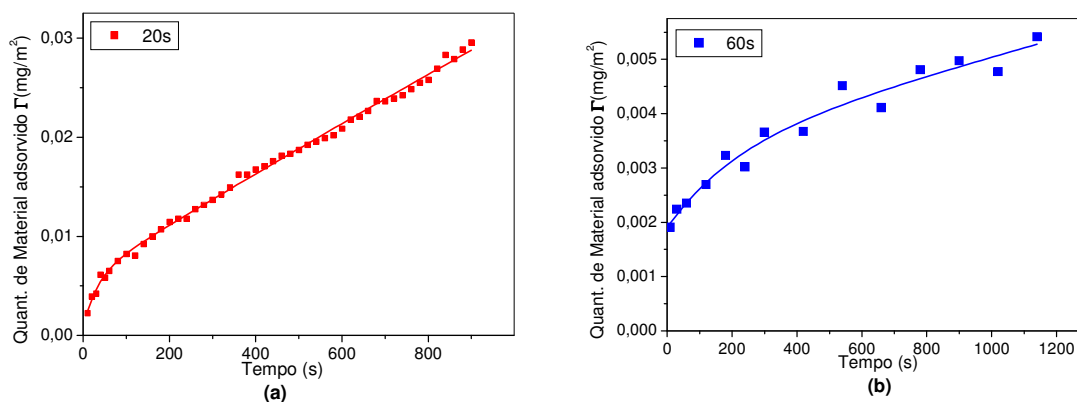
Figura 13: Estudo da cinética de adsorção da 1 a camada de Pani com pH = 5,0 e concentração de 1,0 g/L para dois intervalos distintos de imersão (a) 20s e (b) 60s, sobre substrato de vidro.
