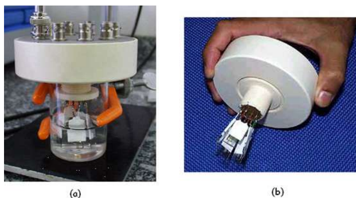
Figura 6: Figura ilustrativa de montagem e utilização da “língua eletrônica” em (a) análise da solução e em (b) arranjo de sensores 49 .
