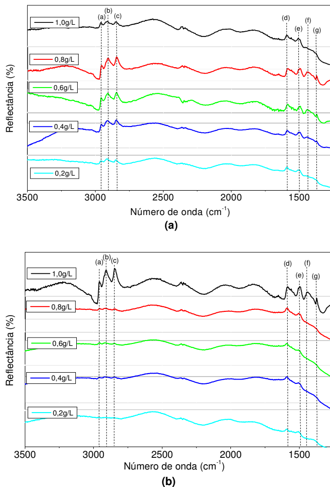
Figura 34: Espectros no infravermelho obtido para filme de Pani/BN obtidos sob diferentes concentrações (a) Pani e (b) BN. Como pH=5,0 para a Pani e pH=7,0 para a BN.
