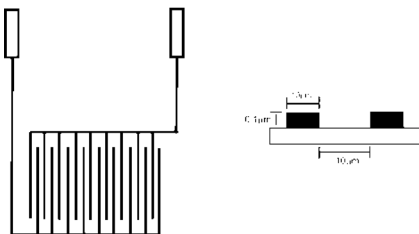
Figura 9: Ilustração do eletrodo utilizado como sensor utilizado e suas dimensões.
