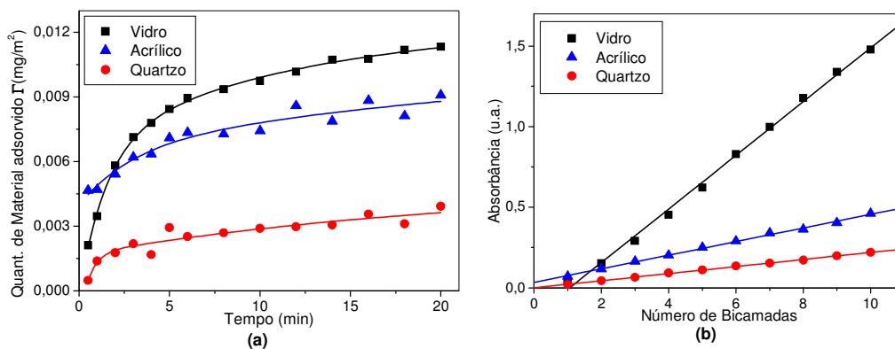
Figura 24: Cinética de adsorção (a) em função do tempo e (b) de formação do filme, para diferentes substratos utilizados. . Soluções com pH 5,0 e 7,0 e concentração de 0,8g/L e 1,0g/L para a Pani e BN, respectivamente.
