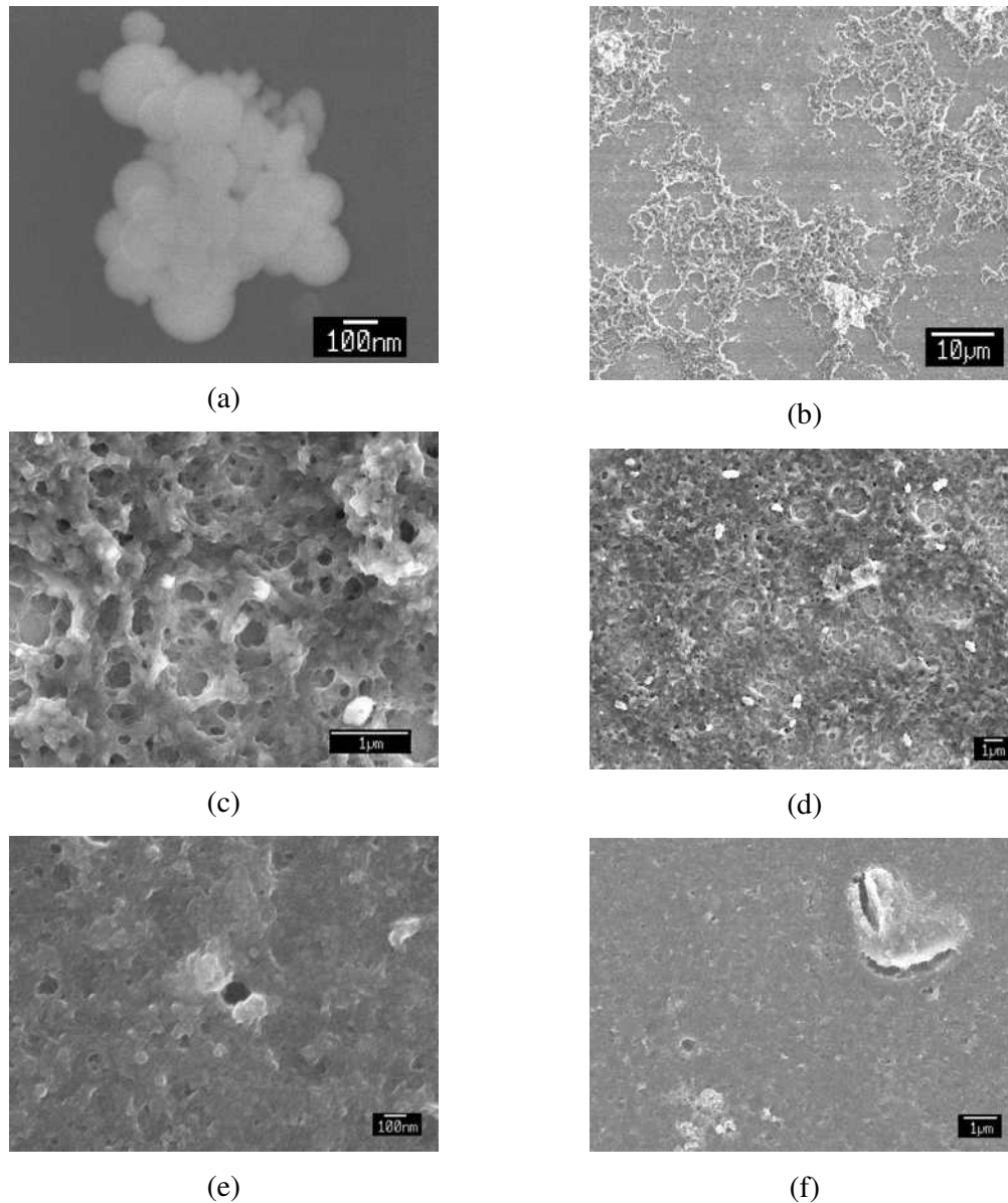
Figura 37: Imagens obtidas pela técnica de FEG para (a) BN depositada por casting em substrato condutor; (b) BN depositada por casting em substrato de vidro; Pani depositada por automontagem em substrato de vidro (c) e (d) desdopada (e) e (f) dopada.
