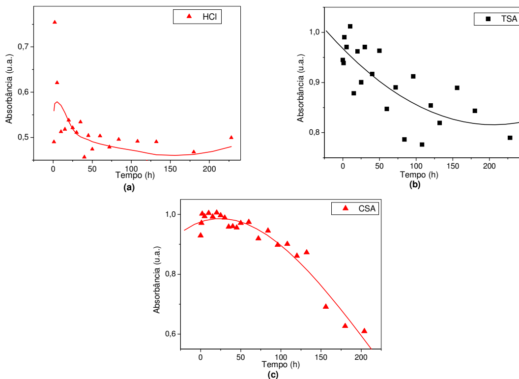
Figura 30: Cinética de dessorção de filmes Pani/BN formados por diferentes dopantes. Com pH 2,5 e concentração de 0,8g/L para a Pani e pH=7,0 e concentração de 1,0g/L para a BN.
