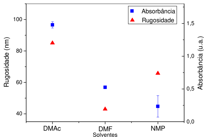
Figura 44: Comportamento da rugosidade e absorbância do filme em função do solvente. Pani adsorvida com pH=5,0 e concentração de 0,8g/L e BN com pH=7,0 e concentração de 1,0g/L.
