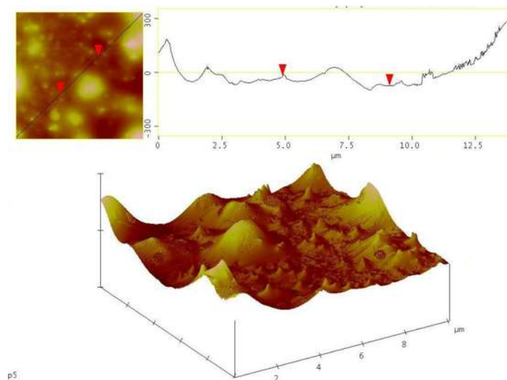
Figura 39: Imagem obtida por AFM do filme de Pani/BN. Pani com pH=5,0 e concentração de 0,8g/L e BN com pH=7,0 e concentração de 1,0g/L.
