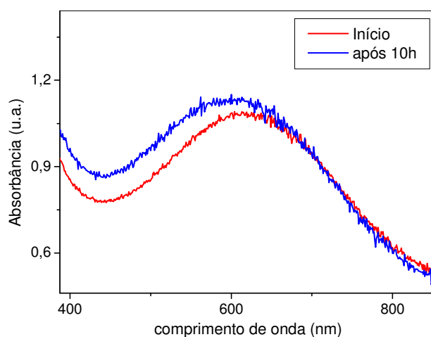
Figura 26: Espectro de absorção do filme de Pani/BN, formado com a Pani em pH=5,0 e concentração de 1,0g/L e a BN em pH=7,0 e concentração de 1,0g/L, antes e depois do processo de lavagem.
