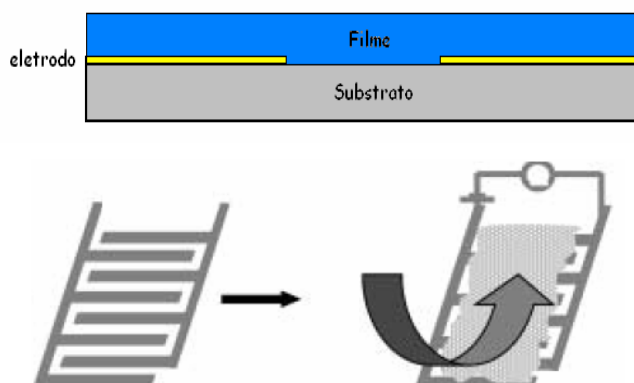
Figura 5: Esquema de um eletrodo utilizado como sensor com camada de filme polimérico depositada.
