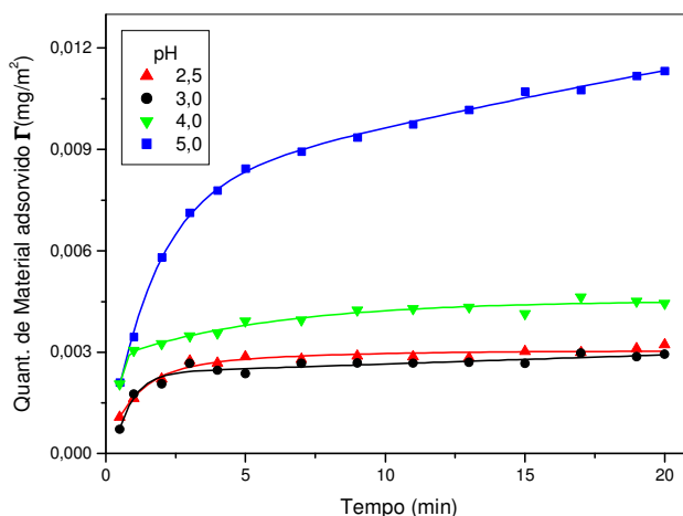
Figura 18: Estudo da cinética de adsorção da primeira camada de Pani em função do tempo de imersão para diferentes pHs. Pani em concentração de 0,8g/L.
