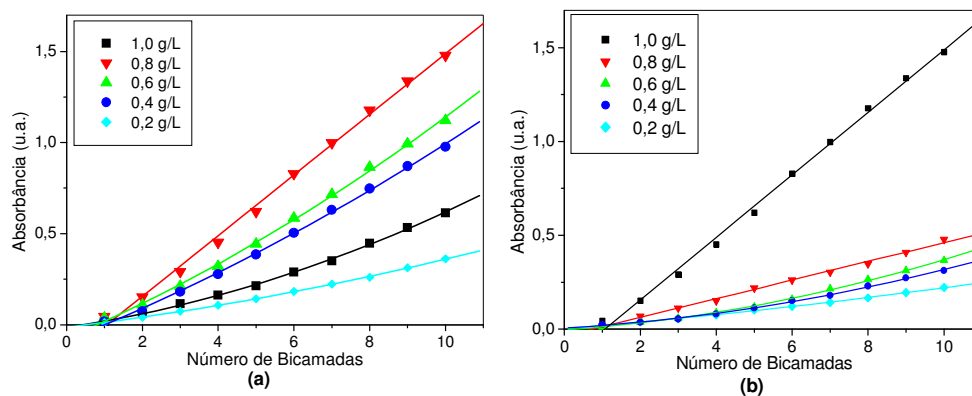
Figura 17: Estudo da cinética de adsorção do filme de Pani/ BN formado a diferentes concentrações: (a) de Pani (b) de BN. Sendo a Pani adsorvida em pH=5,0 e a BN em pH=7,0.
