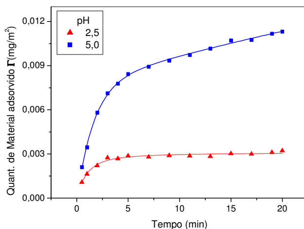
Figura 14: Estudo da cinética de adsorção em função do tempo de imersão da 1ª camada de Pani com concentração de 0,8g/L para dois pHs distintos, sobre substratos de vidro.
