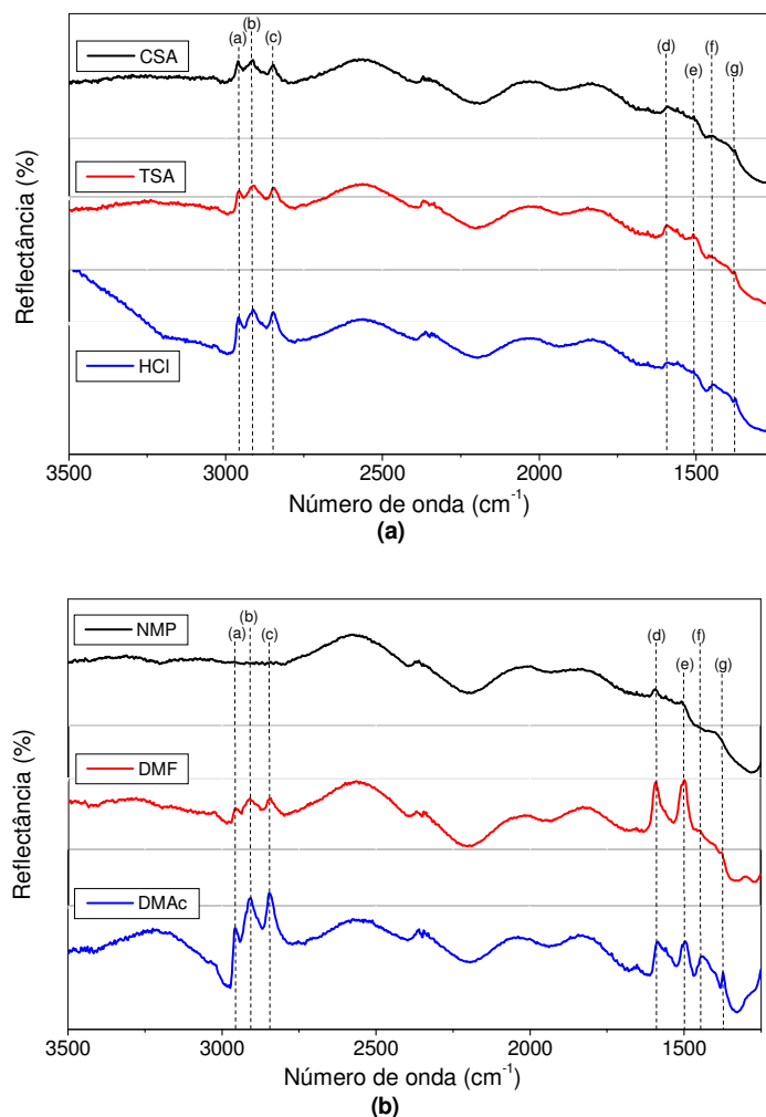
Figura 36: Espectros no infravermelho obtido para filme de Pani/BN obtidos sob diferentes (a) dopantes e (b) solventes, com concentrações de 0,8 e 1,0g/l e pH 5,0 e 7,0, respectivamente.
