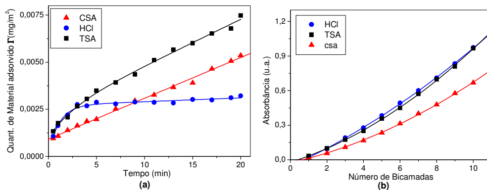
Figura 21: Cinética de adsorção (a) em função do tempo e (b) de formação do filme, para diferentes dopantes utilizados. Pani adsorvida com pH=2,5 e concentração de 0,8g/L e a BN com pH=7,0 e concentração de 1,0g/L.
