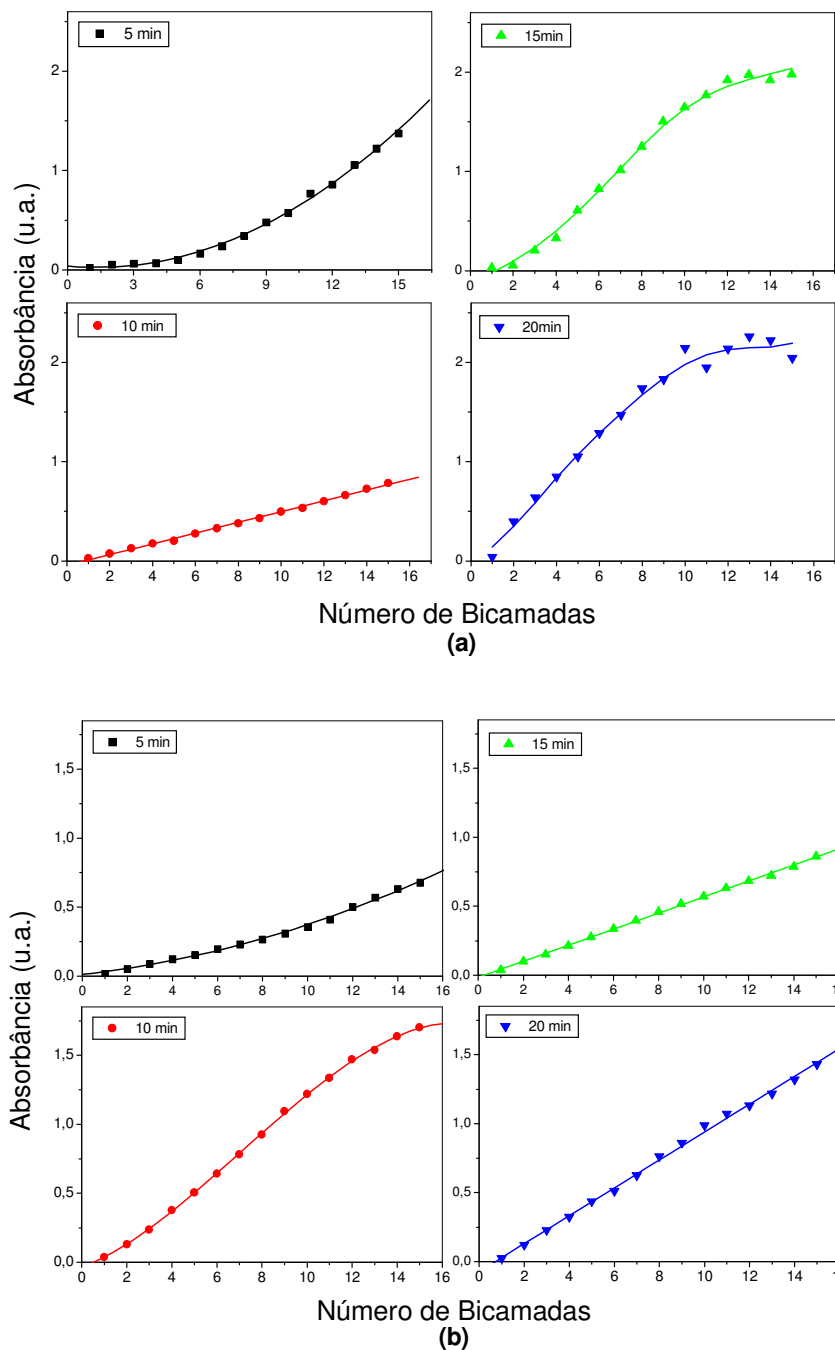
Figura 15: Cinética de adsorção de um filme de Pani/BN com um total de 15 bicamadas formado em diferentes tempos de deposição. A Pani com (a) pH=2,5 e (b) pH=5,0, com concentração de 1,0g/L e a BN com pH=7,0 e concentração de 1,0g/L.
