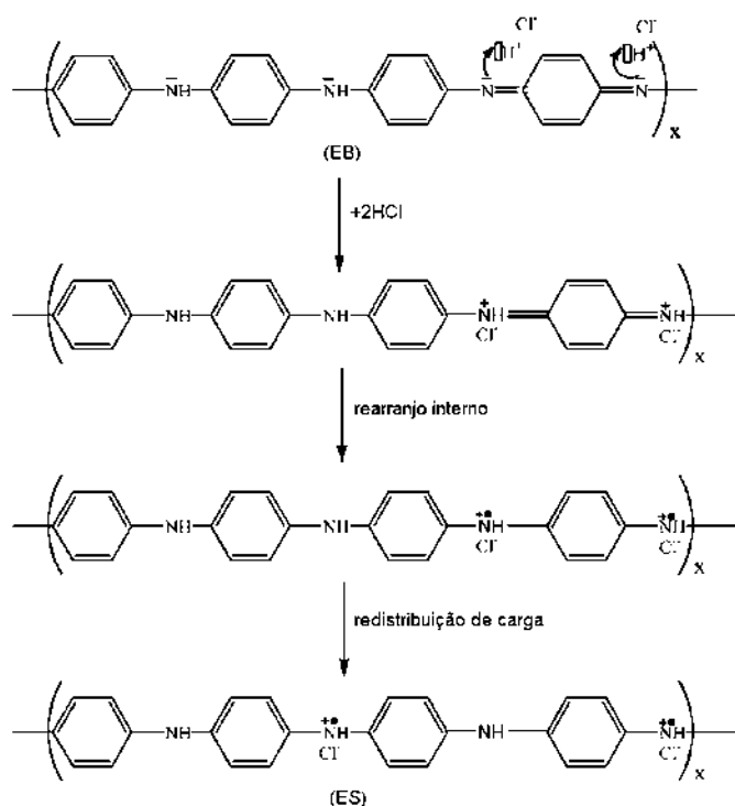
Figura 3: Esquema do processo de dopagem da polianilina por protonação 38 .
