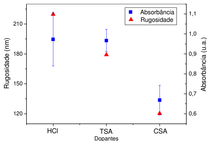
Figura 43: Comportamento da rugosidade e absorvância do filme em função do dopante. Pani adsorvida com pH=2,5 e concentração de 0,8g/L e BN com pH=7,0 e concentração de 1,0g/L.
