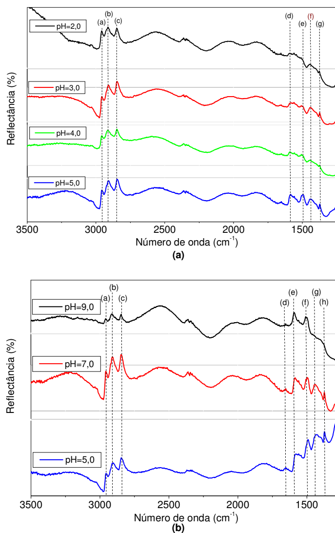
Figura 35: Espectros no infravermelho obtido para filme de Pani/BN obtidos sob diferentes pHs e concentrações 0,8 e 1,0g/L, respectivamente.
