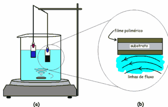
Figura 7: Ilustração do sistema para estudo da cinética de dessorção: (a) lavagem e (b) cisalhamento na interface filme/fluido causado pelo vórtice.
