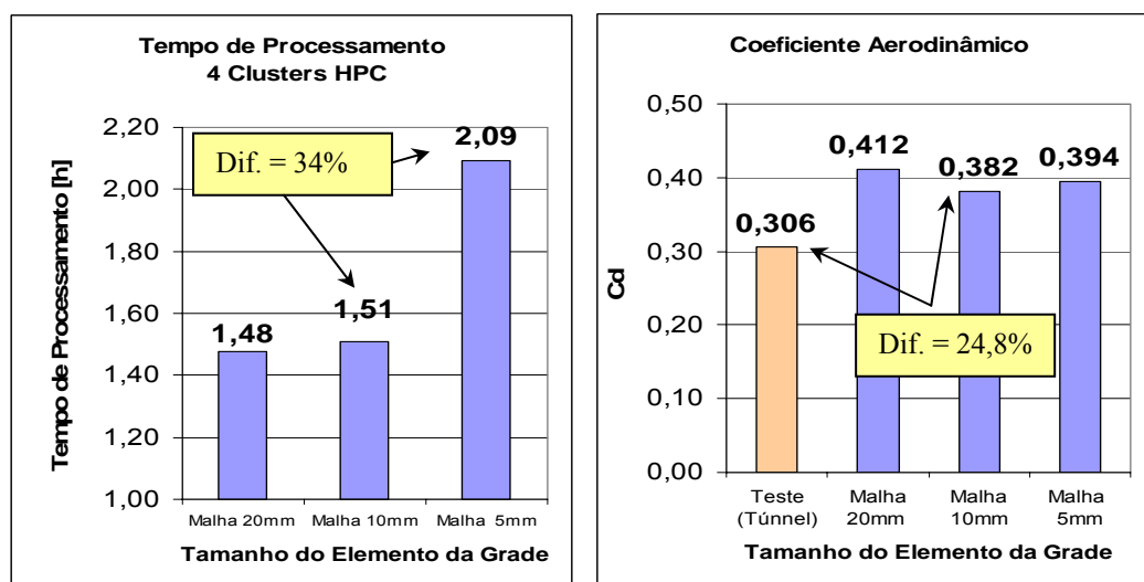
Figura 5.18 - Estudo da Influência de malha da grade no fluxo de ar no radiador. a) Tempo de processamento. b) Coeficiente aerodinâmico.
