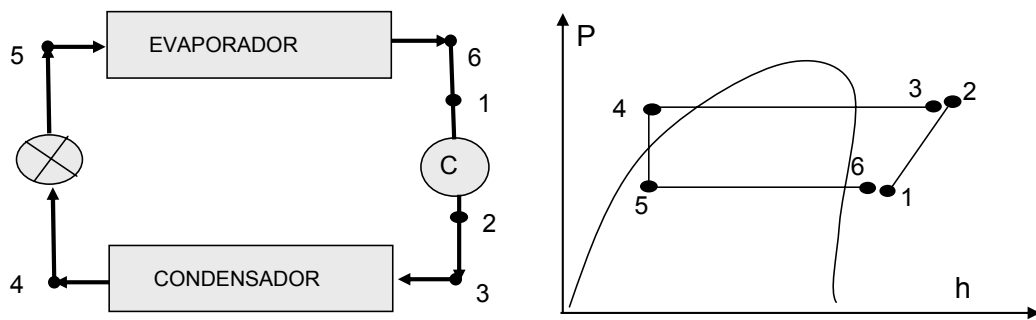
Figura 6.4 - Pontos instrumentados do circuito de refrigeração do veículo A.
