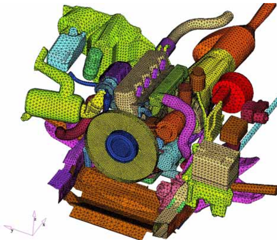
Figura 6.13 - Malha superficial dos componentes do motor.
