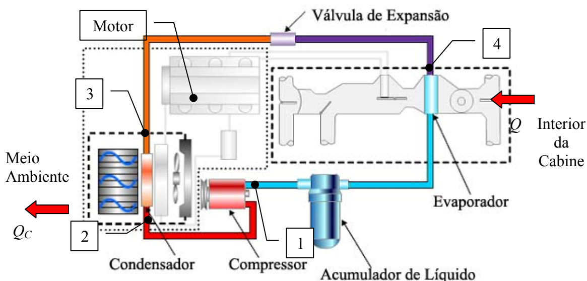
Figura 1.12 - Sistema de arrefecimento da cabine.
