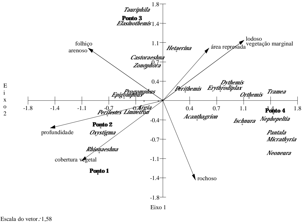
Figura 17. Diagrama de ordenação da Análise de Correspondência Canônica (CCA) da distribuição dos gêneros de Odonata, nos pontos de coleta, em função dos fatores ambientais com os vetores dos mesmos.
