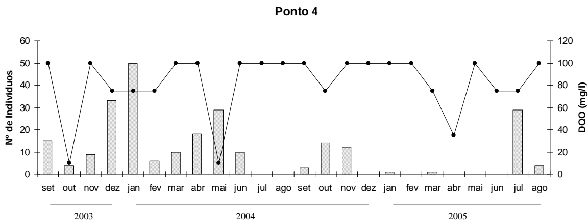
Figura 16. Variação de DQO e número de indivíduos da família Libellulidae no Ponto 4 durante o período de agosto de 2003 a setembro de 2005.
