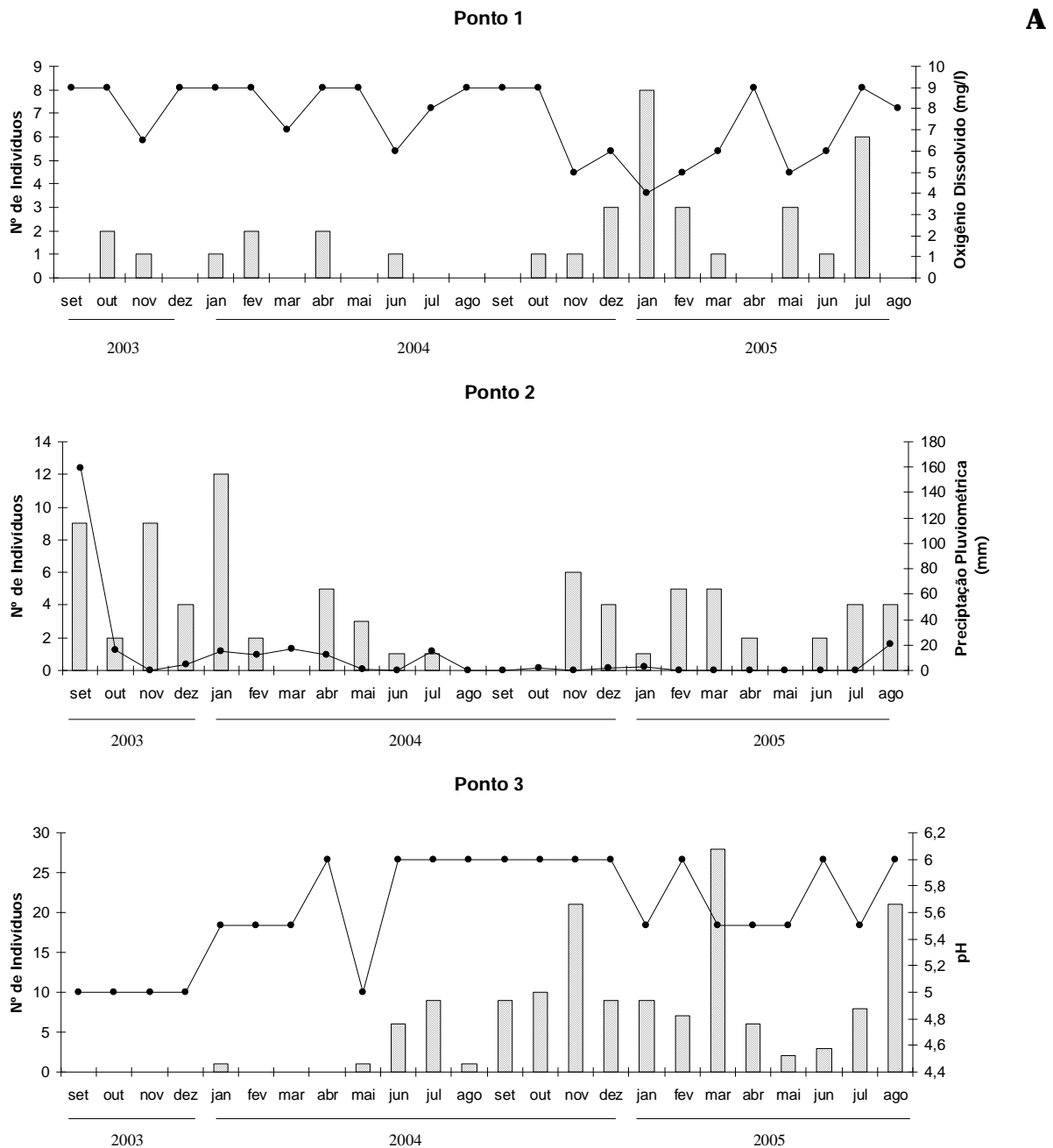
Figura 15: A-C. Variação de fatores abióticos e número de indivíduos da família Megapodagrionidae durante o período de agosto de 2003 a setembro de 2005. (A) Oxigênio Dissolvido – Ponto 1; (B) Precipitação Pluviométrica; (C) pH – Ponto 3.
