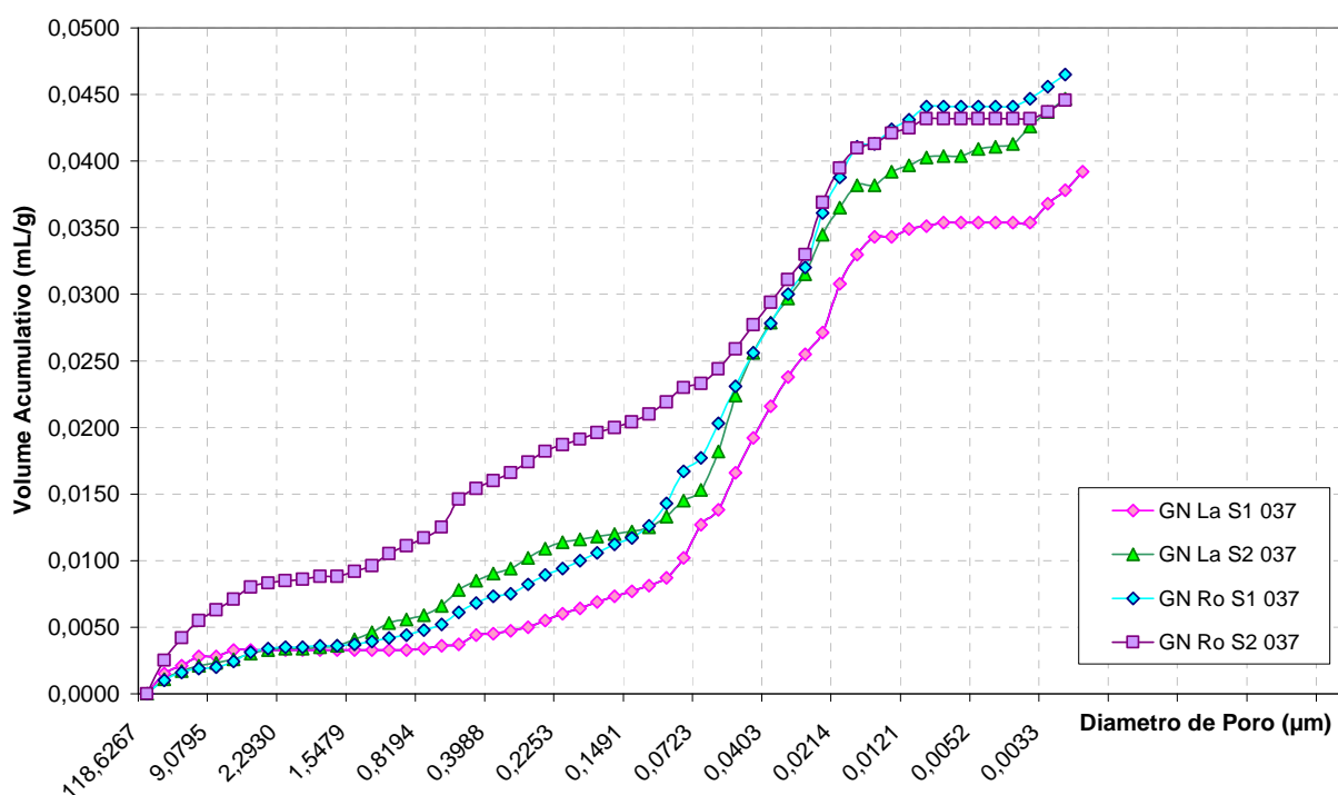
Figura 128: gráfico “diâmetro de poro x volume acumulativo” - comparativo.
