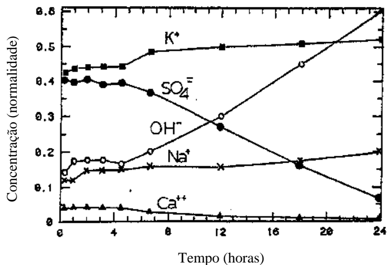
Figura 10: composição da solução dos poros x tempo (DIAMOND, 1983).
