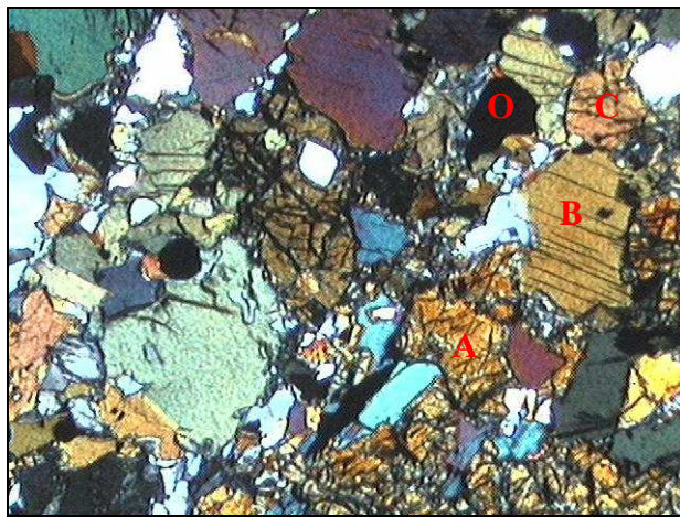
Figura 34: porção da matriz onde predomina anfibólio (A), clinopiroxênio (C), biotita (B) e minerais opacos (O). Aumento de 40x / luz polarizada.
