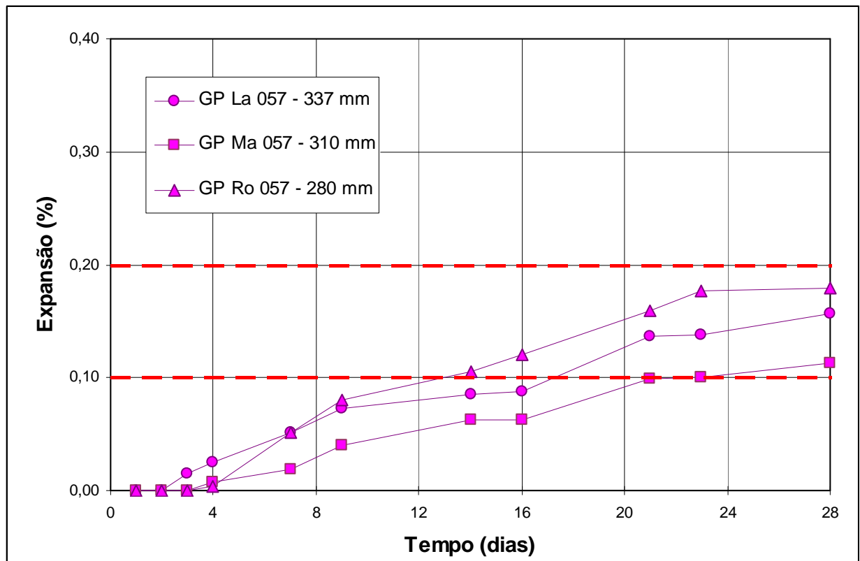
Figura 66: expansões até 28 dias da rocha GP, relação a/c 0,57, três moagens (S1).
