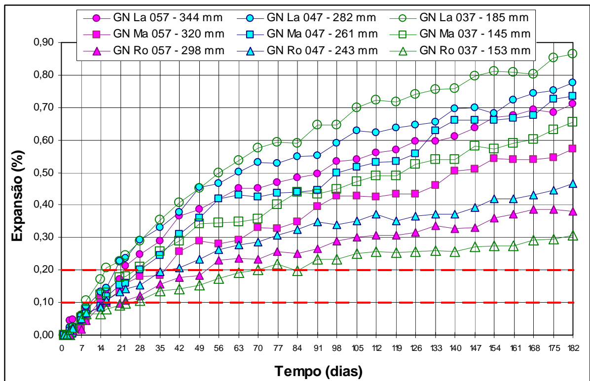
Figura 63: expansões até 182 dias, da rocha GN, três relações a/c e três moagens (S1).
