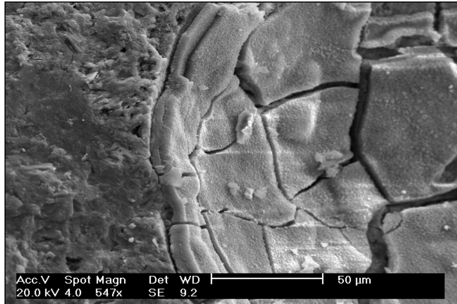
Figura 24: imagem de gel maciço gretado da reação álcali-agregado obtida por Microscopia Eletrônica de Varredura. (VALDUGA, 2002).
