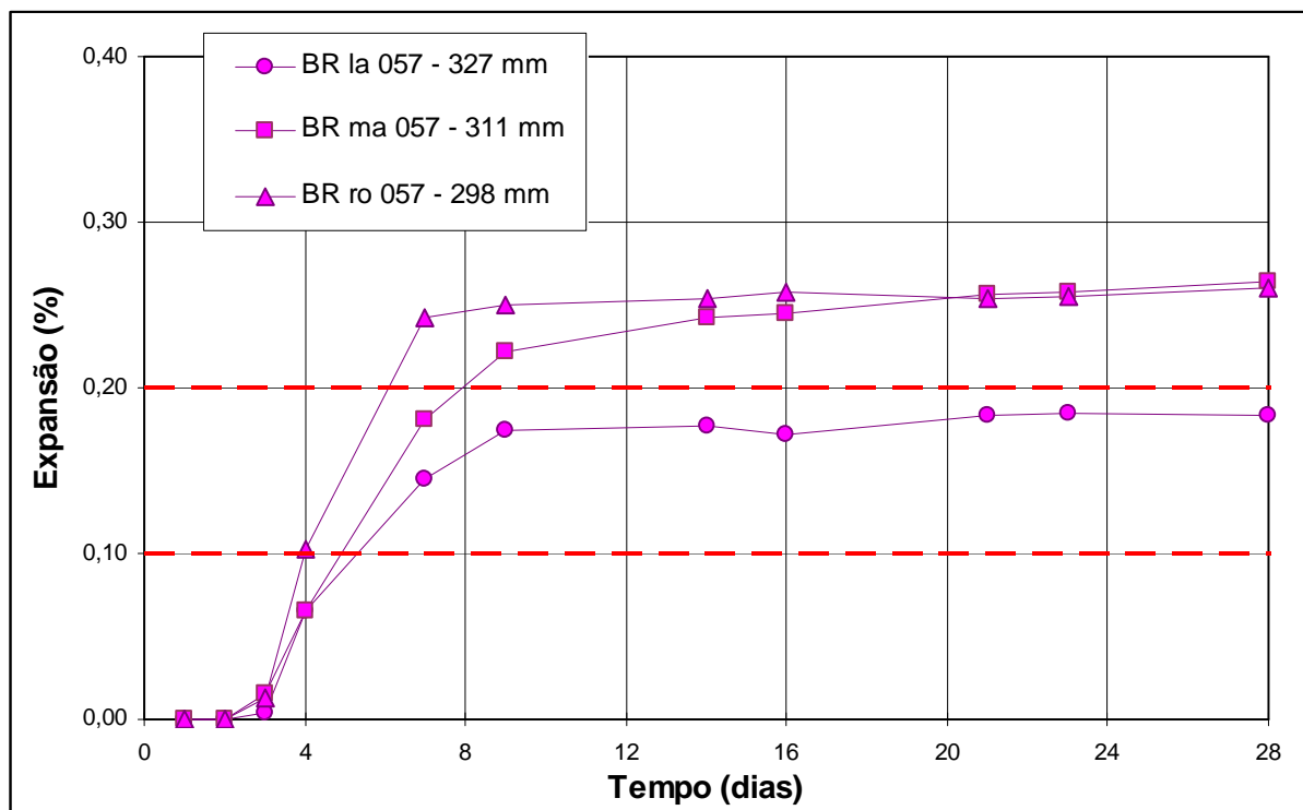
Figura 70: expansões até 28 dias da rocha BR, relação a/c 0,57, três moagens (S1).
