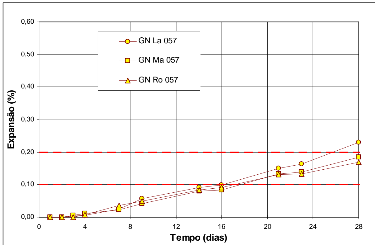
Figura 74: expansões até 28 dias da rocha GN, relação a/c 0,57, três moagens (S2).
