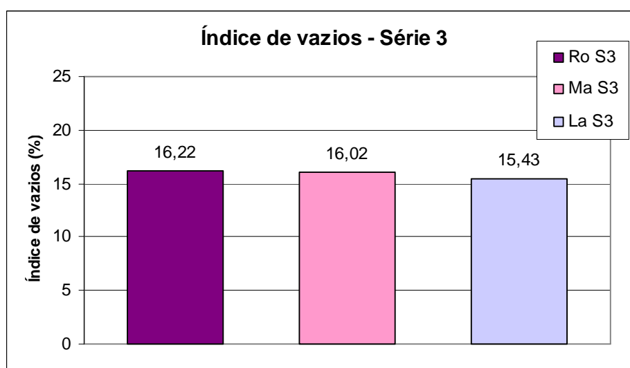
Figura 124: índice de vazios (médias) da Série 3.
