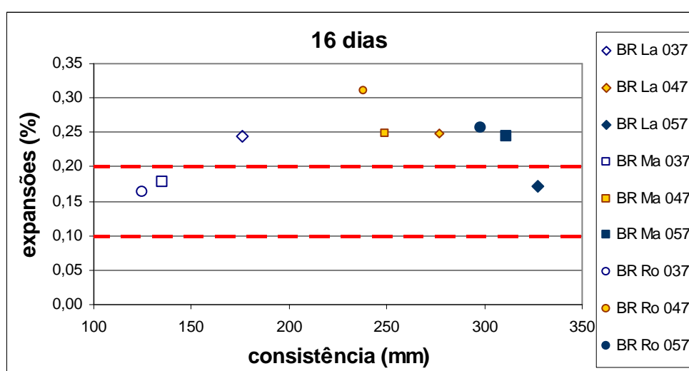
Figura 99: comparativo entre os dados da série 1, rocha BR, 16 dias.
