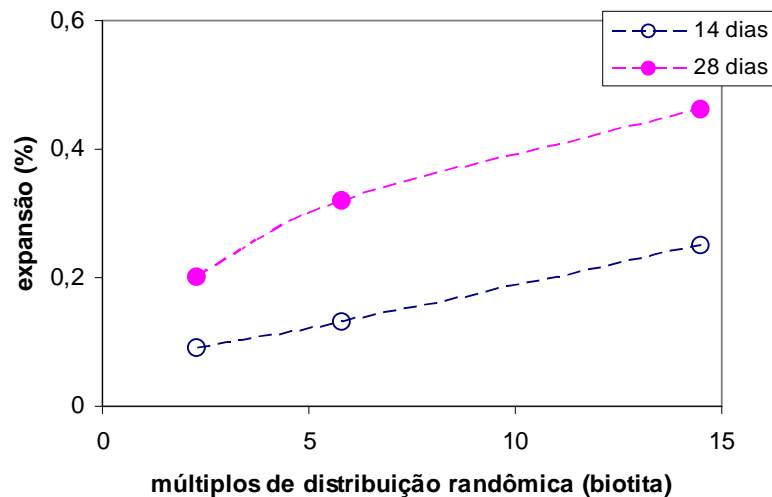
Figura 19: correlação entre expansões medidas pela ASTM C – 1260 e a textura da rocha, adaptado de Monteiro et al. (2001).
