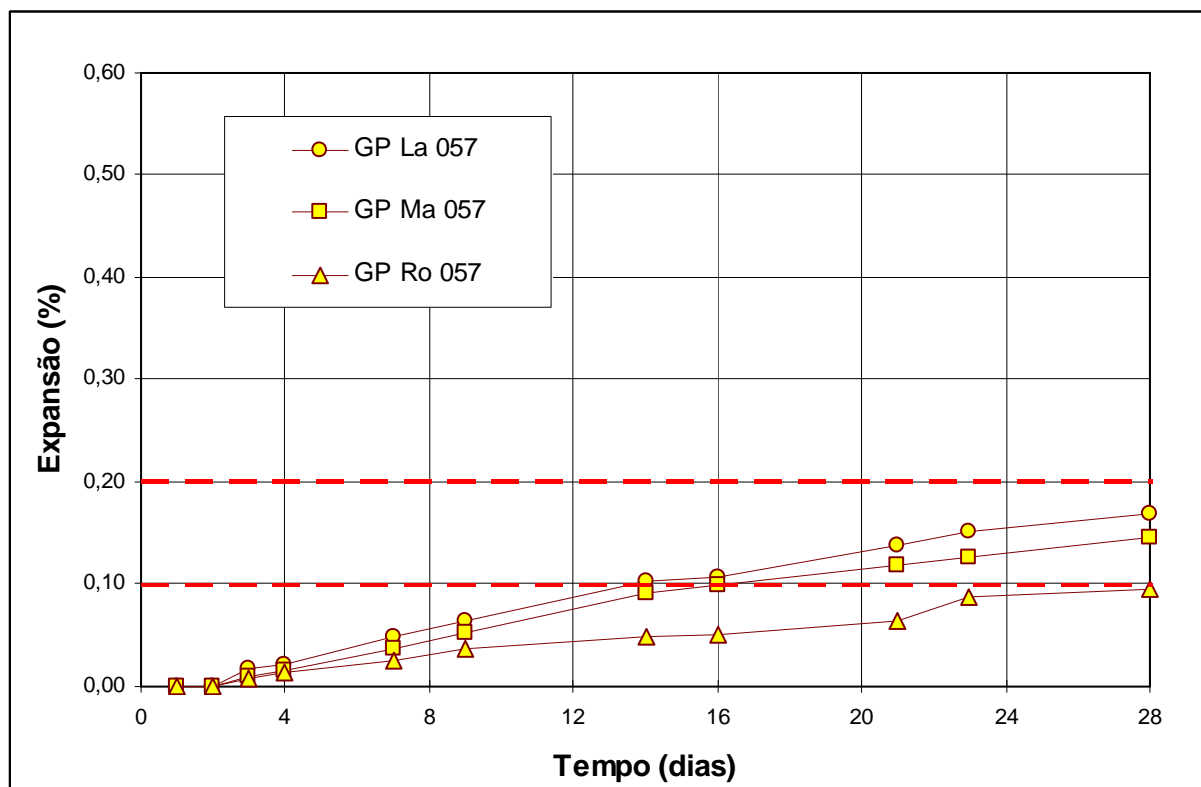
Figura 78: expansões até 28 dias da rocha GP, relação a/c 0,57, três moagens (S2).
