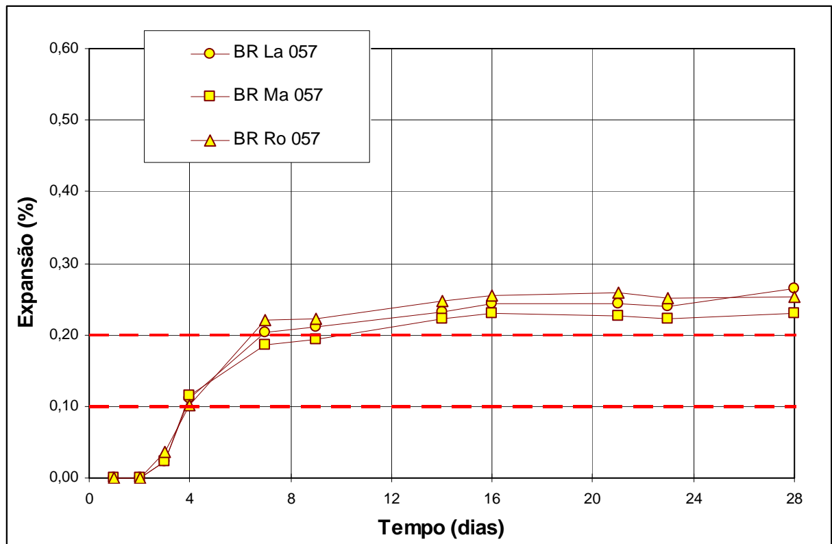
Figura 82: expansões até 28 dias da rocha BR, relação a/c 0,57, três moagens (S2).
