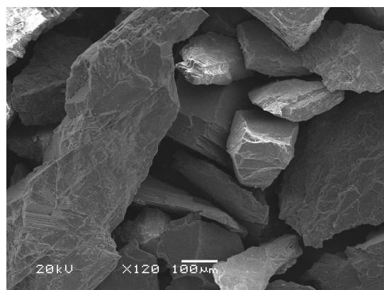
Figura 45: amostra GN Ro, aumento de 120x.
