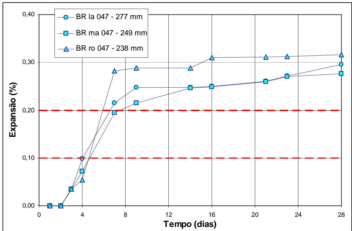
Figura 69: expansões até 28 dias da rocha BR, relação a/c 0,47, três moagens (S1).
