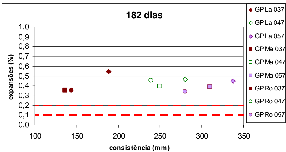
Figura 98: comparativo entre os dados da série 1, rocha GP, 182 dias.
