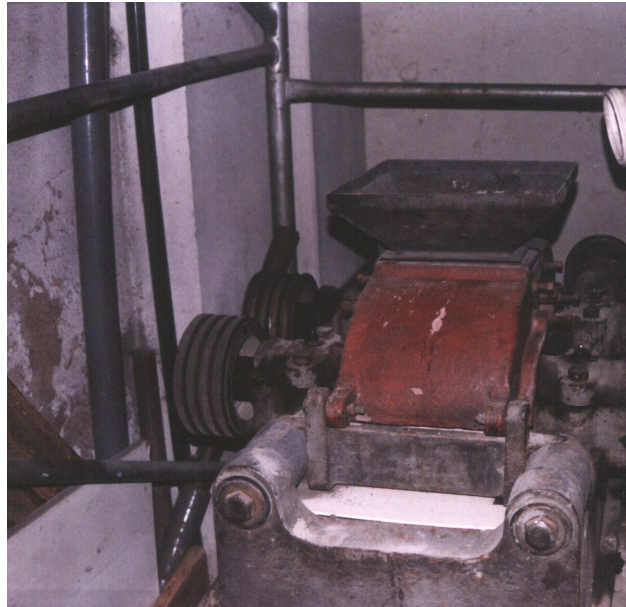
Figura 29: moinho de rolos empregado na pesquisa (UFRGS).
