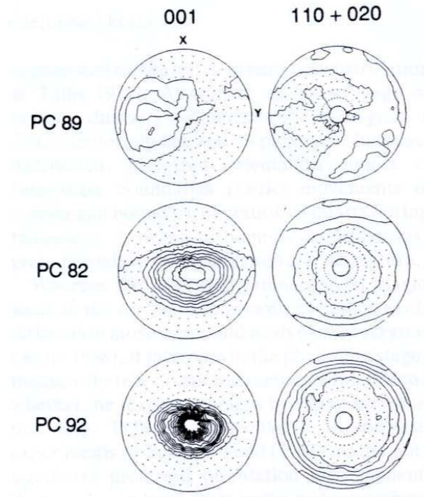
Figura 18: figuras de pólo para o mineral biotita. (WENK e PANNETIER, 1990).
