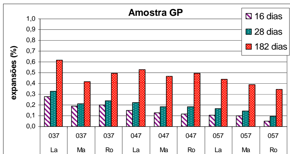
Figura 103: comparativo entre os dados da série 2, rocha GP.
