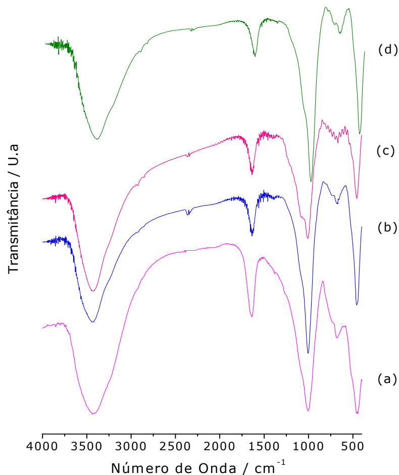
Figura 3.37 – Espectro na região do infravermelho da vermiculita sódica (a) e trocada com os metais cobre (b), cobalto (c) e níquel (d).
