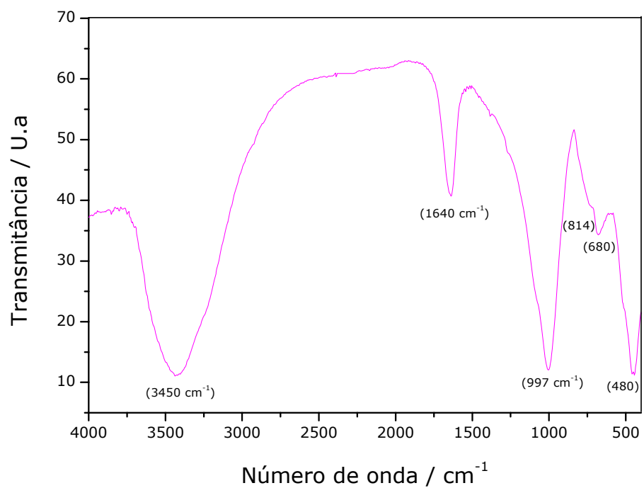
Figura 3.4 - Espectro na região do infravermelho da vermiculita sódica.
