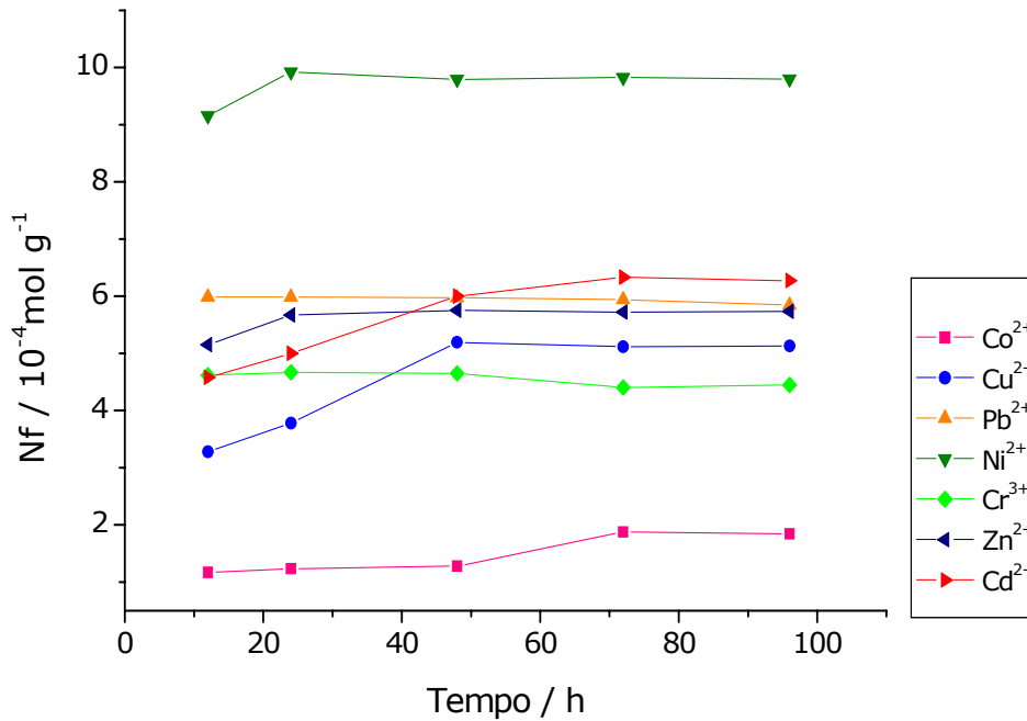
Figura 3.14 - Isothermas de tempo dos metais pesados em vermiculita a 298,15 K e 1 atm.
