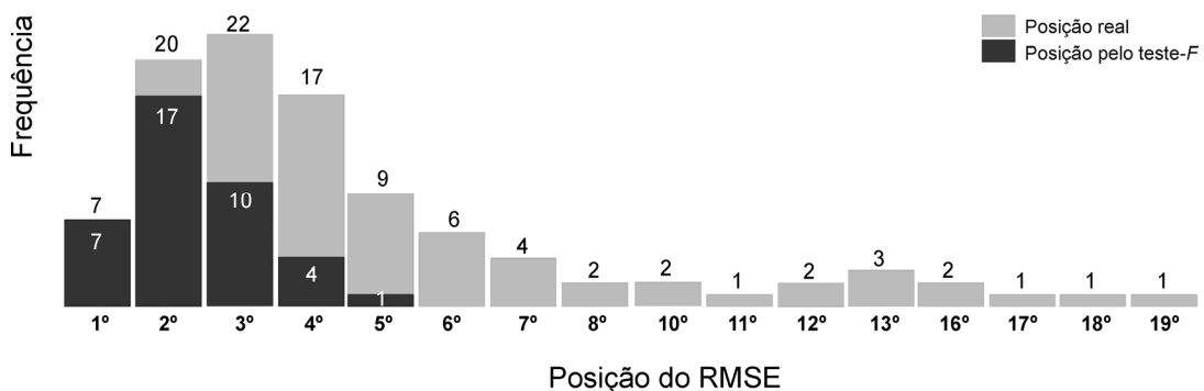
Figura 4.16 Gráfico de barras apresentando a posição da wavelet selecionada pelo MDL para cada um dos cem sinais gerados, com relação ao RMSE obtido.
