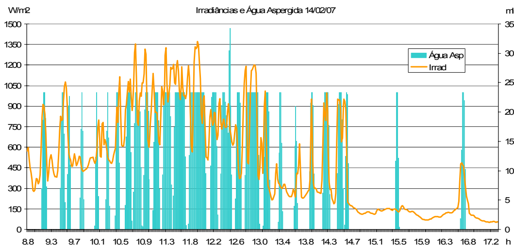
Figura 59: Volumes de Água Aspergidos e Irradiâncias em 14/02/07
