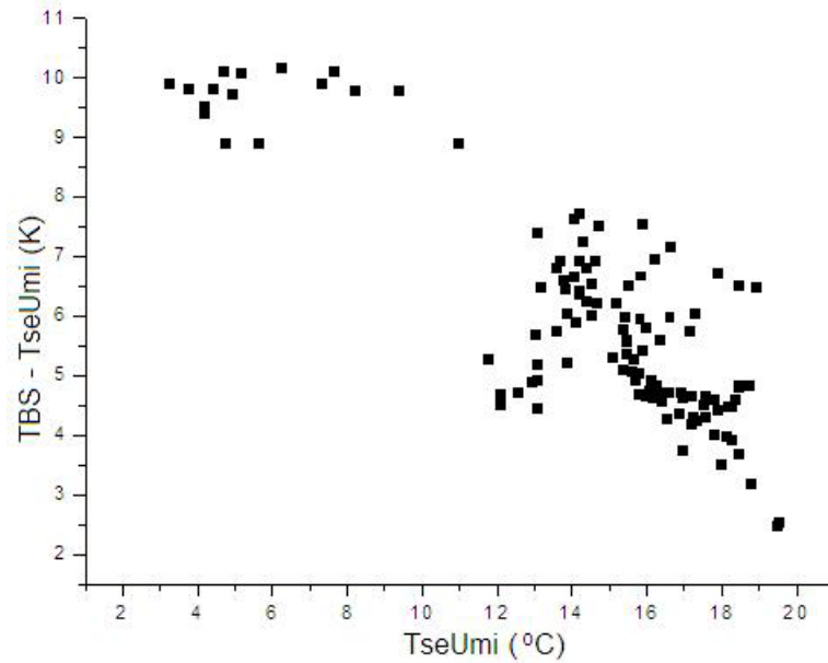
Figura 78: Diferença entre TBS e TseUmi x Temperatura da Superfície (TseUmi)
