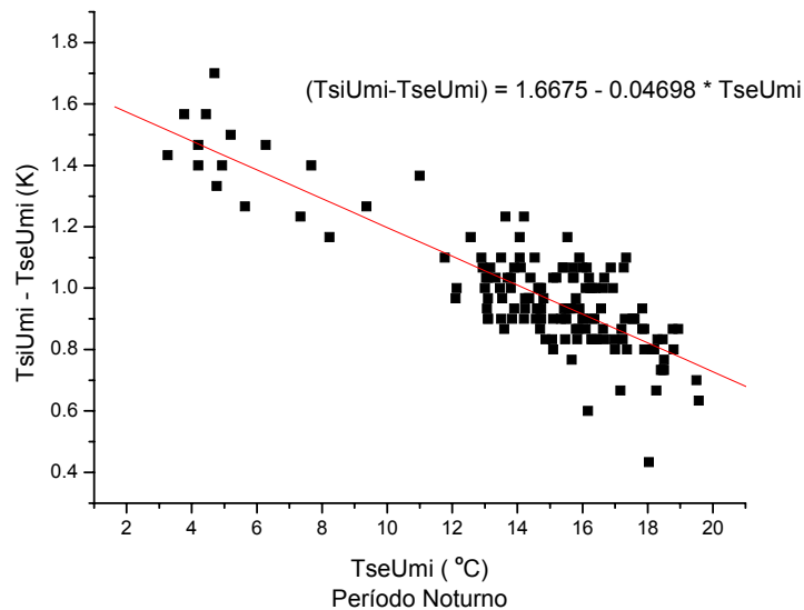
Figura 82: Diferença entre as Temperaturas Superficiais x Temperatura Superficial Externa.
