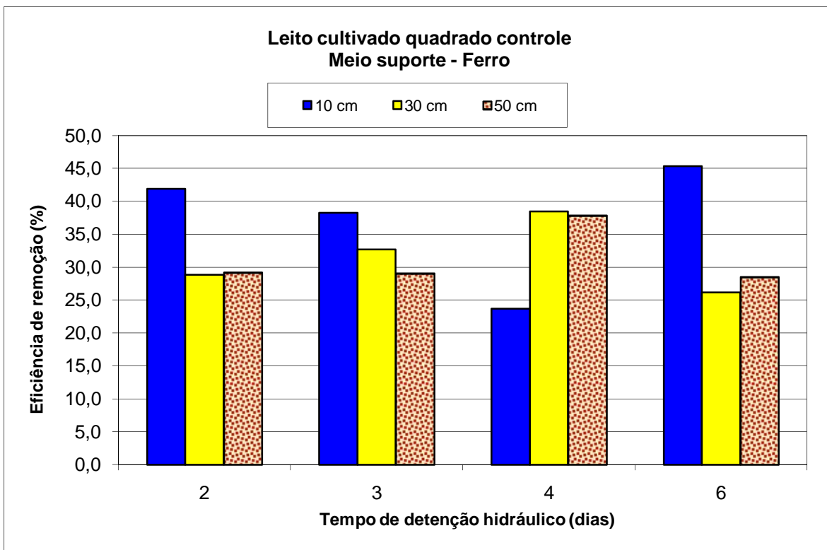
Figura 5.22 - Eficiência média de remoção do Fe pelo meio suporte a diferentes profundidades e tempos de detenção hidráulico, no leito cultivado controle quadrado.
