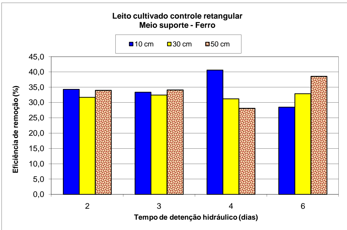
Figura 5.42 - Eficiência média de remoção do Fe pelo meio suporte a diferentes profundidades e tempos de detenção hidráulica, no leito cultivado controle retangular.
