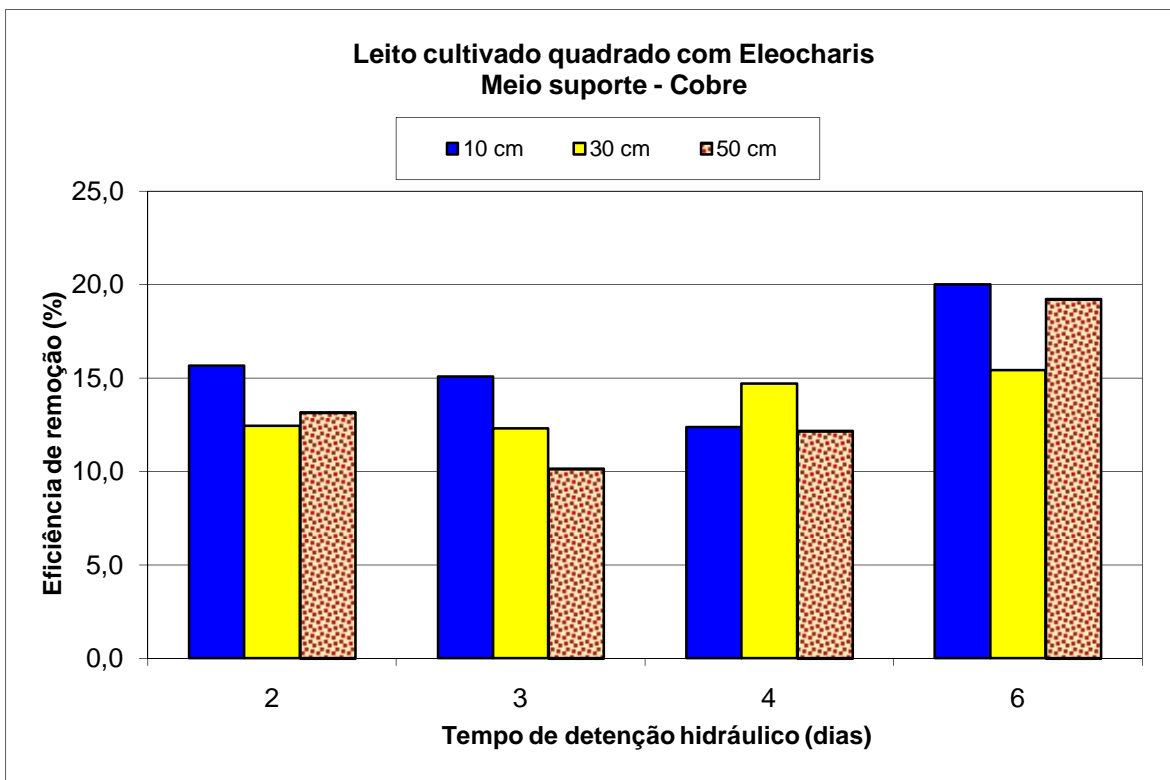
Figura 5.10 - Eficiência média de remoção do Cu pelo meio suporte a diferentes profundidades e tempos de detenção hidráulica, no leito cultivado quadrado com Eleocharis sp.
