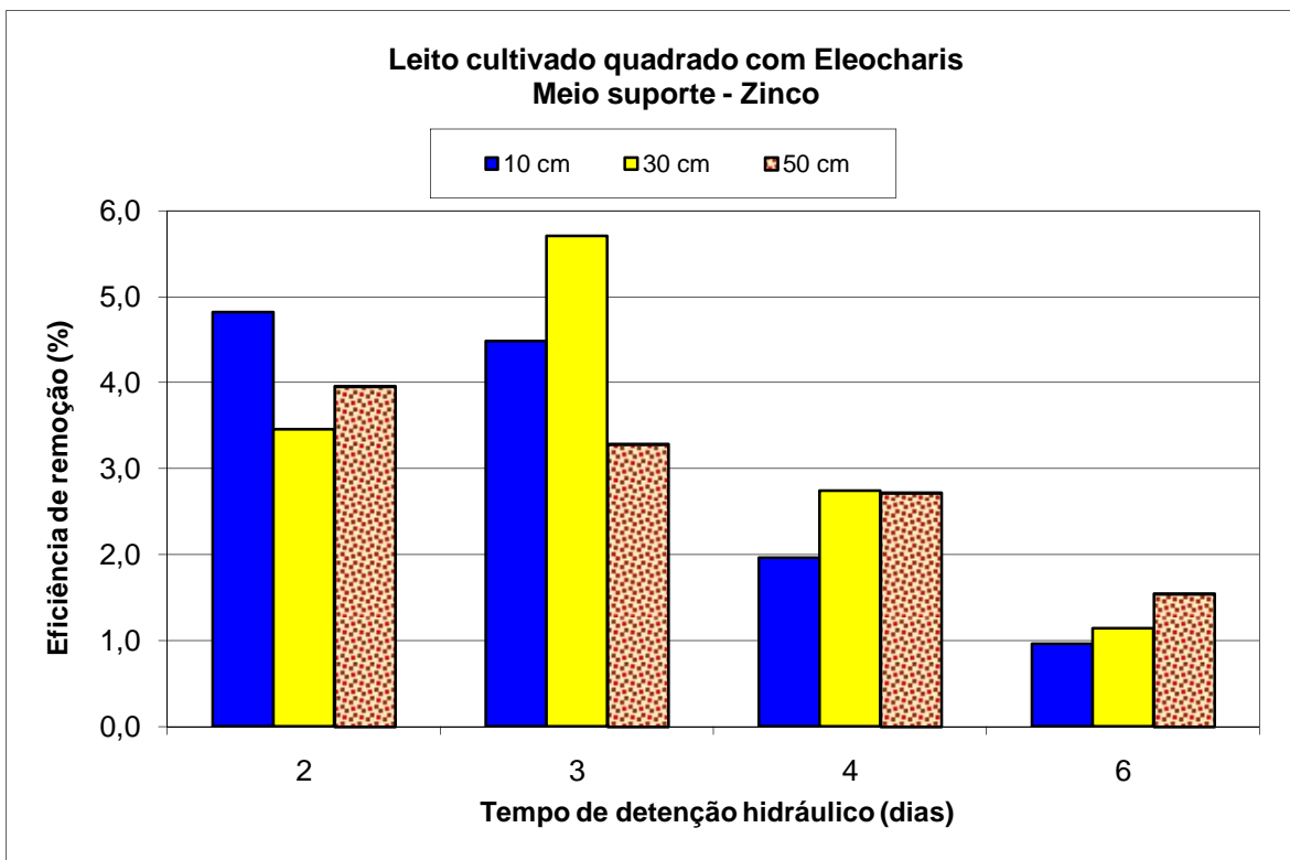
Figura 5.11 - Eficiência média de remoção do Zn pelo meio suporte a diferentes profundidades e tempos de retenção hidráulica, no leito cultivado quadrado com Eleocharis sp.
