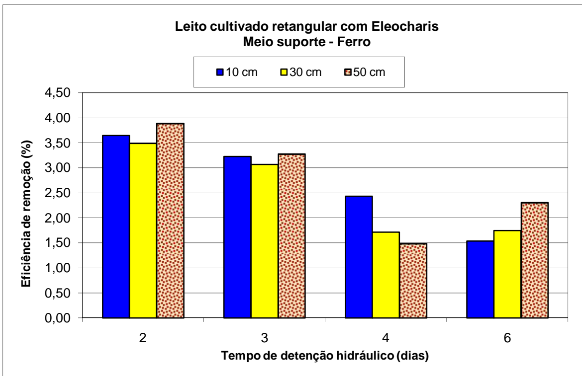
Figura 5.29 - Eficiência média de remoção do Fe pelo meio suporte a diferentes profundidades e tempos de detenção hidráulica, no leito cultivado retangular com Eleocharis sp.
