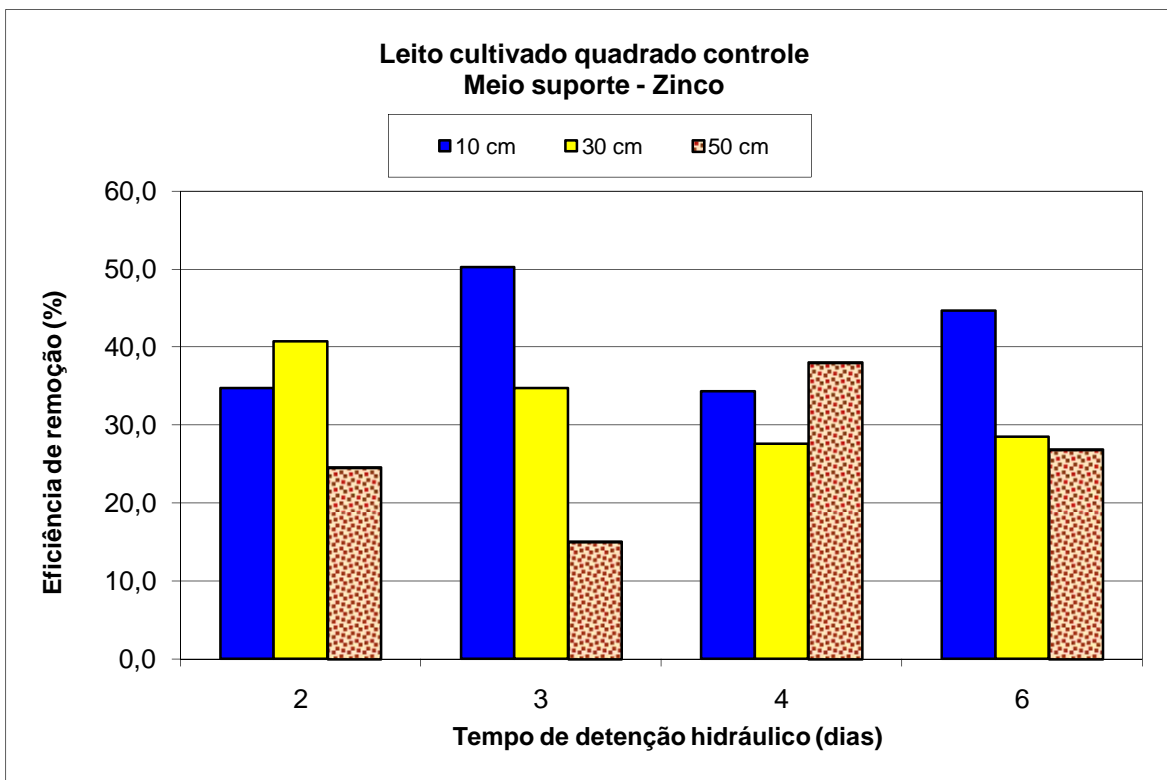
Figura 5.24 - Eficiência média de remoção do Zn pelo meio suporte a diferentes profundidades e tempos de detenção hidráulica, no leito cultivado controle quadrado.
