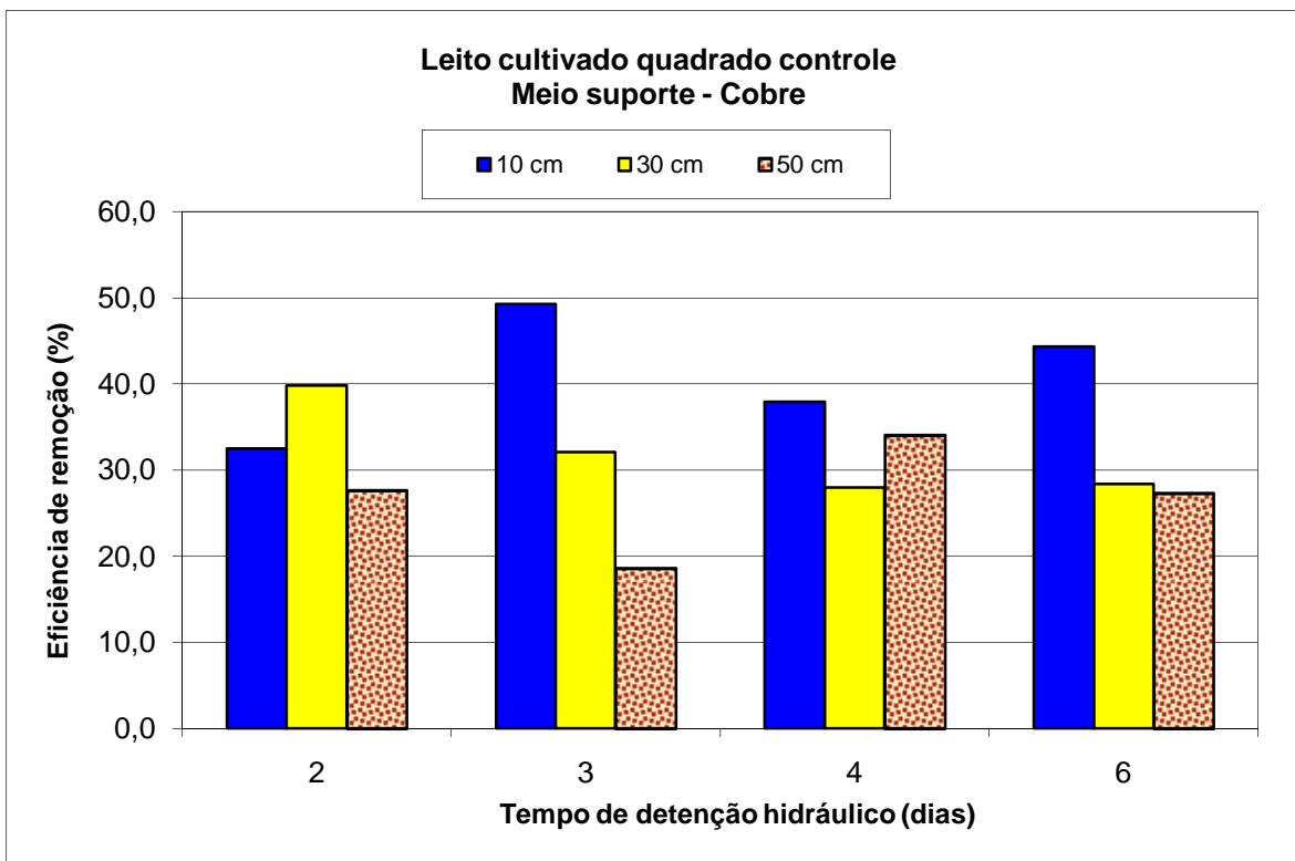
Figura 5.23 - Eficiência média de remoção do Cu pelo meio suporte a diferentes profundidades e tempos de detenção hidráulica, no leito cultivado controle quadrado.
