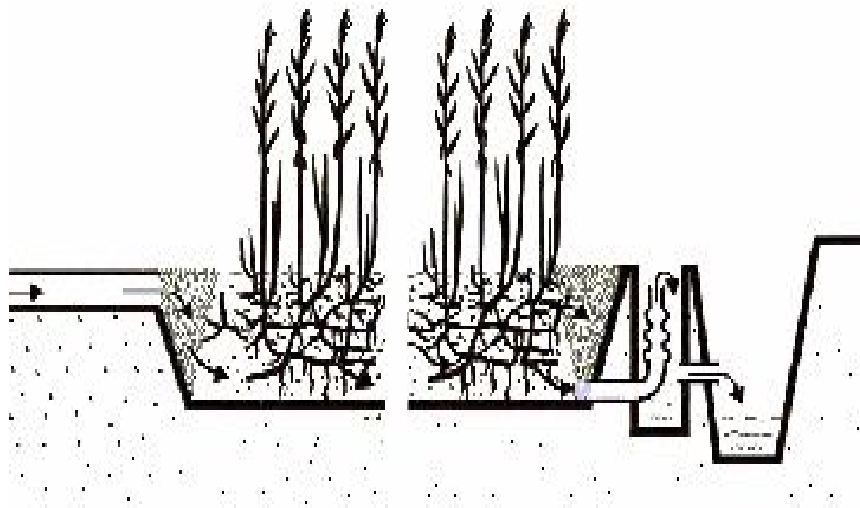
Figura 3.2 - Representação esquemática de um Leito Cultivado de Fluxo Subsuperficial horizontal com macrófitas aquáticas emergentes, ilustra-se a espécie Phragmites australis (BRIX, 1993).
