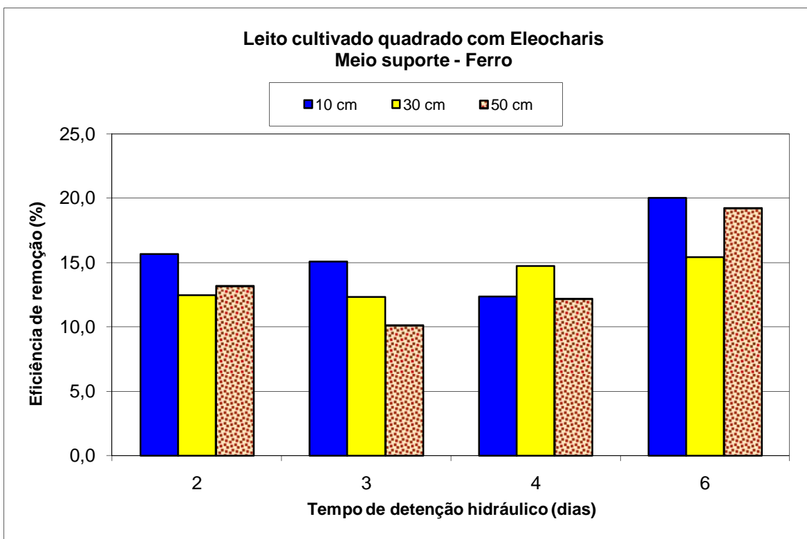
Figura 5.9 - Eficiência média de remoção do Fe pelo meio suporte a diferentes profundidades e tempos de detenção hidráulica, no leito cultivado quadrado com Eleocharis sp.
