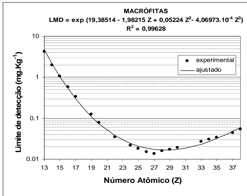
Figura 5.4 - Limite mínimo de detecção para os elementos da série K contidos nas amostras das folhas das macrófitas por SR-TXRF.
