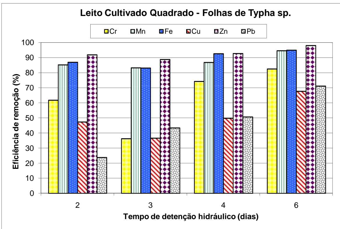
Figura 5.13 - Eficiência de remoção média para Cr, Mn, Fe, Cu, Zn e Pb pelas folhas da macrófita Typha sp no leito cultivado quadrado com diferentes tempos de detenção hidráulica.
