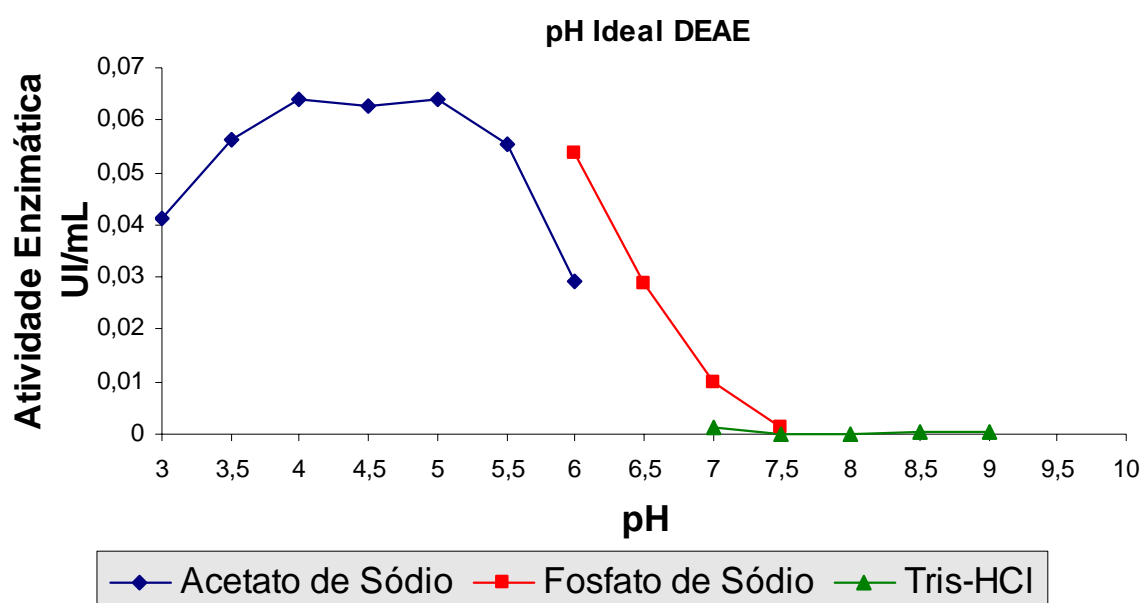
Figura 18: Efeito do pH na atividade de alfa-galactosidase do eluato da DEAE-Sepharose obtido de sementes de Guapuruvu germinadas por 48 horas.
