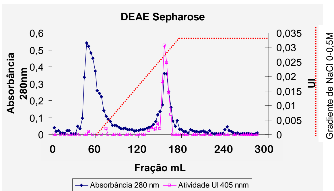
Figura 10 – Perfil cromatográfico em coluna de DEAE Sepharose, do extrato enzimático contendo atividade de alfa-galactosidase proveniente de cromatografia de exclusão molecular Sephadex-G75.
