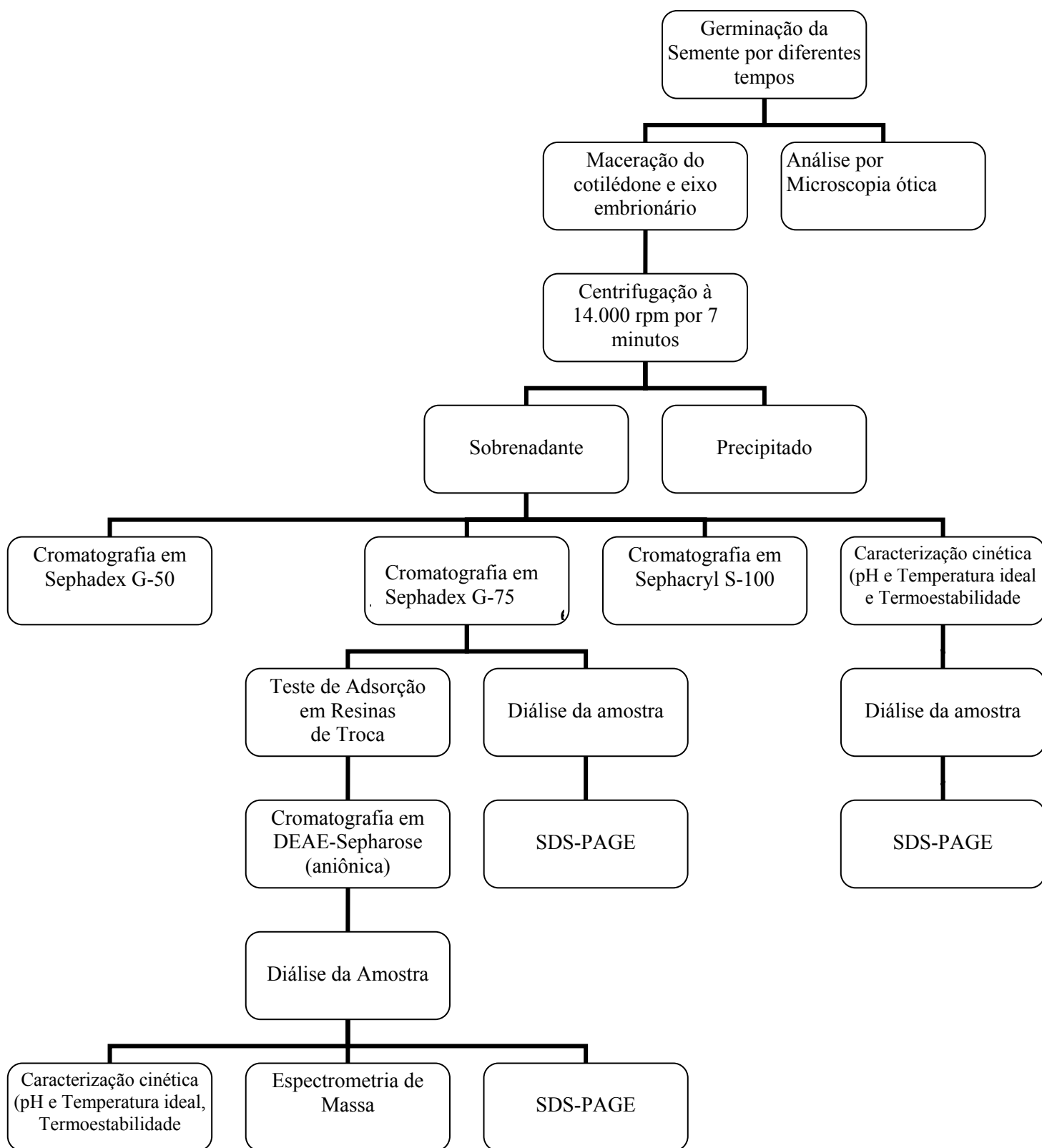
Figura 34 - Fluxograma de purificação parcial da alfa-galactosidase de sementes de Guapuruvu.
