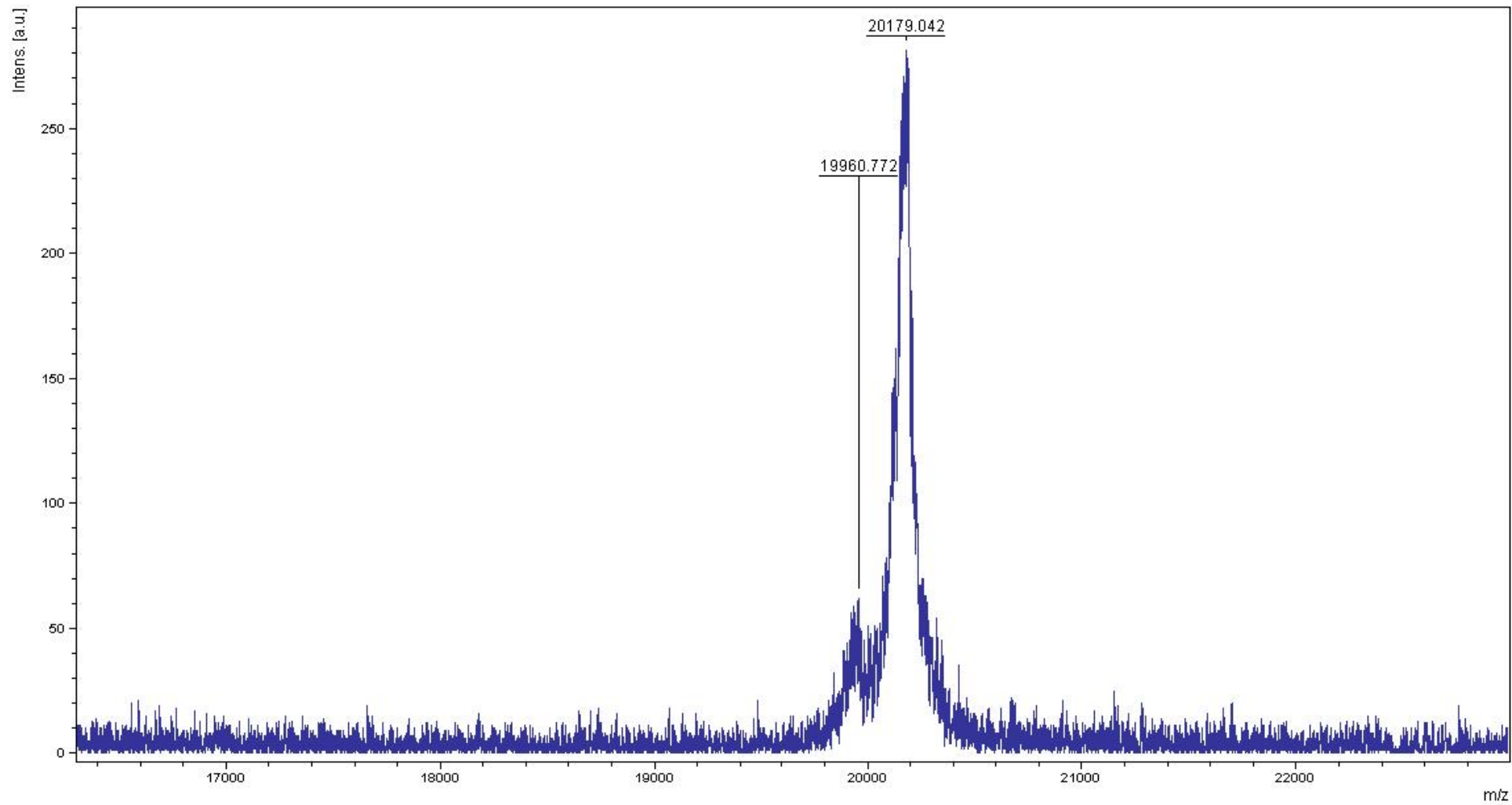
Figura 14 – Espectro de massa da amostra enzimática proveniente da coluna DEAE Sepharose. Aproximação do pico com massa 20179,042 Daltons.
