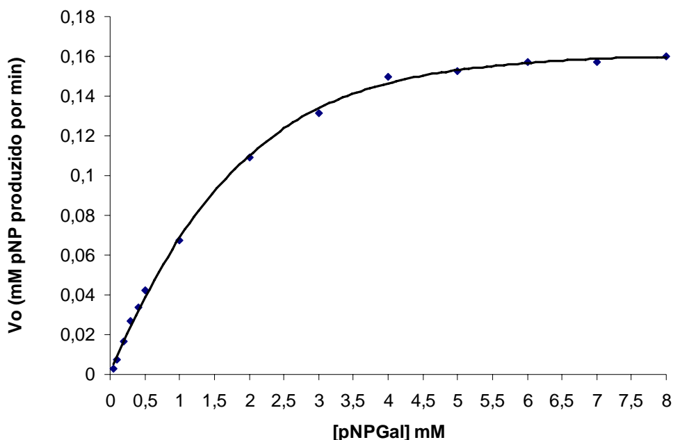
Figura 33 – Efeito da concentração do substrato na velocidade da hidrólise pNPGal, os valores de obtidos de K_M e V_{max} foram 1,68mM 0,182 micromol.min, respectivamente
