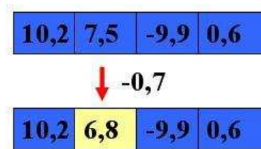
Figura 3.9: Mutação Real
