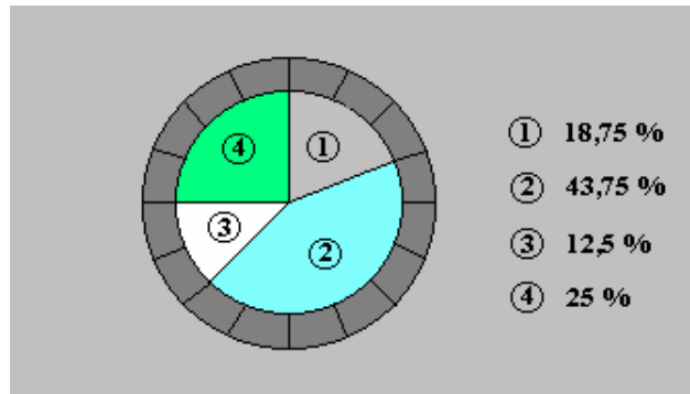
Figura 3.3: Roleta
