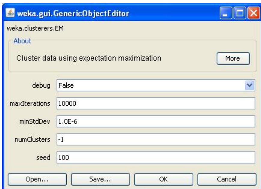
Figura 21 - Parâmetros do Algoritmo EM
