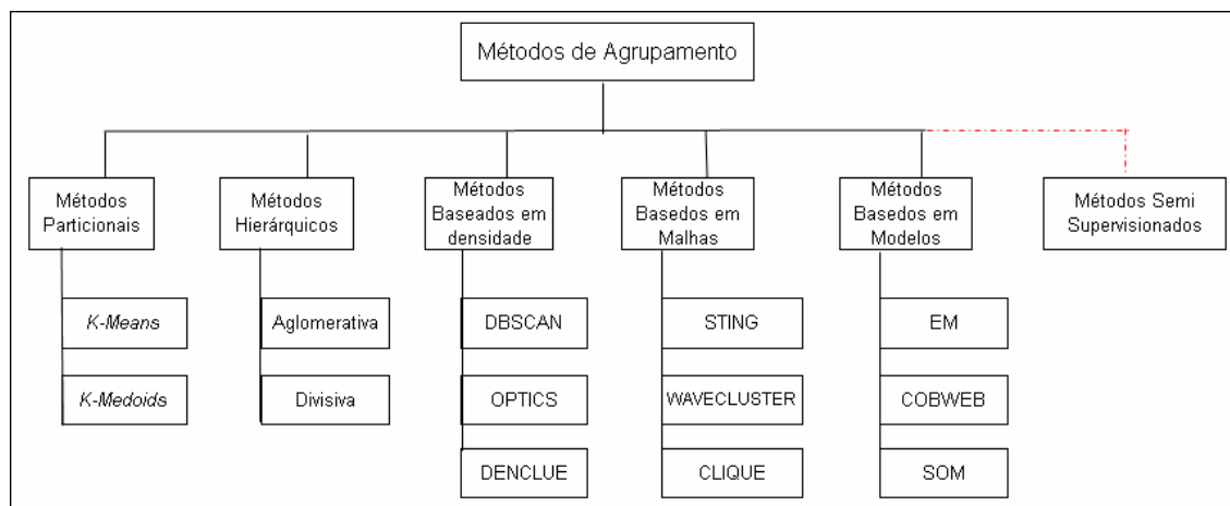
Figura 8 - Métodos de Agrupamentos
