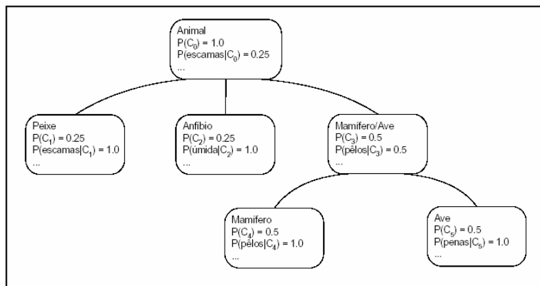
Figura 5 - Árvore de Classificação
