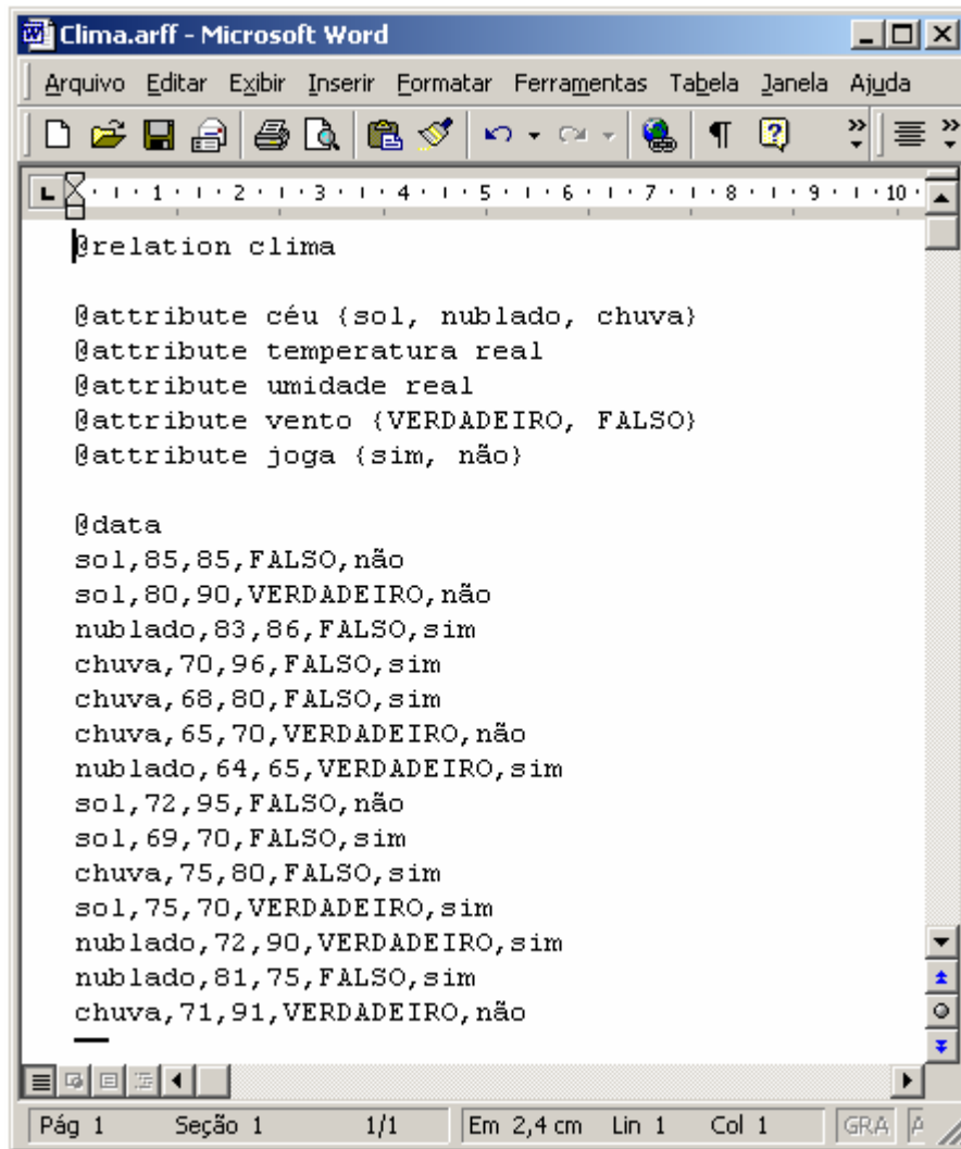
Figura 11 - Arquivo no Formato ARFF
