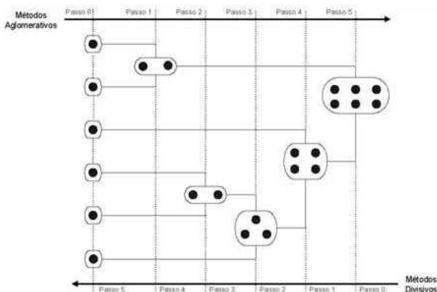
Figura 4 - Segmentação Aglomerativos e Divisivos( HAN & KAMBLER,2006)
