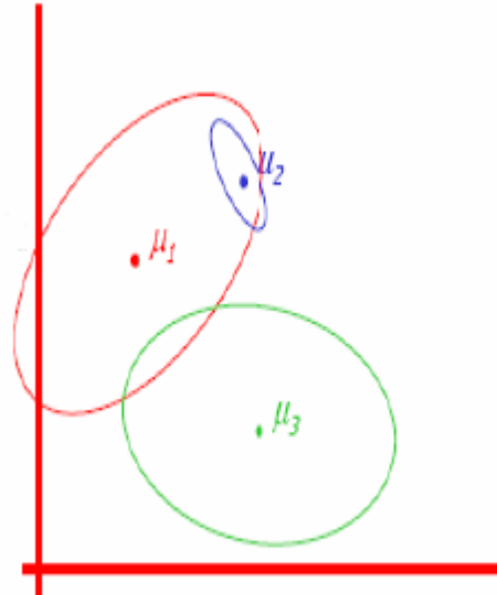
Figura 7 - Gaussianas Elípticas (ZADROZNY, 2006)
