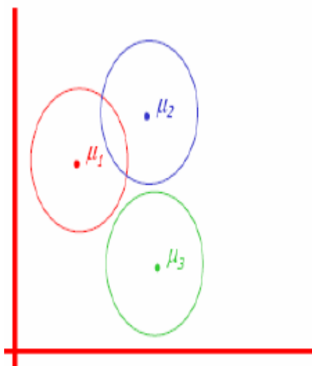
Figura 6 - Gaussianas Circulares (ZADROZNY, 2006)
