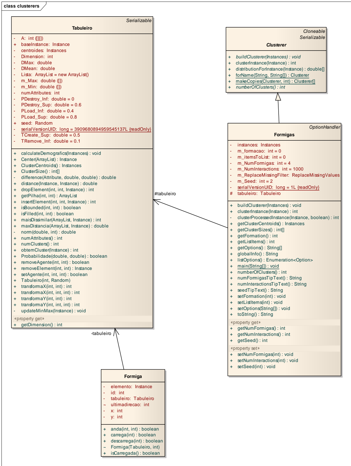
Figura 10 - Diagrama de Classe
