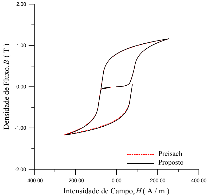
Fig. 5.15. Laços para U_e = 60 \text{ V} , \theta_1 = 0^\circ (energização), \theta_2 = 180^\circ (religamento).
