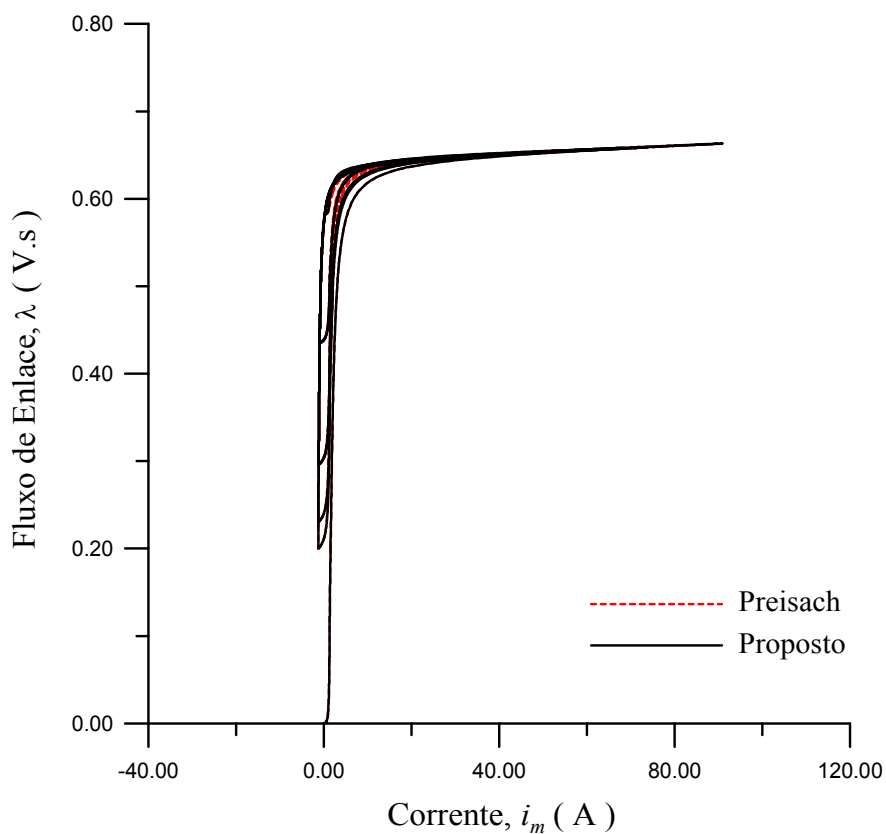
Fig. 6.30. Laços assimétricos para carga de 1,59 + j 0,20 \Omega .
