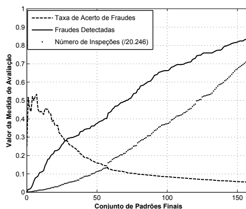
Figura 6.19: Resultado das medidas de avaliação TAF , FD e NI para o Conjunto 4.2.
