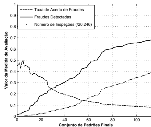
Figura 6.20: Resultado das medidas de avaliação TAF , FD e NI para o Conjunto 4.3.
