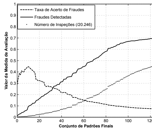
Figura 6.21: Resultado das medidas de avaliação TAF , FD e NI para o Conjunto 4.4.
