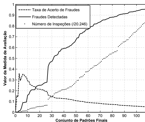
Figura 6.13: Resultado das medidas de avaliação TAF , FD e NI para o Conjunto 3.3.
