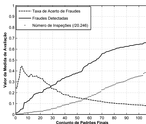
Figura 6.2: Resultado das medidas de avaliação TAF , FD e NI para Teste B.
