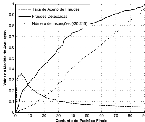
Figura 6.10: Resultado das medidas de avaliação TAF , FD e NI para o Conjunto 2.5.
