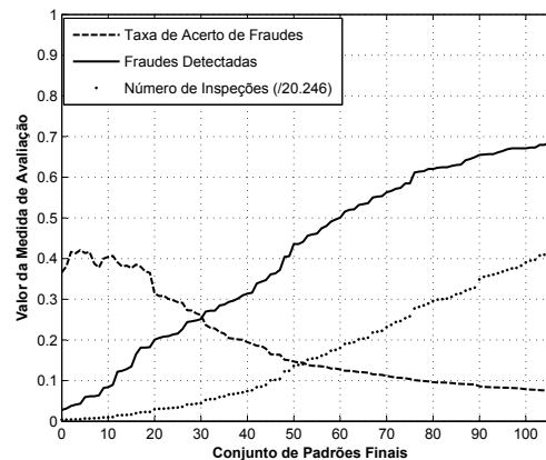
Figura 6.4: Resultado das medidas de avaliação TAF , FD e NI para Teste D.
