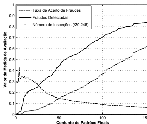
Figura 6.16: Resultado das medidas de avaliação TAF , FD e NI para o Conjunto 3.6.
