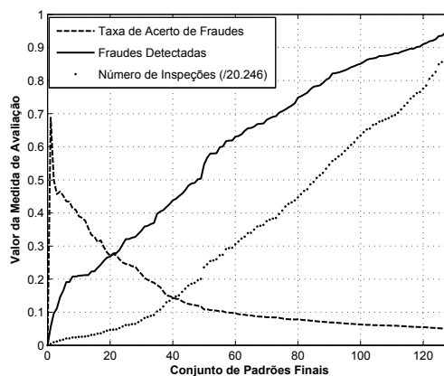
Figura 6.15: Resultado das medidas de avaliação TAF , FD e NI para o Conjunto 3.5.
