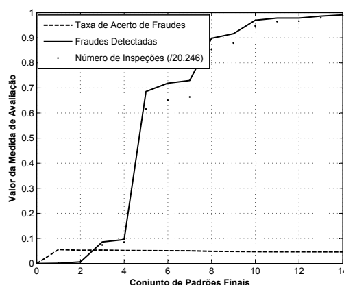
Figura 6.9: Resultado das medidas de avaliação TAF , FD e NI para o Conjunto 2.4.
