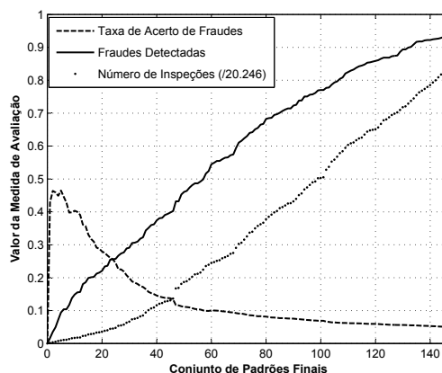
Figura 6.14: Resultado das medidas de avaliação TAF , FD e NI para o Conjunto 3.4.
