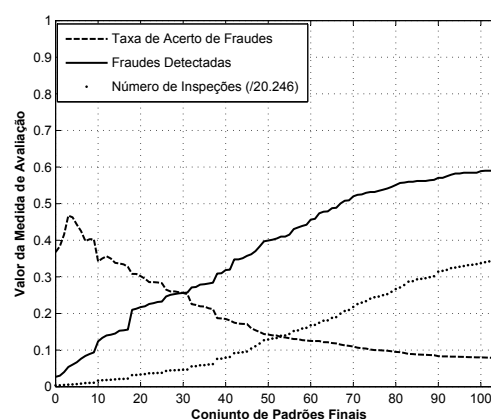
Figura 6.23: Resultado das medidas de avaliação TAF , FD e NI para o Conjunto 5.2.
