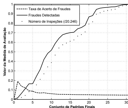
Figura 6.7: Resultado das medidas de avaliação TAF , FD e NI para o Conjunto 2.2.
