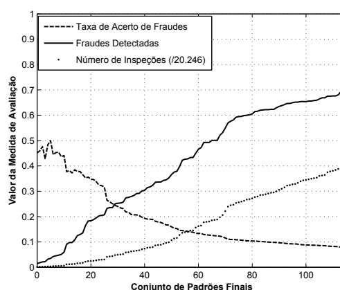
Figura 6.3: Resultado das medidas de avaliação TAF , FD e NI para Teste C.
