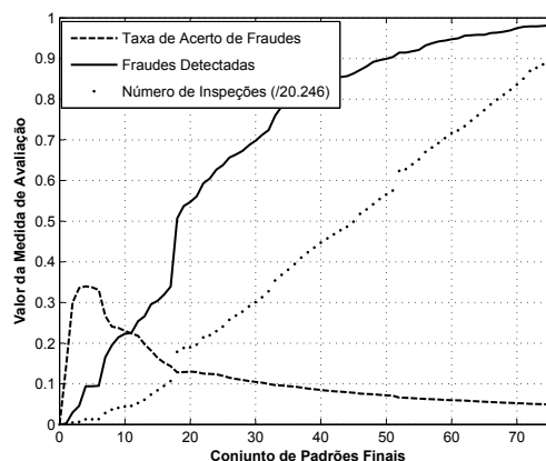
Figura 6.6: Resultado das medidas de avaliação TAF , FD e NI para o Conjunto 2.1.
