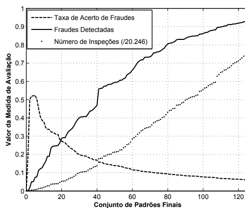
Figura 6.11: Resultado das medidas de avaliação TAF , FD e NI para o Conjunto 3.1.
