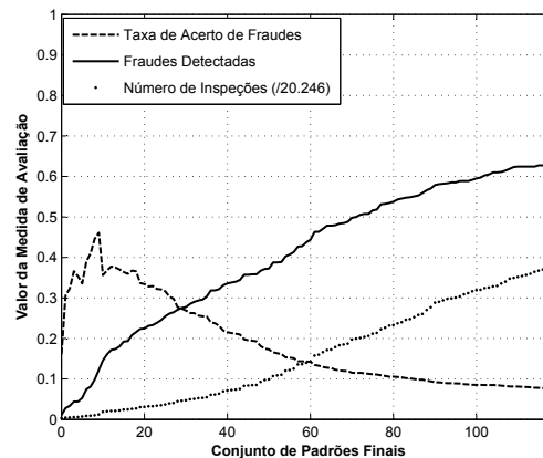
Figura 6.22: Resultado das medidas de avaliação TAF , FD e NI para o Conjunto 5.1.
