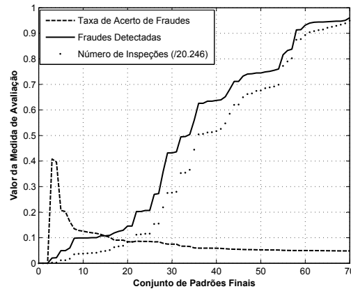
Figura 6.17: Resultado das medidas de avaliação TAF , FD e NI para o Conjunto 3.7.
