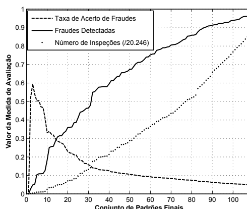
Figura 6.12: Resultado das medidas de avaliação TAF , FD e NI para o Conjunto 3.2.
