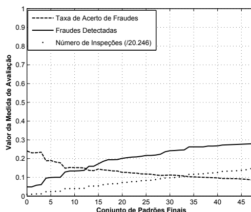
Figura 6.24: Resultado das medidas de avaliação TAF , FD e NI para o Conjunto 5.3.
