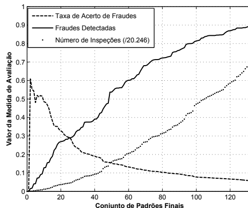
Figura 6.18: Resultado das medidas de avaliação TAF , FD e NI para o Conjunto 4.1.
