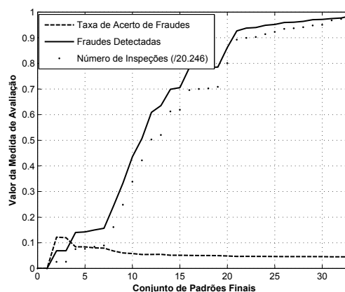
Figura 6.8: Resultado das medidas de avaliação TAF , FD e NI para o Conjunto 2.3.
