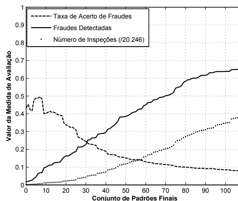
Figura 6.1: Resultado das medidas de avaliação TAF , FD e NI para Teste A
