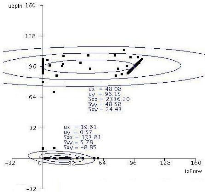
Figura 4-4 - Modelagem com periodicidade de consulta de 3 segundos.
