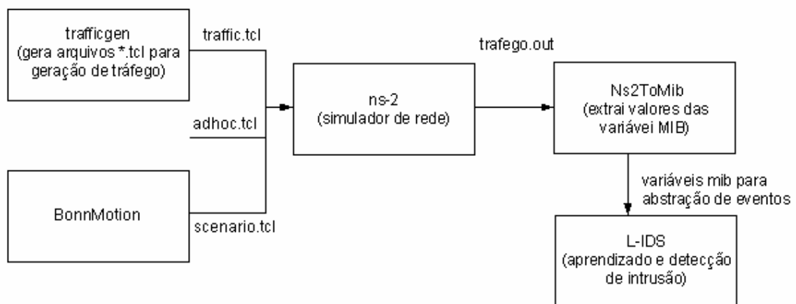
Figura 4-1 – Processo de geração da simulação
