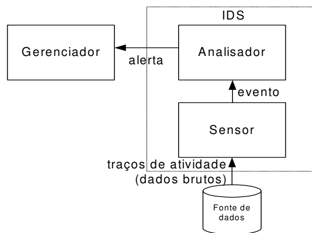
Figura 2-1 – Framework de detecção de intrusão do IDWG
