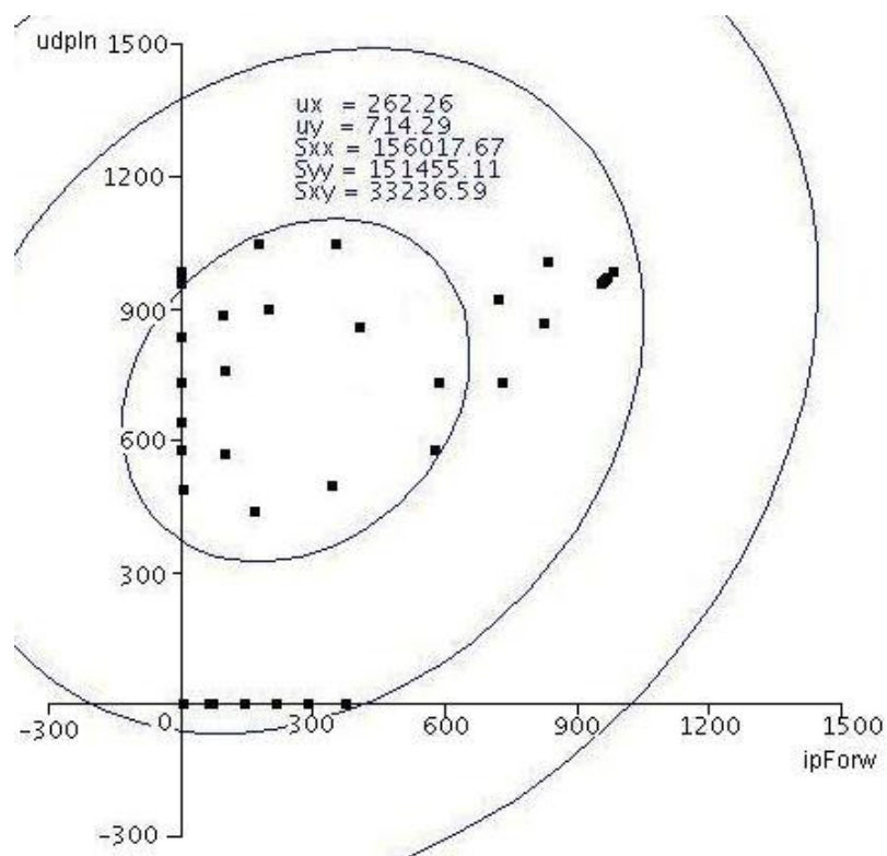
Figura 4-5 - Modelagem com periodicidade de consulta de 30 segundos.
