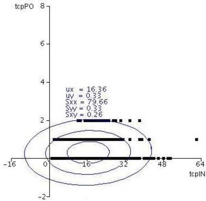
Figura 4-9 – Modelagem com periodicidade de consulta de 0,3 segundos.
