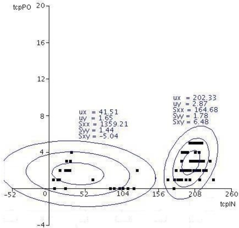
Figura 4-10 - Modelagem com periodicidade de consulta de 3 segundos.
