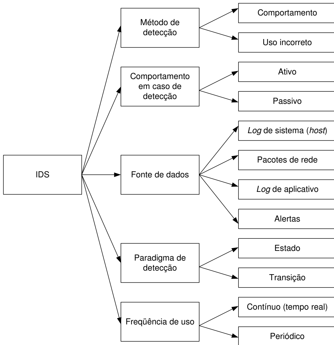
Figura 2-2 – Taxionomia dos Sistemas de Detecção de Intrusão (Fonte: R. Puttini [1] p. 39)
