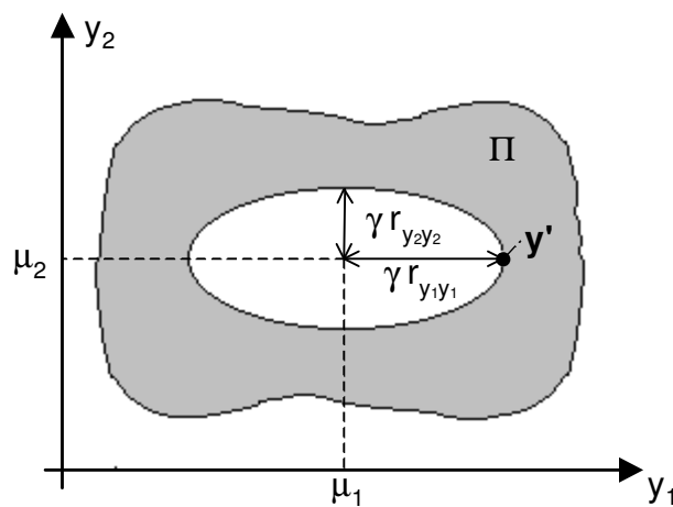
Figura 3-2 - \Pi para um cluster com distribuição Gaussiana bivariada e matriz de covariância diagonal (Fonte: R. Puttini [1] p. 127)
