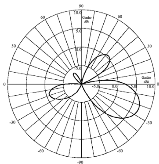
DIAGRAMA DE ELEVAÇÃO (ESPAÇO LIVRE) FREQUÊNCIA: 26 MHz
