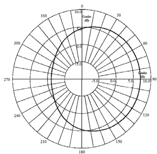
DIAGRAMA DE AZIMUTE (ESPAÇO LIVRE) FREQUÊNCIA: 26 MHz
