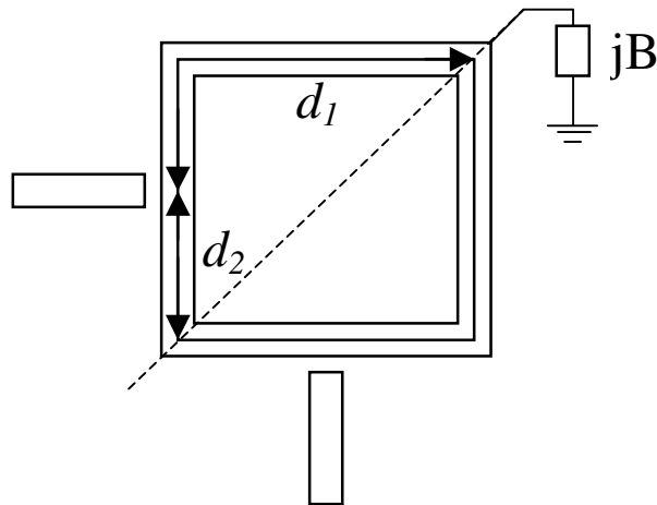
Figura 5.9 Modelo do ressoador anel quadrado com a adição de uma perturbação.
