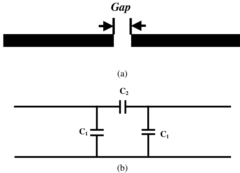
Figura 3.4 – (a) Acoplamento end-to-end e (b) circuito equivalente do acoplamento end-to-end .
