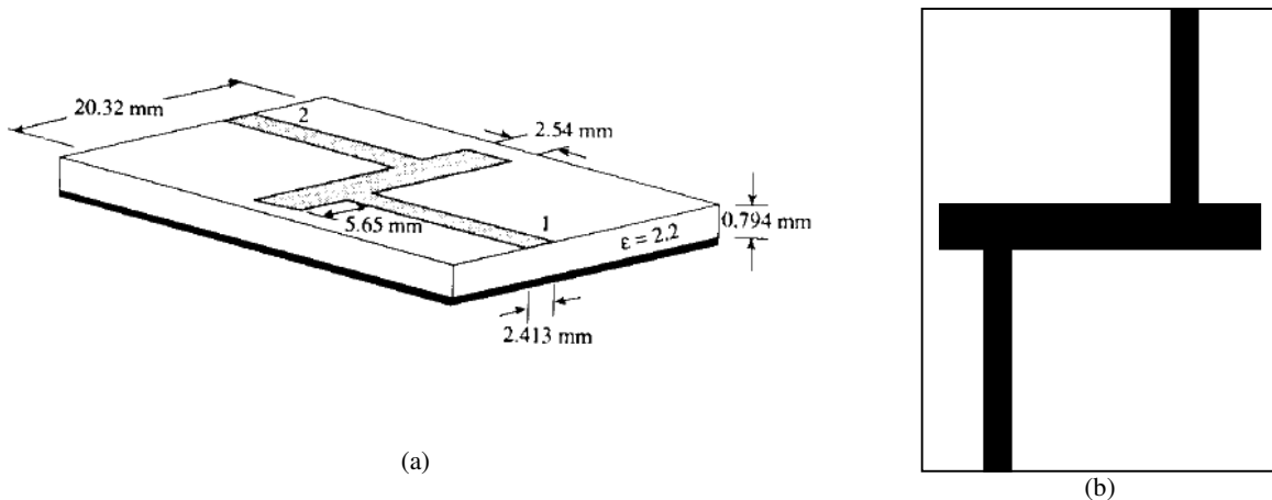
Figura 2.11 Estrutura utilizada para validar o software . (a) dimensões. (b) estrutura no plano xy
