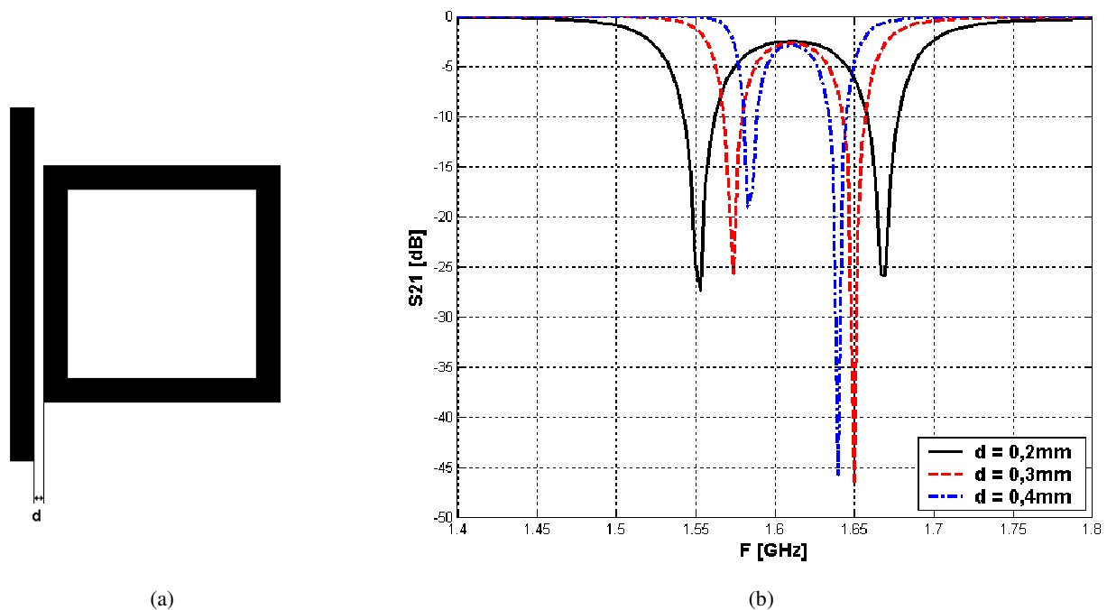
Figura 4.14 Efeito da variação da distância entre a linha de alimentação e o ressoador.
