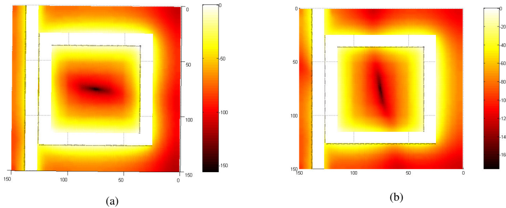
Figura 4.13 Distribuição de campo magnético para o ressonador da Figura 4.11: (a) 1,57 GHz. (b) 1,65 GHz. Os valores do campo H foram normalizados e expressos em dB.
