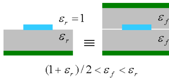
Figura 2.5 - Constante dielétrica efetiva.
