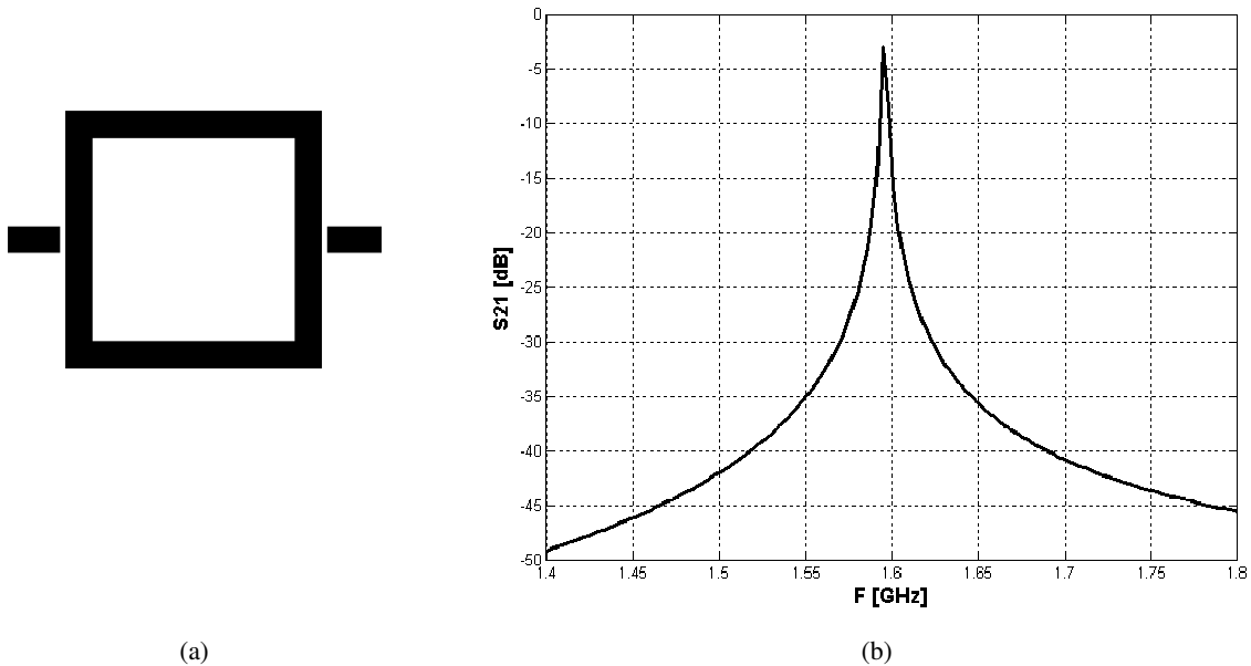
Figura 4.6 Ressorador em anel alimentado por gap . (a) Estrutura. (b) Parâmetro S_{21} em função da frequência nas proximidades do modo fundamental do ressoador. Valor do gap = 0,8 mm.
