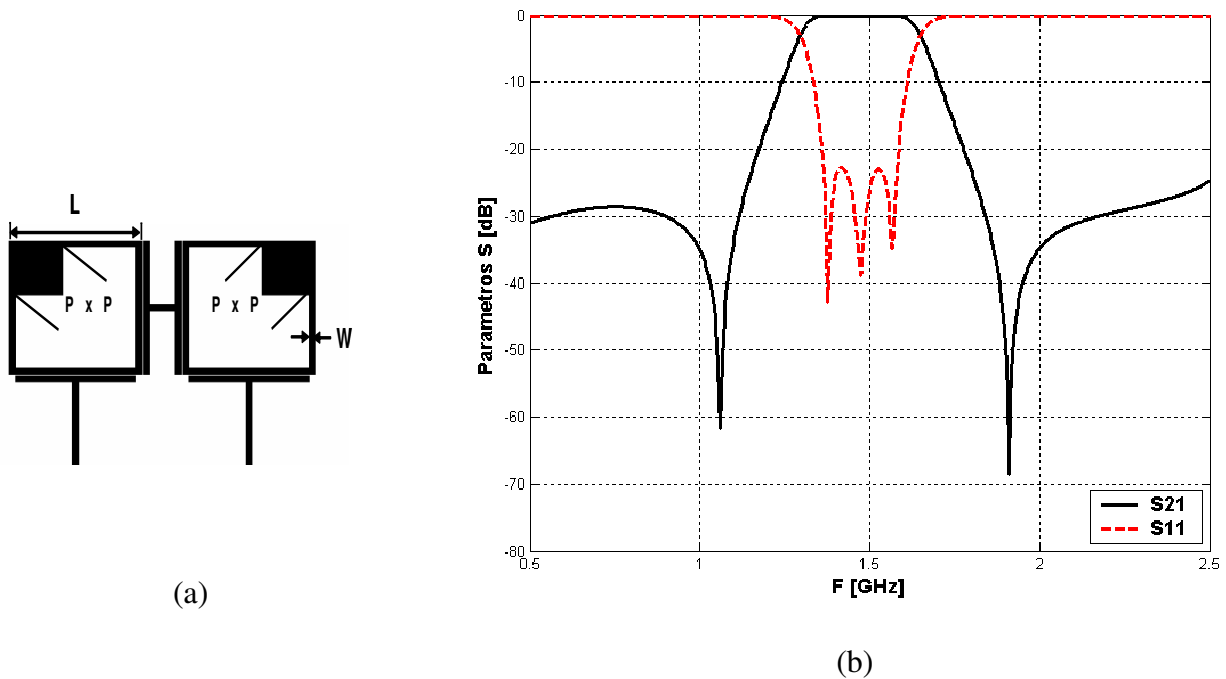
Figura 6.4 Filtro obtido concatenando dois ressoadores dual-mode . (a) Estrutura onde w = 1 mm, L = 20 mm, P = 7,5 mm e gap = 0,2 mm; (b) Parâmetros S.
