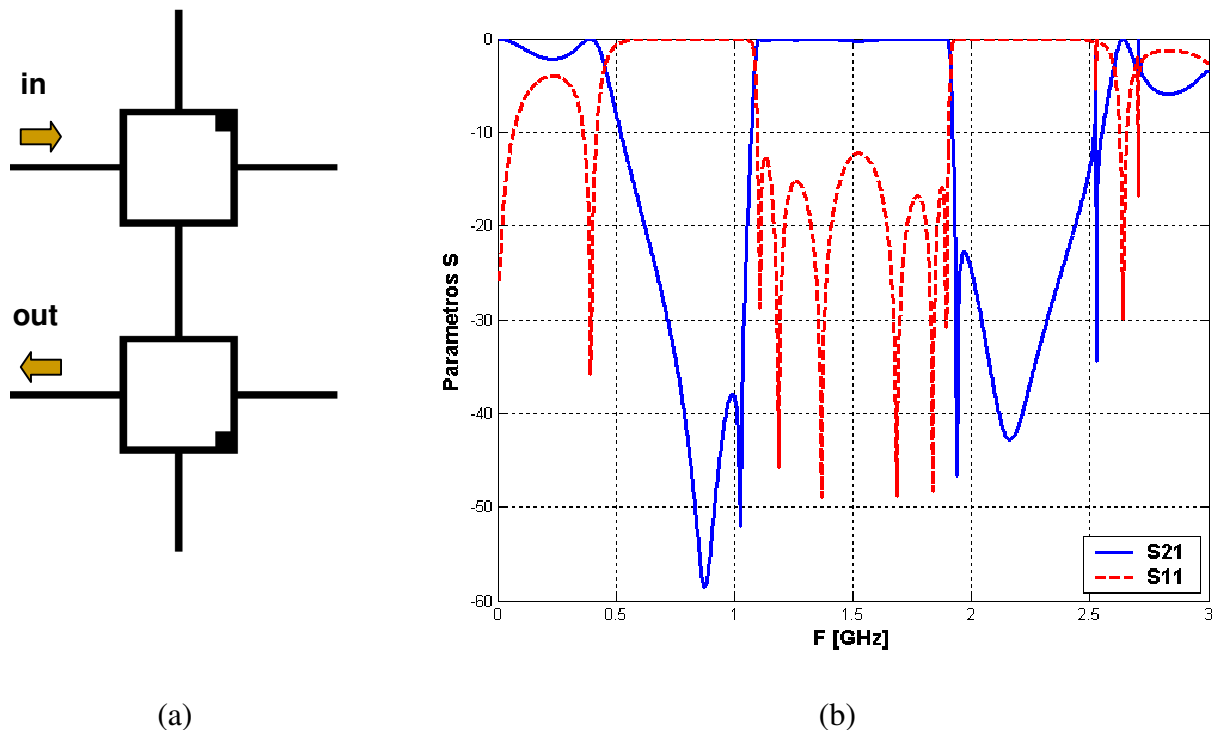
Figura 6.14 Filtro obtido concatenando dois ressoadores equivalentes aos mostrados na Figura 6.12. (a) Dimensões da estrutura: anel de comprimento médio = 80 mm, largura das linhas = 1 mm, stubs = 17,8 mm, P = 2,8 mm. (b) Parâmetros S .
