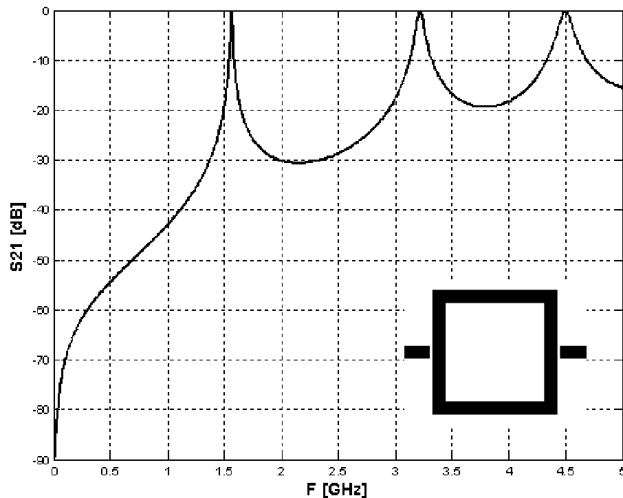
Figura 5.3 |S_{21}| [dB] vs F [GHz] para um ressoador quadrado de comprimento 72 mm alimentado por linhas colineares, gap de 0,2 mm, \epsilon_r = 10,8 e h = 1,27 mm
