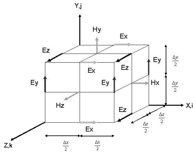
Figura A.2 Célula de Yee
