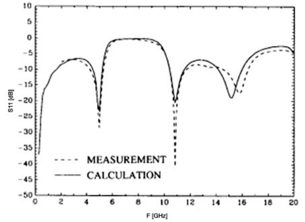
Figura 2.12 Resultados obtidos para o parâmetro S_{11} (a) na simulação do software e (b) extraídos da literatura [6].
