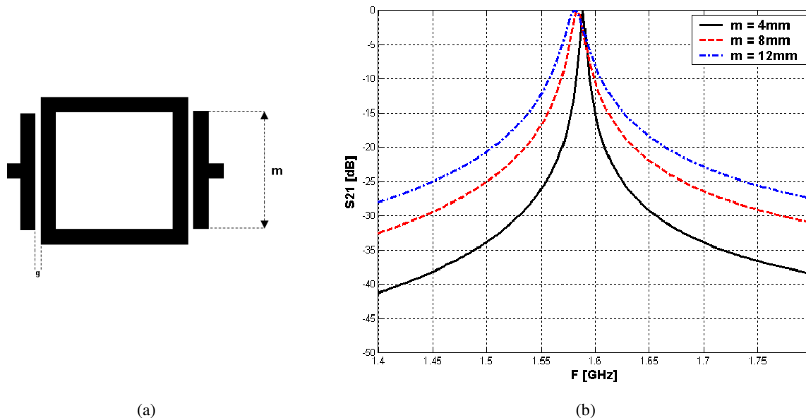
Figura 4.10 Simulações variando-se a área de acoplamento para g = 0,8 mm. (a) Estrutura. (b) Parâmetro S_{21} em função da frequência nas proximidades do modo fundamental do ressoador.
