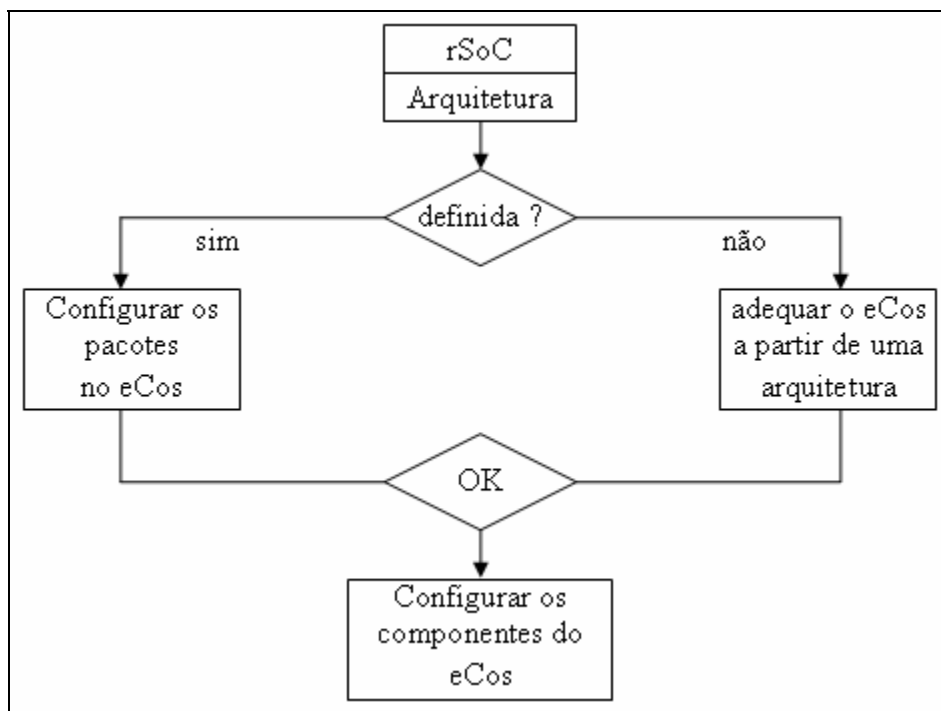
Figura 3.9: Projeto do rSoC com o eCos
