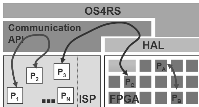
Figura 2.2: Comunicação entre tarefas no RTOS [8]
