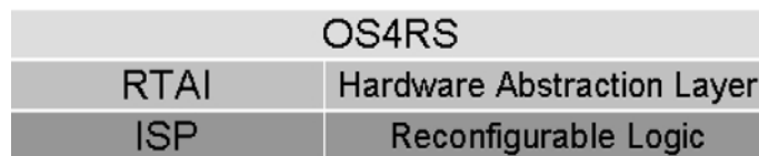
Figura 2.1: RTOS com a camada de abstração de hardware [8]
