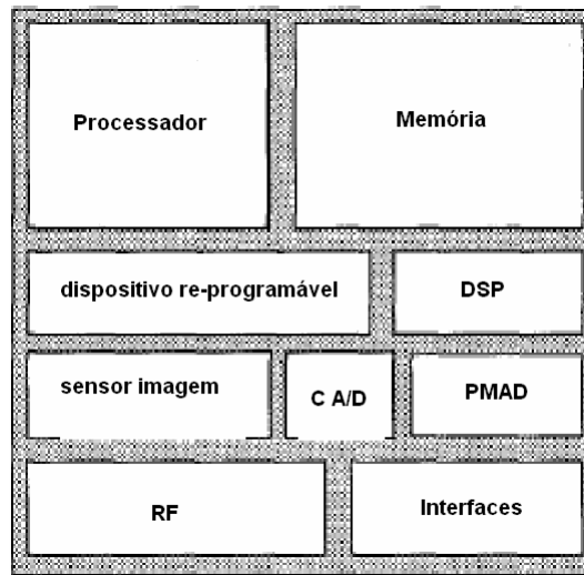
Figura 2.7: Blocos do rSoC
