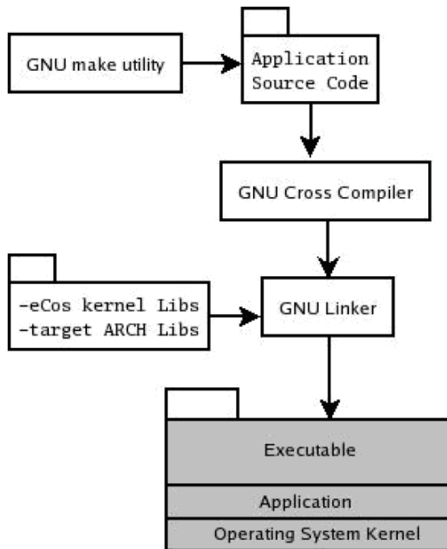
Figura 3.4: Fluxo do processo de desenvolvimento do eCos [49]
