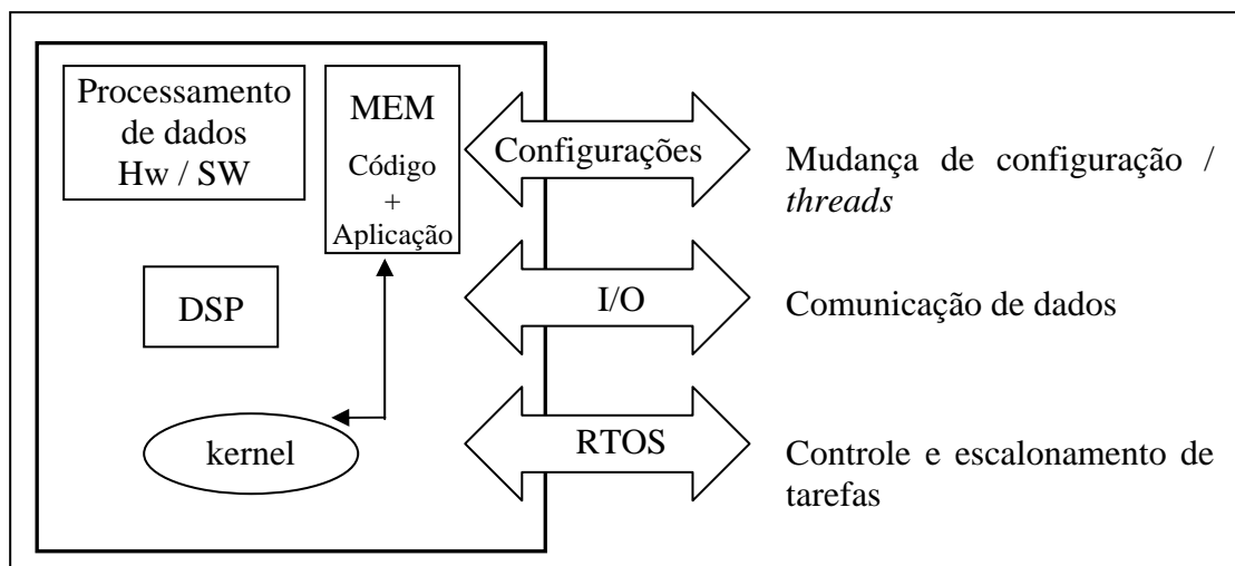
Figura 3.8: Projeto do rSoC com o eCos
