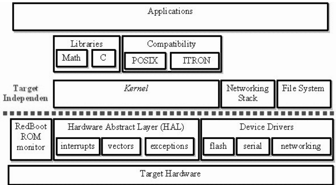
Figura 2.6: Arquitetura do eCos [32]
