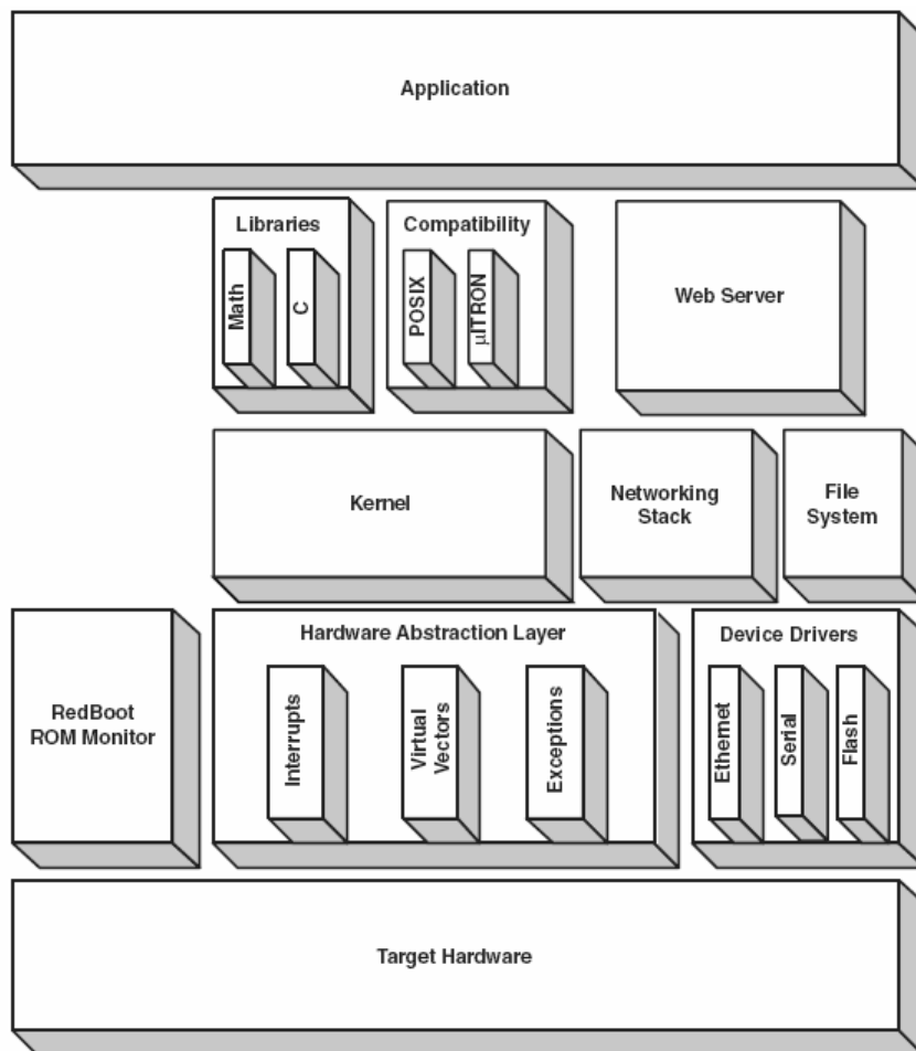
Figura 2.3: Arquitetura de software em camadas do eCos [32]
