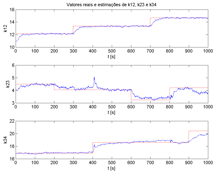
Figura 7.15: Valores reais e estimados de k_{12} , k_{23} e k_{34} - LEA controle MPC
