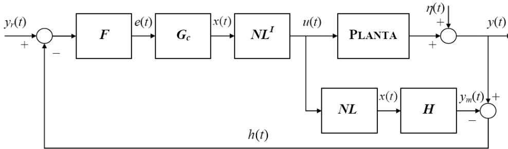
Figura 2.2: Estrutura do Controlador de Fruzzetti
