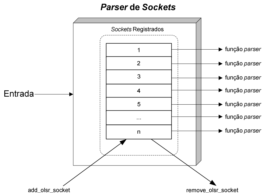
Figura 3.2 – Parser de Sockets
