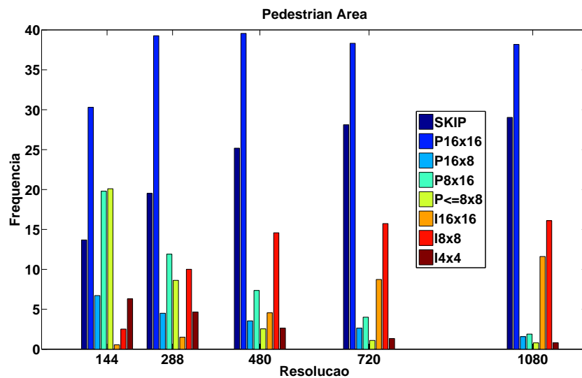
Figura 3.1: Frequência de ocorrência de modos de predição × resolução para a seqüência Pedestrian Area.
