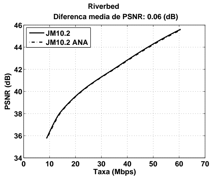
Figura 5.12: Curva de taxa \times distorção para a seqüência Riverbed: JM10.2 \times JM10.2-ANA.
