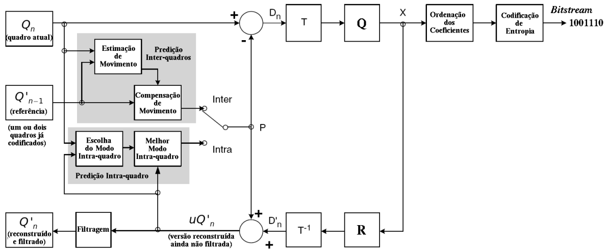
Figura 4.1: Codificador de Vídeo DPCM Híbrido. Adaptado de [2].
