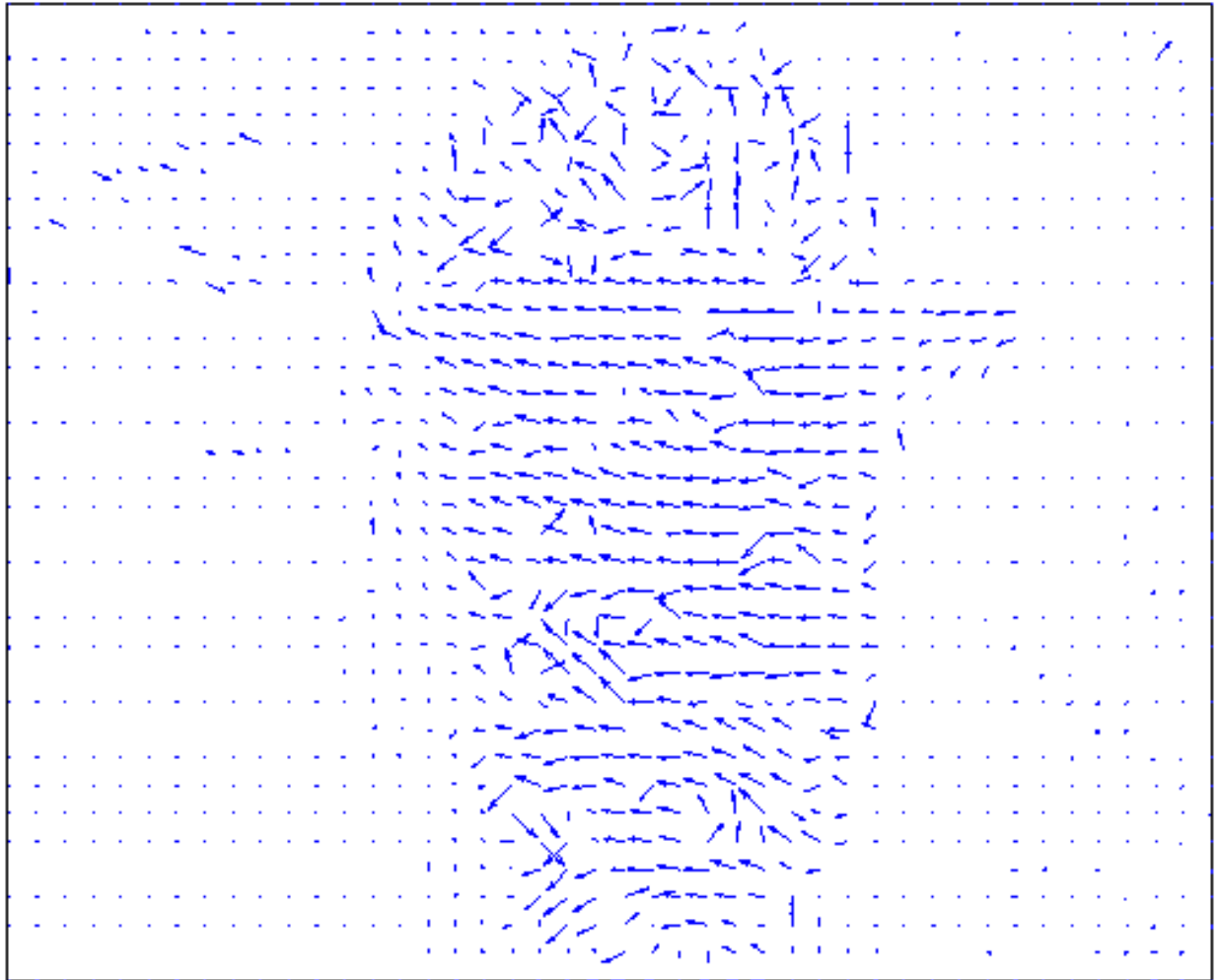
Figura 2.3: Fluxo óptico composto por vetores de movimento para cada bloco de 8 \times 8 pixels da imagem da Figura 2.2(b) com relação à Figura 2.2(a).
