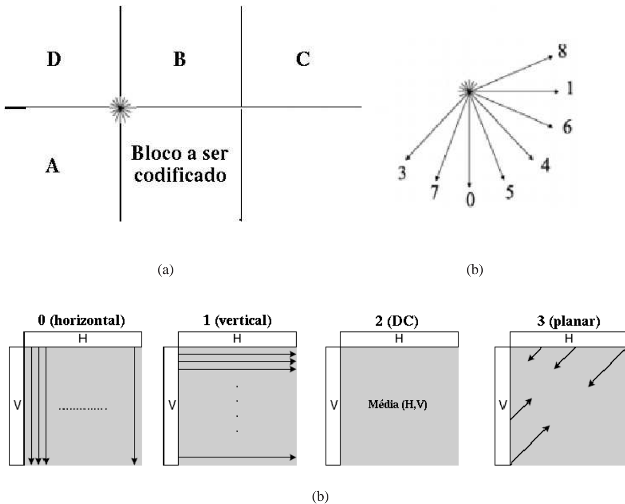
Figura 2.8: Janela causal (a) para codificação e modos de predição para codificação Intra-quadro com suas direções de interpolação planar para blocos 4 \times 4 e 8 \times 8 (b) e 16 \times 16 (c). O modo 2, não apresentado em (b), é o DC.
