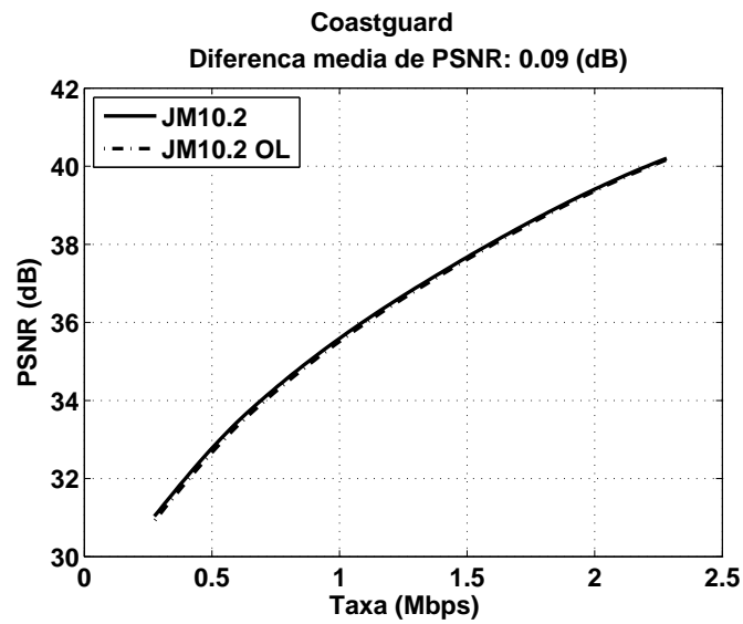
Figura 5.18: Curva de taxa \times distorção para a seqüência Coastguard: JM10.2 \times JM10.2-ANA.
