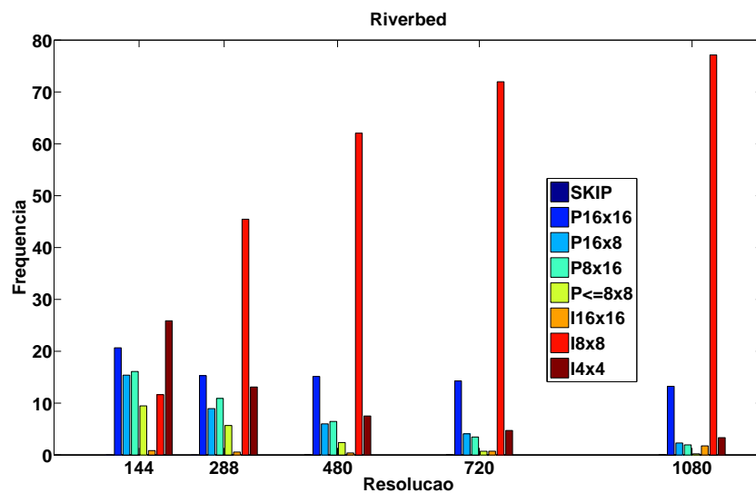
Figura 3.2: Frequência de ocorrência de modos de predição × resolução para a seqüência Riverbed.
