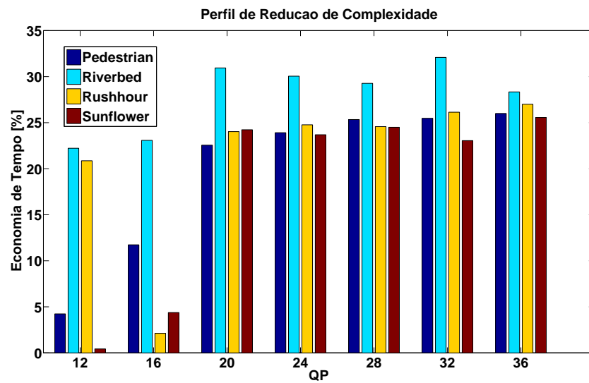
Figura 5.15: Curva do perfil de redução de complexidade (quanto tempo foi economizado) para as quatro seqüências de vídeo analisadas.
