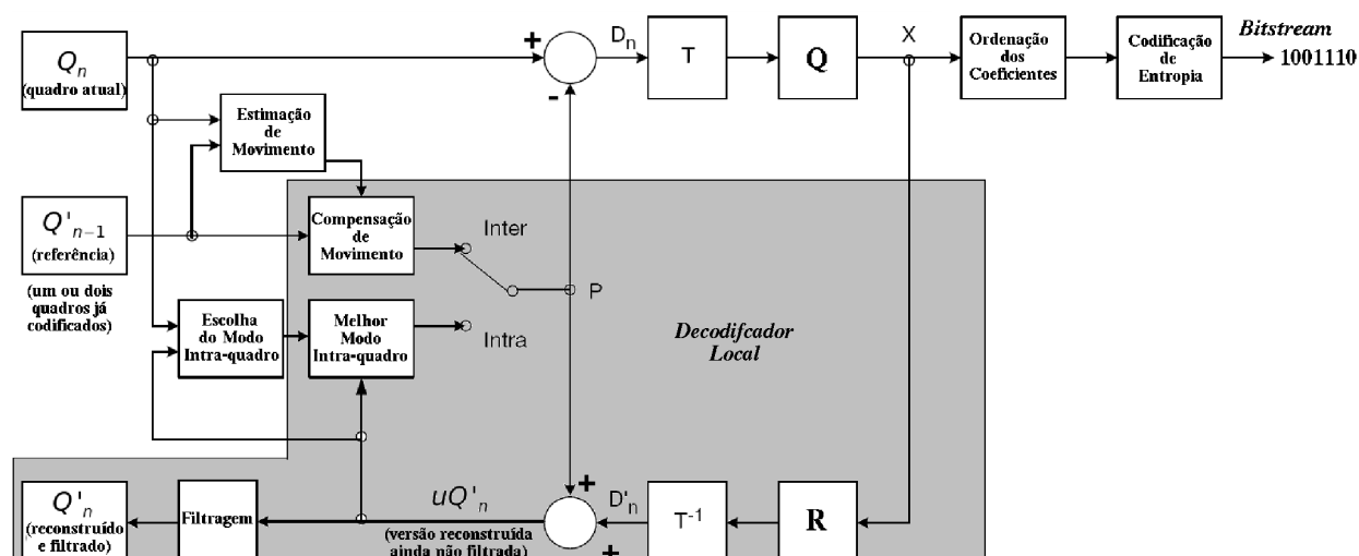
Figura 2.6: Codificador de vídeo DPCM híbrido. Adaptado de [2].
