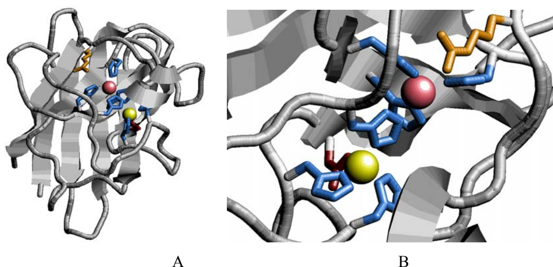
Figura 3. Estrutura molecular da CuZnSOD. A) Estrutura tridimensional da CuZnSOD. B) Detalhe do centro ativo. Desenhados a partir de modelo descrito para CuZnSOD de levedura (Cod. 1SDY do Protein Data Bank ), utilizando o programa RasMol (SAYLE & MILNER-WHITE, 1995). Em azul, os resíduos de histidina; em vermelho o resíduo de aspartato; em laranja, o resíduo de arginina; em amarelo, Zn^{+2} ; em rosa, Cu^{2+} ; em cinza, \beta -fitas e \alpha -hélices.
