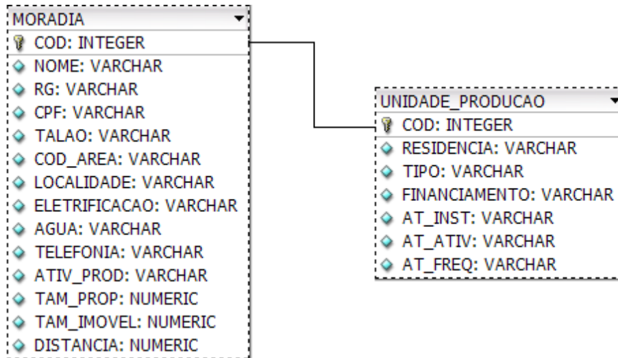
Figura 3 – Relacionamento entre tabelas do tipo 1:1
