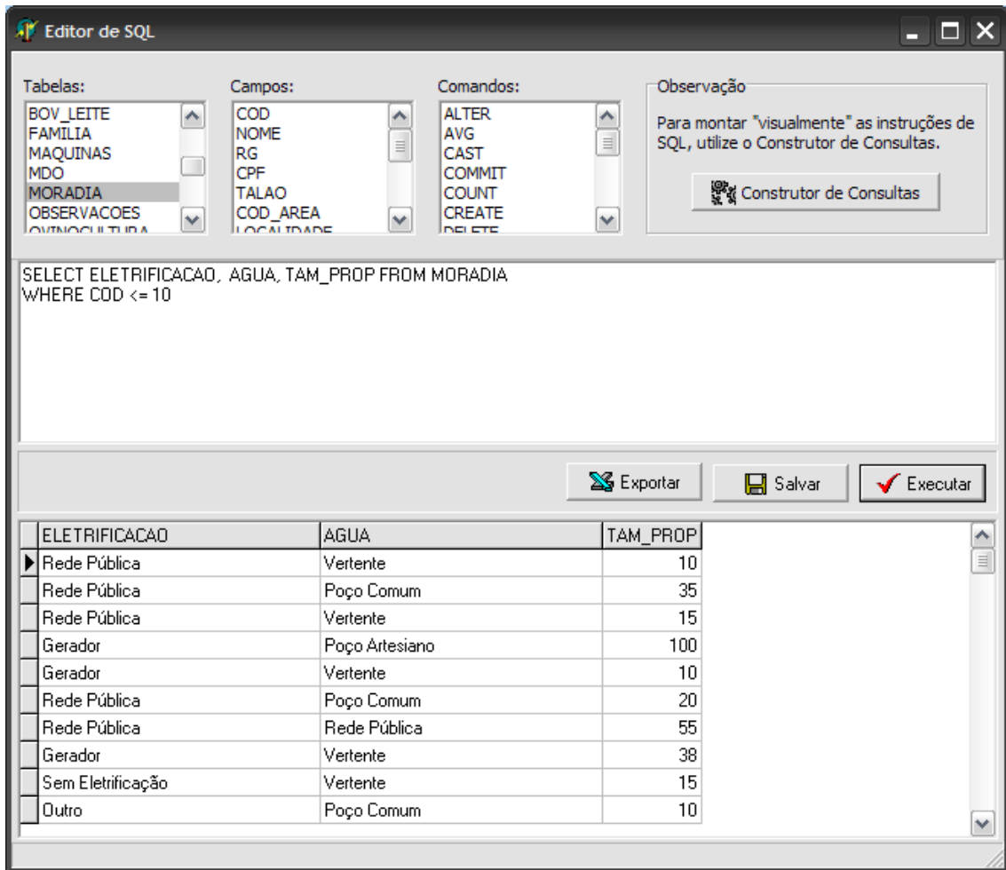
Figura 22 – Tela do Editor de SQL
