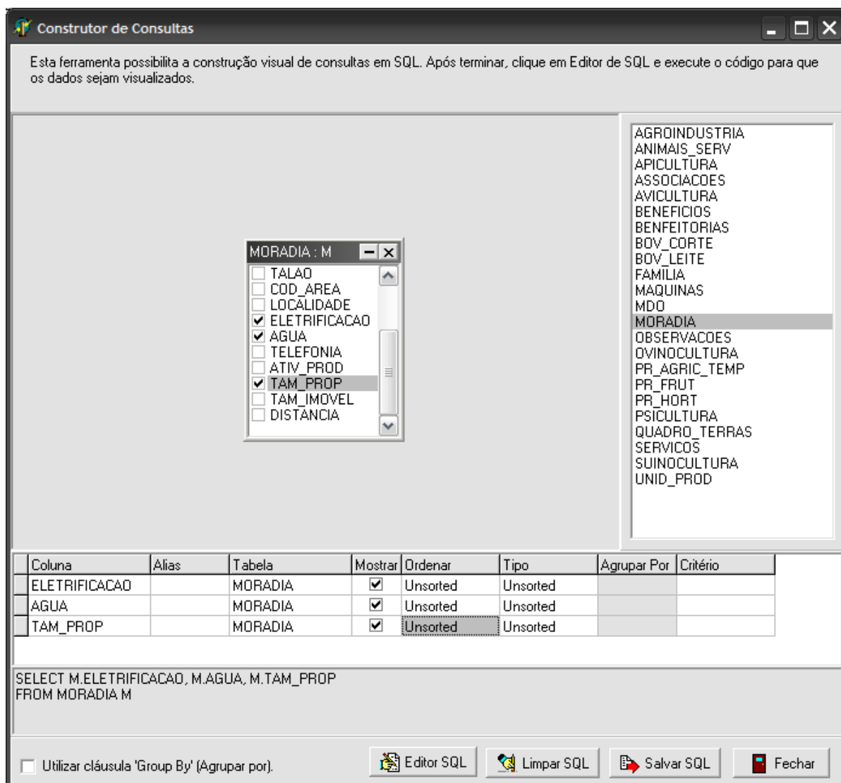
Figura 23 – Tela do Construtor de Consultas
