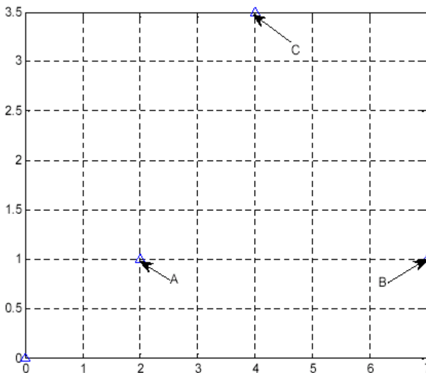
Figura 1 – Dispersão entre três indivíduos mensurados com relação a duas variáveis quantitativas contínuas.
