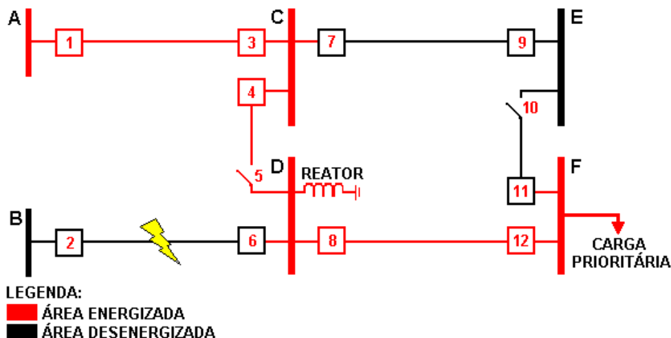
Figura 2.6 – Recomposição seqüência do sistema até a subestação F
