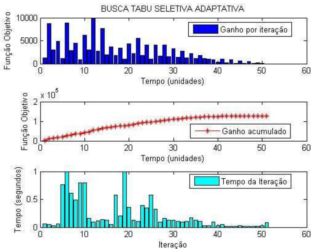
Figura 5.3 - Resultado gráfico da recomposição para o caso 01 aplicando a BTSA
