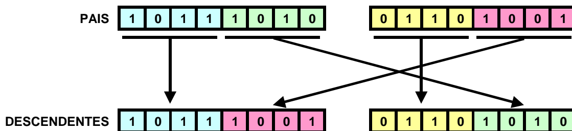
Figura 3.8 - Exemplo de recombinação com 01 ponto de cruzamento
