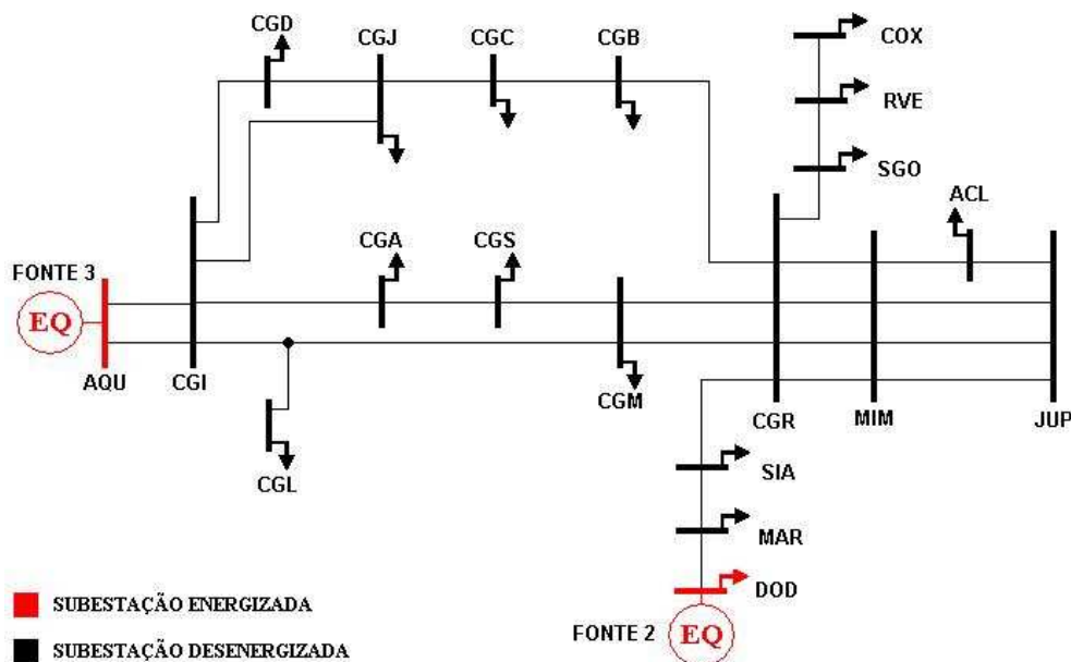
Figura 5.8 – Condição inicial do caso 02
