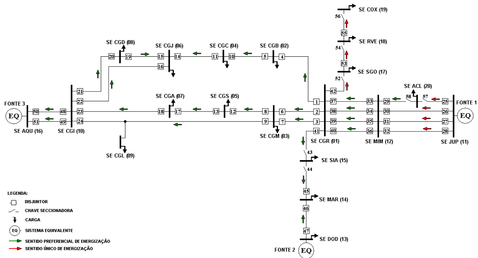
Figura A.1 - Parte do sistema elétrico de sub-transmissão do Estado de Mato Grosso do Sul
