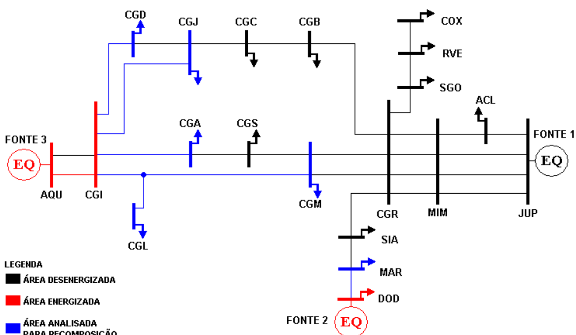
Figura 5.12 – Exemplo da ramificação da árvore de soluções em uma iteração
