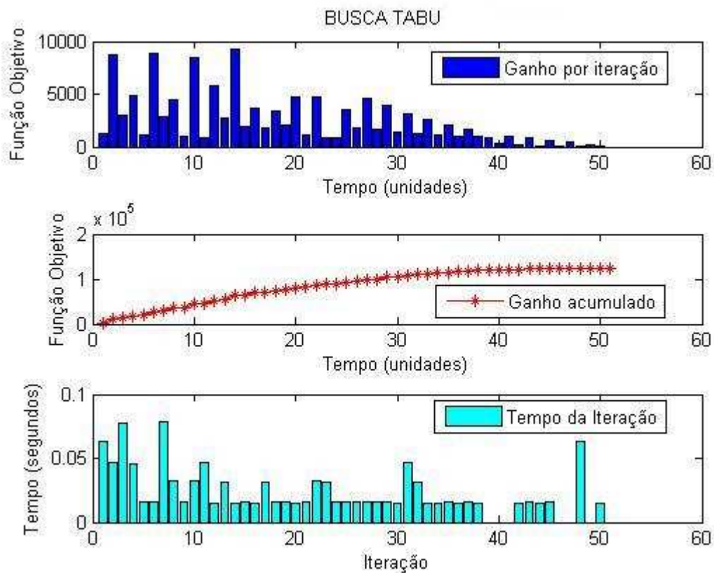
Figura 5.5 - Resultado gráfico da recomposição para o caso 01 aplicando a BT
