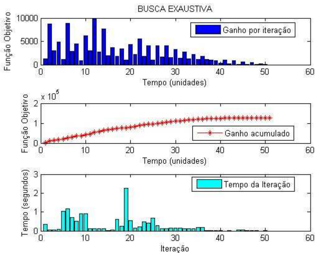
Figura 5.6 - Resultado gráfico da recomposição para o caso 01 aplicando a BE
