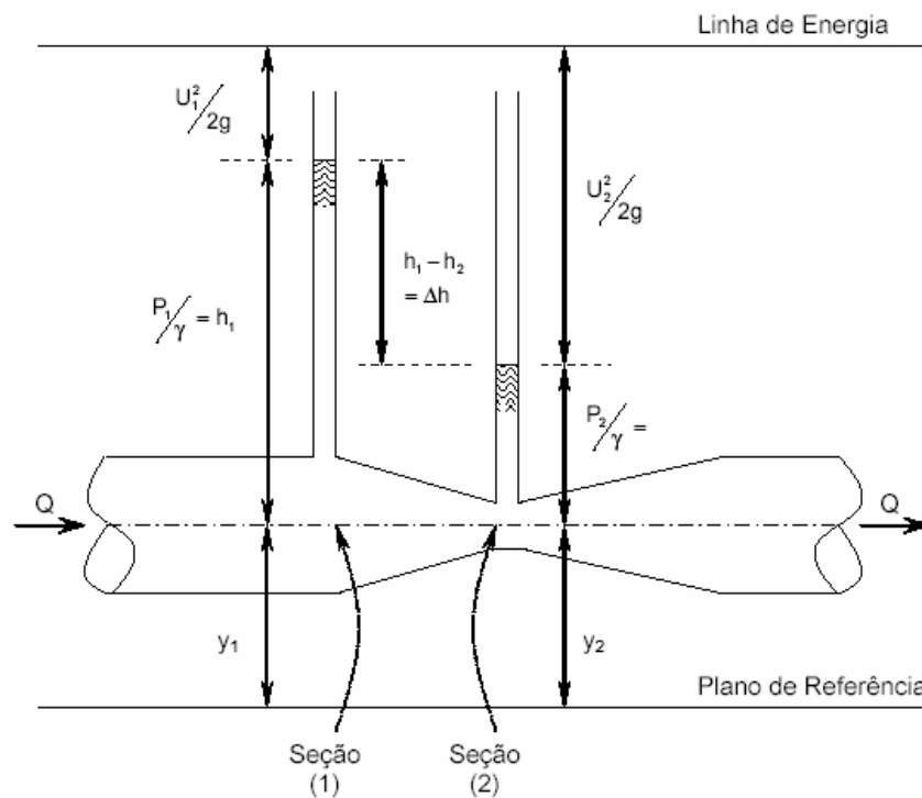
Figura 19. Tubo Venturi
