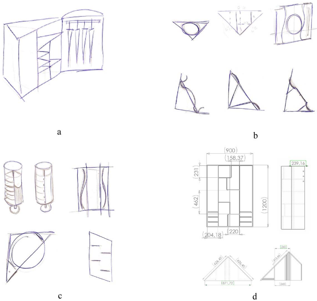
Figura 49. a), b) e c) Desenho e esboços na criação do chapeleiro “no Hat”; d) Desenho técnico do móvel.(Alunas: Caroline Bonfim, Samara Pereira e Vanessa Sueishi, 2006).
