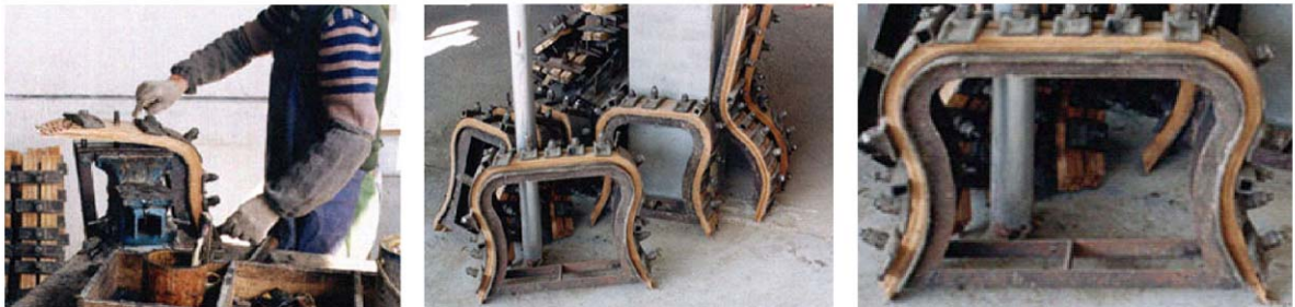
Figura 23. Moldes de metal (Fonte: INBAR, 2001).
