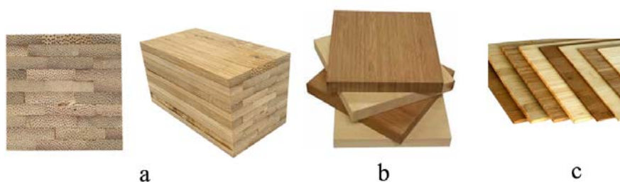
Figura 20. a) Bambu laminado colado (PEREIRA, 1997); b) BLC, com duas camadas verticais. (Fonte: http://.zenbamboo.com , 2006); c) BLC com uma camada. (Fonte: http://www.cbamboo.com 2006).
