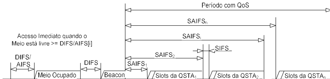
Figura 4.11 – SAIFS durante um período com QoS de um SuperFrame.
