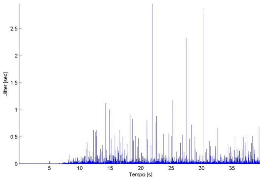
Figura 5.22 - Jitter do EDCA.
