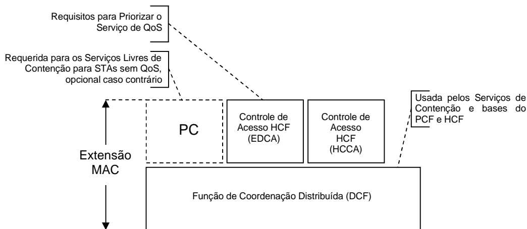
Figura 3.1 – Arquitetura MAC.
