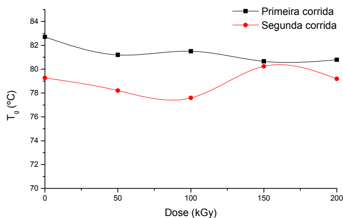
FIG. 4.16 - Variação da temperatura de transição vítrea ( T_g ) do PETG, antes e após irradiação gama (1ª e à 2ª varredura)
