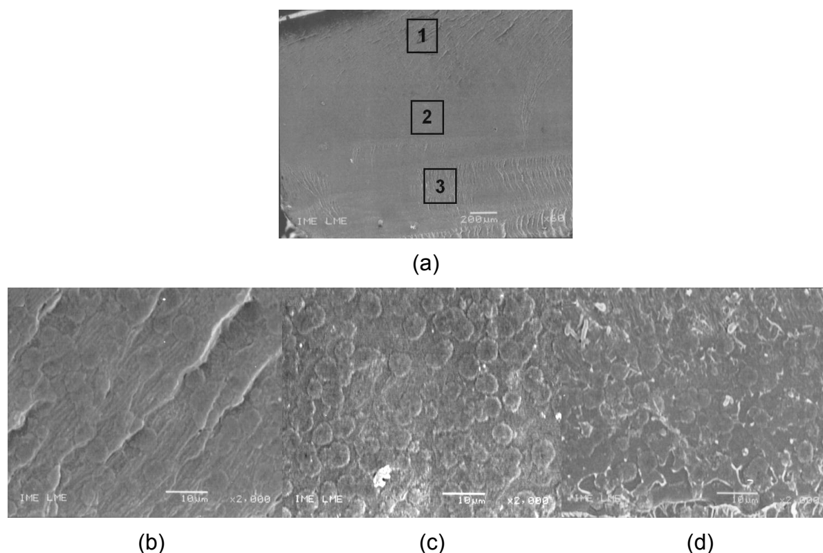
FIG 4.35 - Microfotografias, por SEM, das superfícies de fratura da amostra de PETG recozida a 140°C após ataque químico com o reativo permangânico de composição A: (a) vista geral; (b) detalhe de (a) na região 1; (c) idem na região 2; (d) idem na região 3
