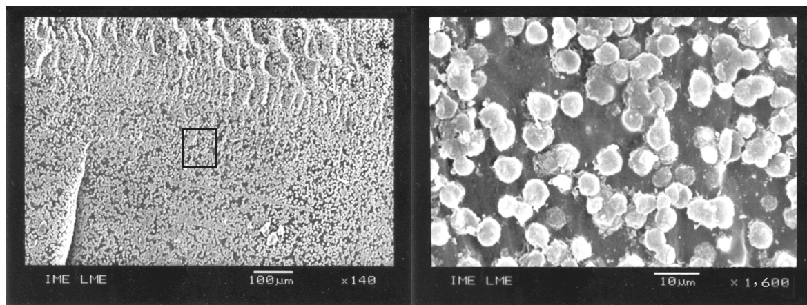
FIG 4.36 - Microfotografias, por SEM, das superfícies de fratura da amostra de PETG recozida a 140°C após ataque químico com o reativo permangânico de composição B: (a) vista geral; (b) detalhe da região assinalada em (a)
