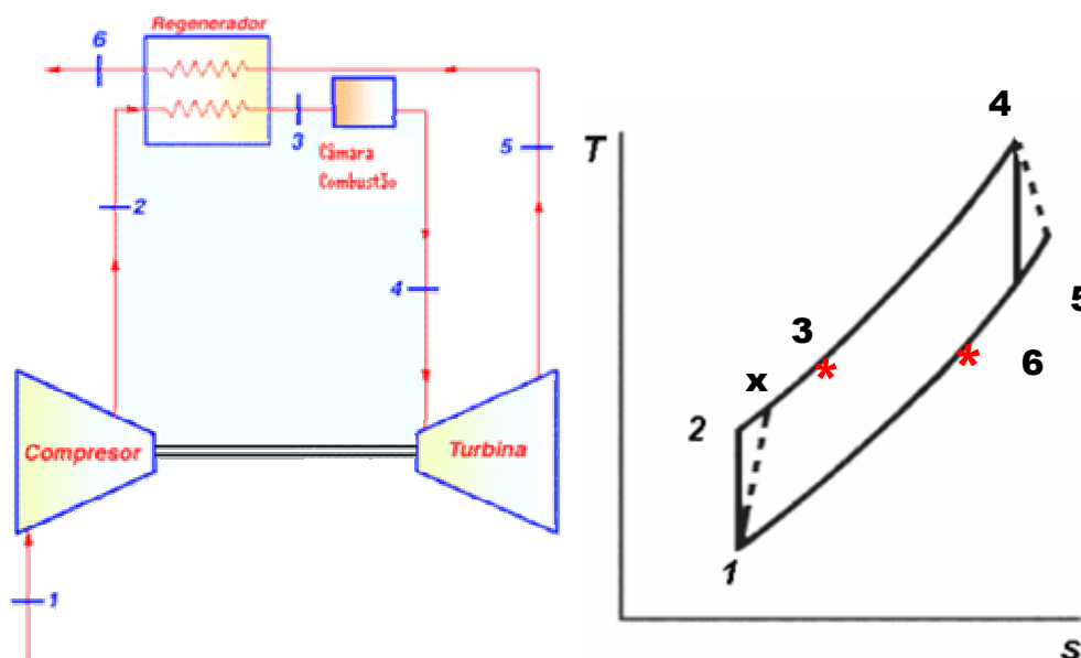
Figura 3.3. Ciclo regenerativo
