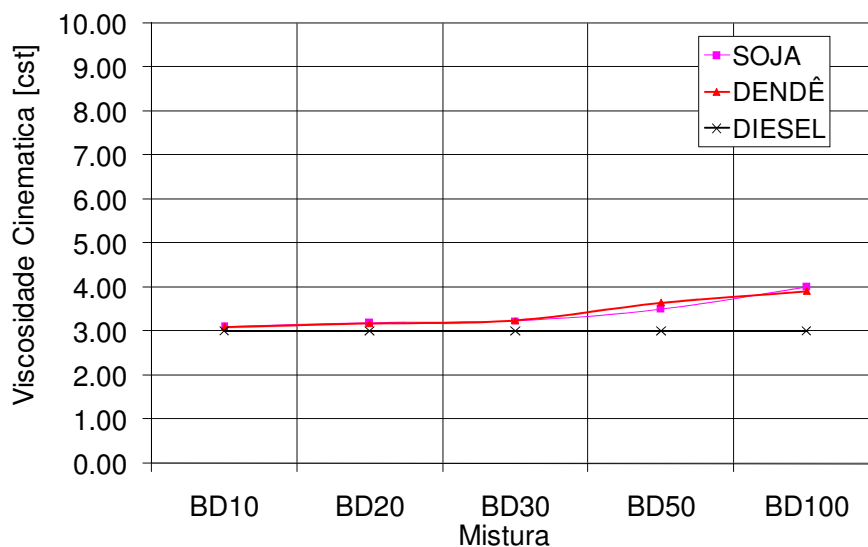
Figura 4.2. Viscosidade cinemática das misturas Biodiesel/Diesel a 40 °C.
