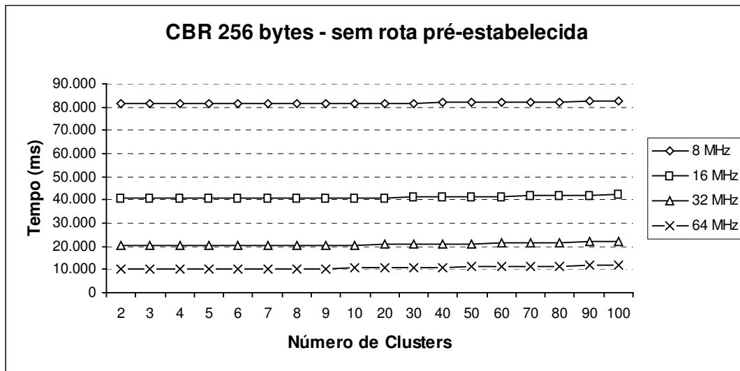
Gráfico 5: Tempo máximo para troca de uma mensagem CBR de 256 bytes sem rota pré-estabelecida
