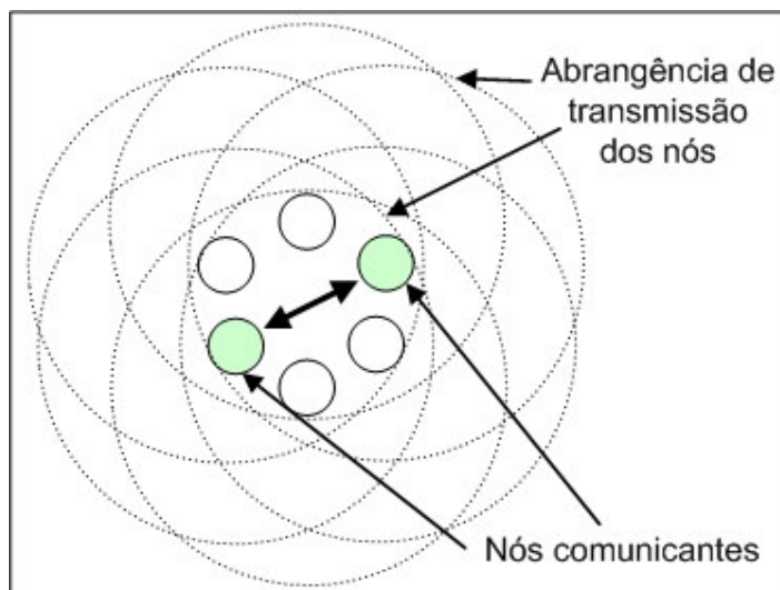
Figura 8: Comunicação direta numa rede ad hoc
