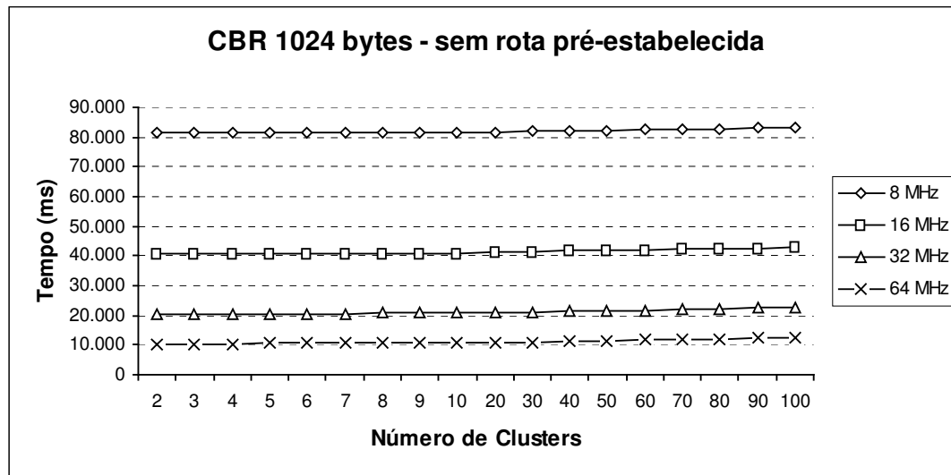
Gráfico 9: Tempo máximo para troca de uma mensagem CBR de 1024 bytes sem rota pré-estabelecida
