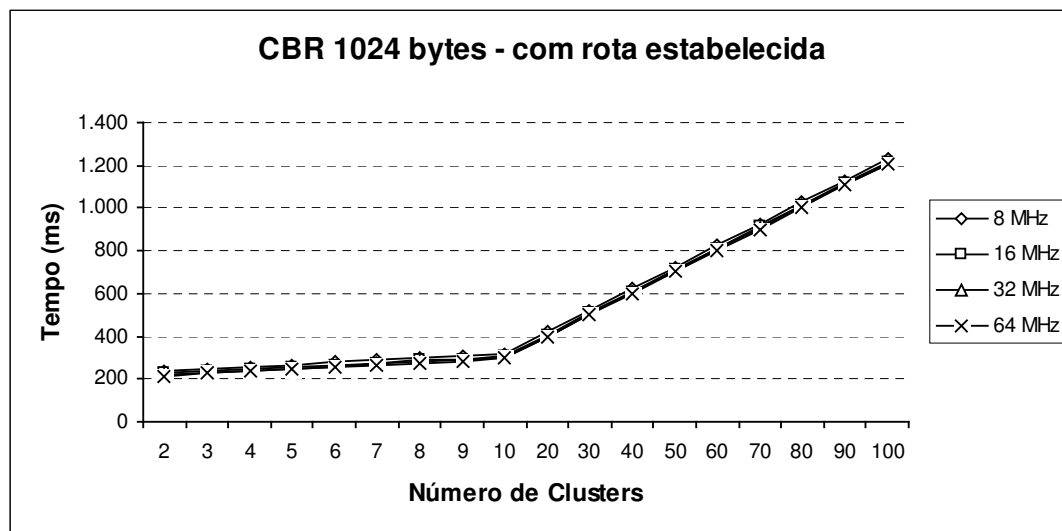
Gráfico 10: Tempo máximo para troca de uma mensagem CBR de 1024 bytes com rota estabelecida
