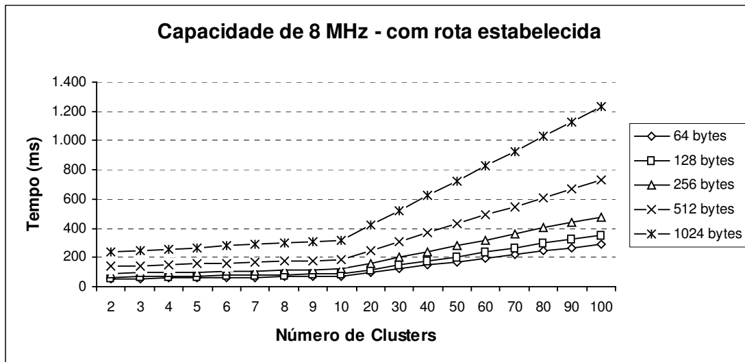
Gráfico 12: Envio de mensagem utilizando cluster heads de 8Mhz com rota pré-estabelecida
