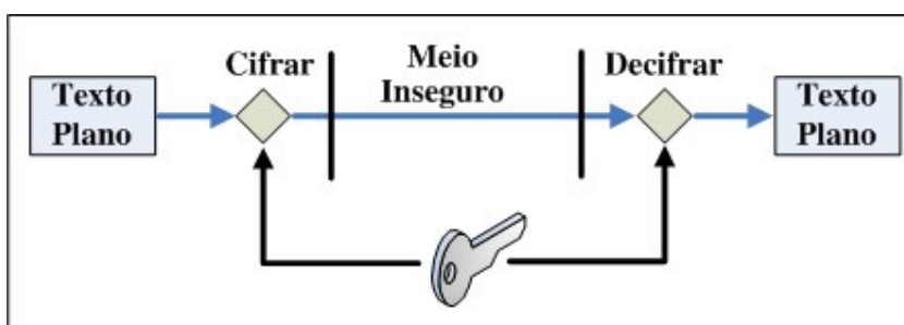
Figura 2: Criptografia com chave simétrica
