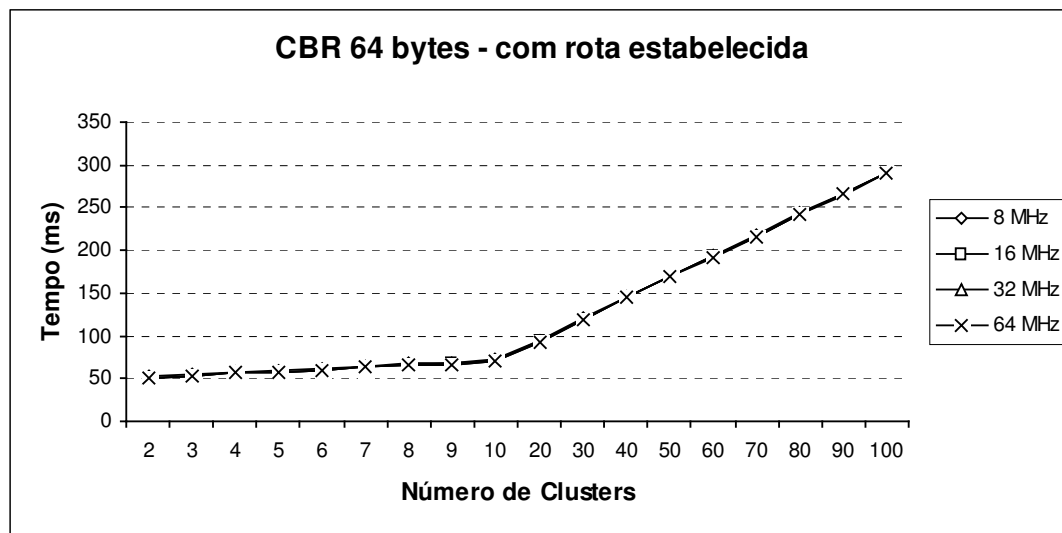
Gráfico 2: Tempo máximo para troca de uma mensagem CBR de 64 bytes com rota estabelecida
