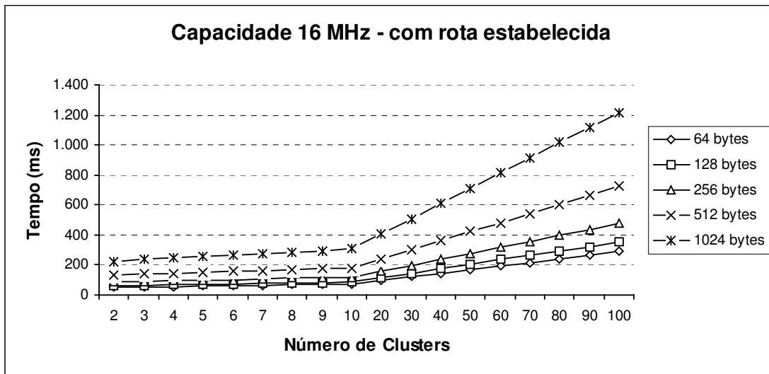
Gráfico 14 : Envio de mensagem utilizando cluster heads de 16 Mhz com rota pré-estabelecida
