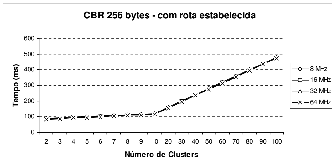
Gráfico 6: Tempo máximo para troca de uma mensagem CBR de 256 bytes com rota estabelecida
