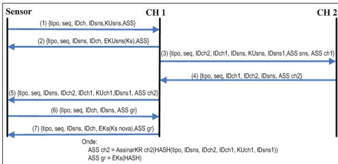
Figura 17: O protocolo de distribuição de chaves
