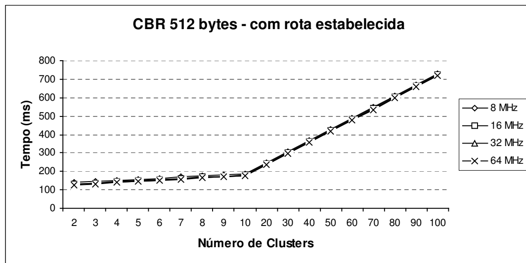
Gráfico 8: Tempo máximo para troca de uma mensagem CBR de 512 bytes com rota estabelecida
