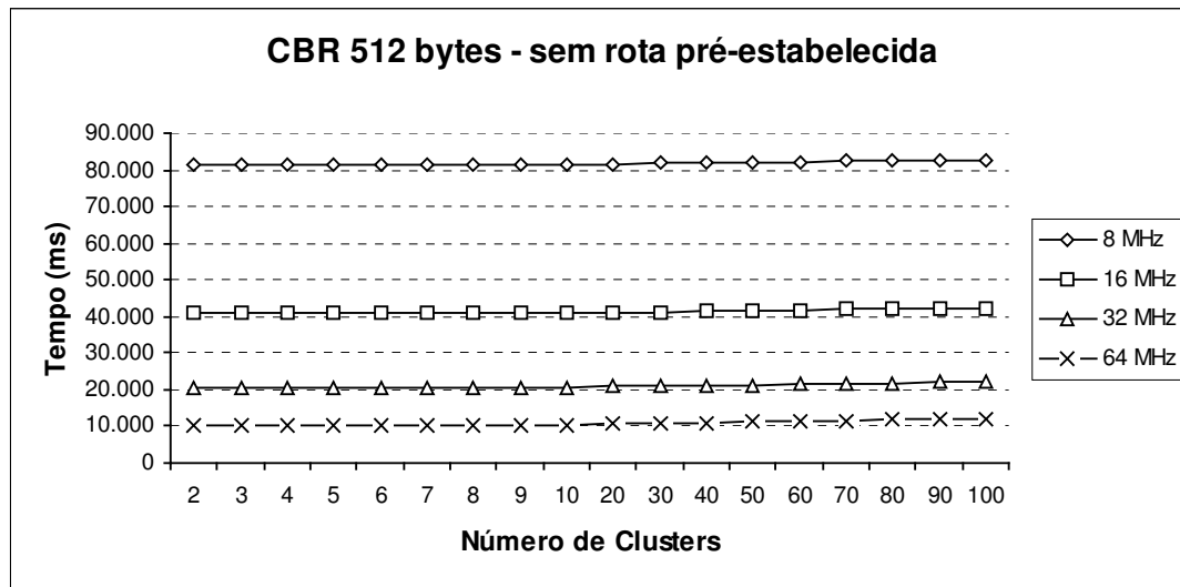
Gráfico 7: Tempo máximo para troca de uma mensagem CBR de 512 bytes sem rota pré-estabelecida
