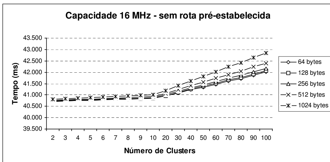
Gráfico 13: Envio de mensagem utilizando cluster heads de 16 Mhz sem rota pré-estabelecida
