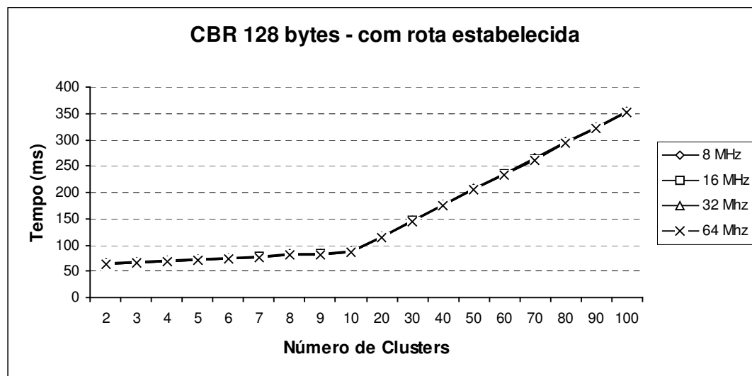
Gráfico 4: Tempo máximo para troca de uma mensagem CBR de 128 bytes com rota estabelecida
