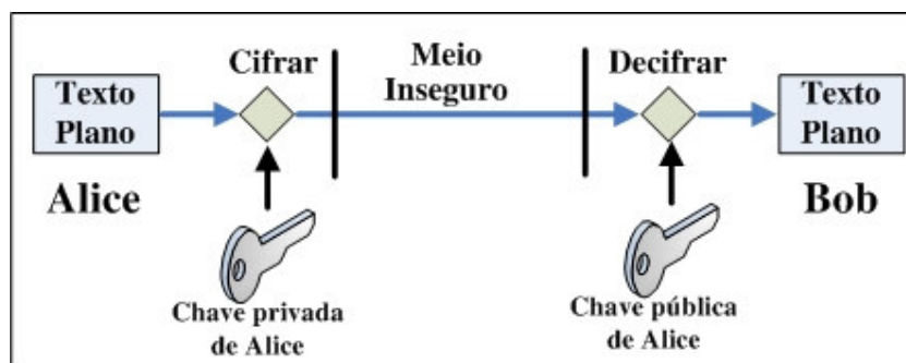
Figura 4: Uso de criptografia assimétrica para garantir autenticidade
