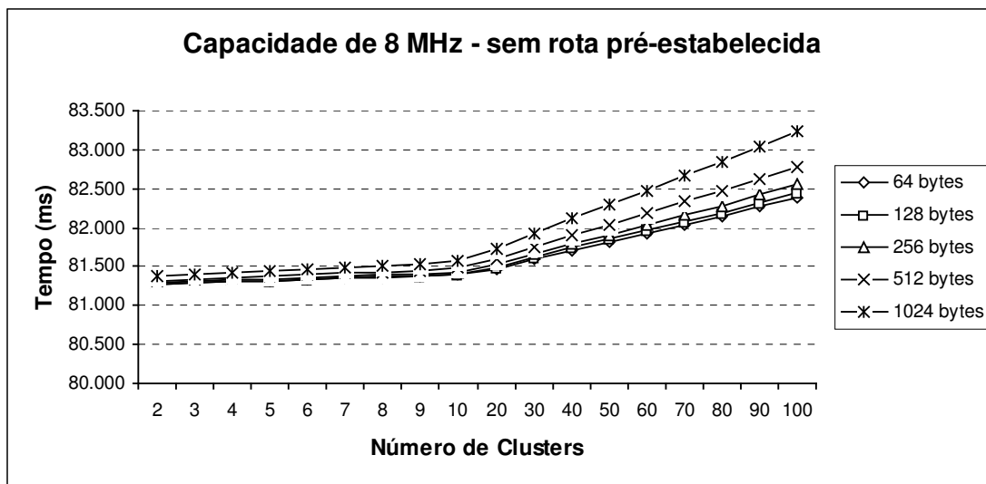
Gráfico 11: Envio de mensagem utilizando cluster heads de 8Mhz sem rota pré-estabelecida
