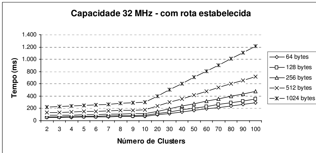
Gráfico 16: Envio de mensagem utilizando cluster heads de 32 Mhz com rota pré-estabelecida
