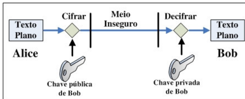
Figura 3: Uso de criptografia assimétrica para garantir confidencialidade
