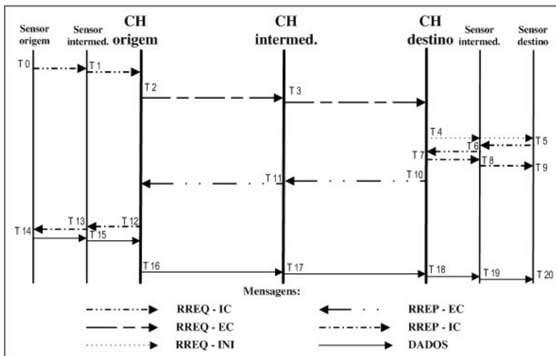
Figura 18: seqüência de mensagens para estabelecimento de rota e envio de dados
