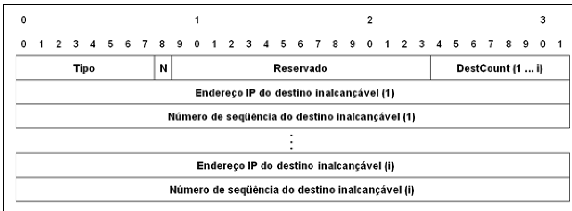
Figura 12: O formato da mensagem de erro de rota RERR do AODV
