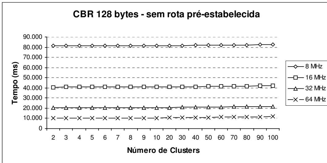
Gráfico 3: Tempo máximo para troca de uma mensagem CBR de 128 bytes sem rota pré-estabelecida
