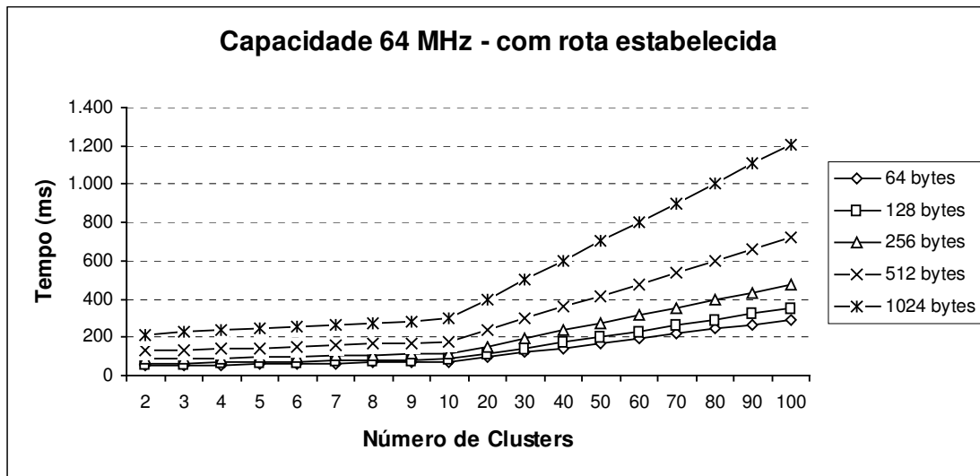
Gráfico 18: Envio de mensagem utilizando cluster heads de 64 Mhz com rota pré-estabelecida
