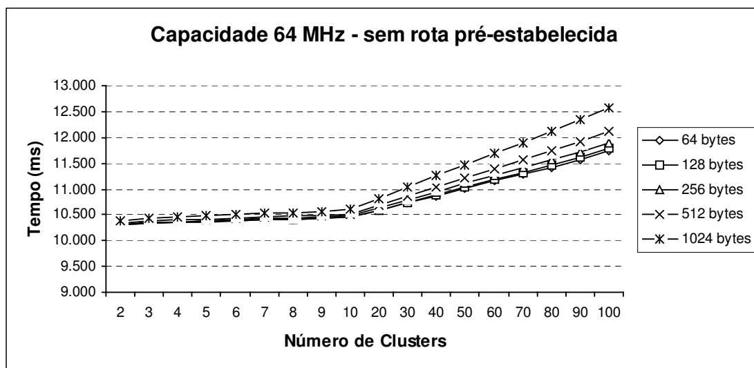
Gráfico 17: Envio de mensagem utilizando cluster heads de 64 Mhz sem rota pré-estabelecida
