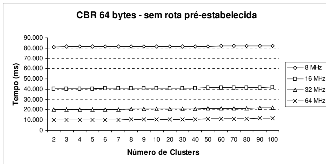
Gráfico 1: Tempo máximo para troca de uma mensagem CBR de 64 bytes sem rota pré-estabelecida
