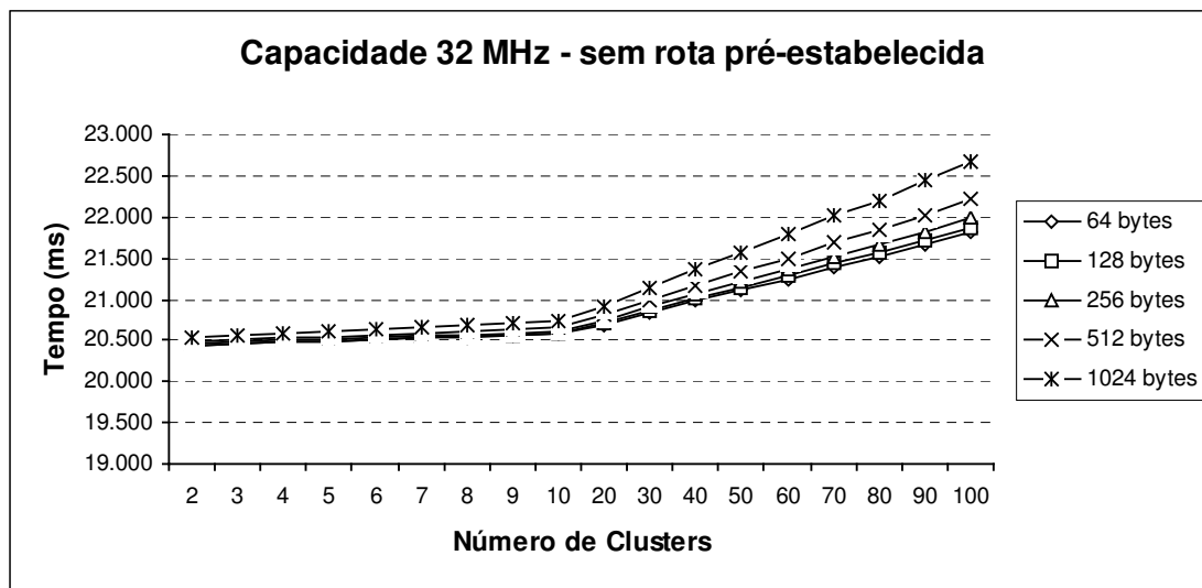
Gráfico 15: Envio de mensagem utilizando cluster heads de 32 Mhz sem rota pré-estabelecida
