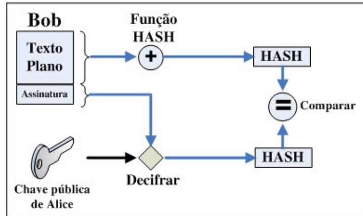
Figura 7: Verificação de uma assinatura digital
