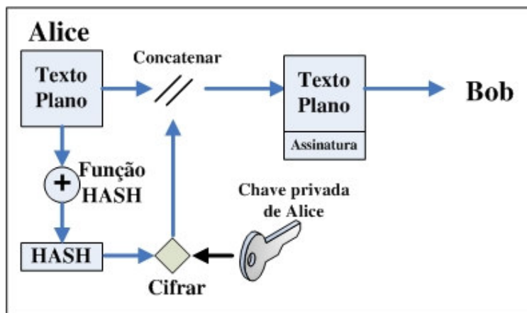
Figura 6: Criação de uma assinatura digital
