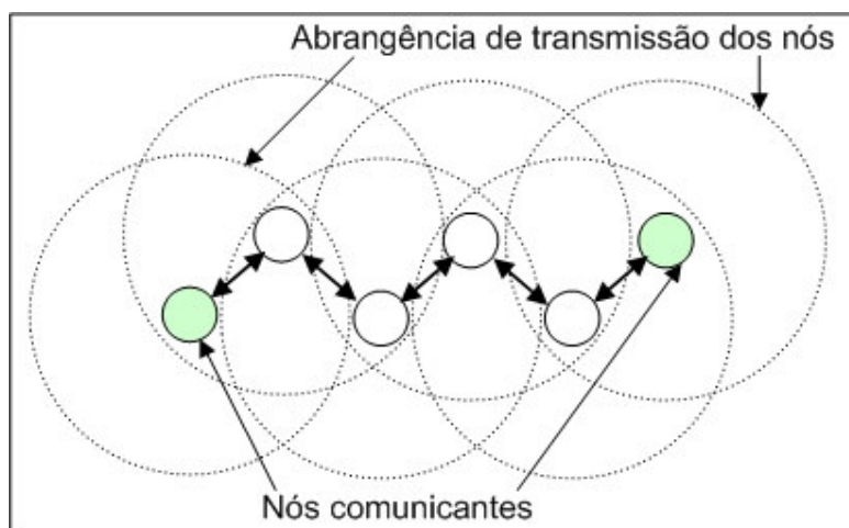
Figura 9: Comunicação de múltiplos saltos numa rede ad hoc
