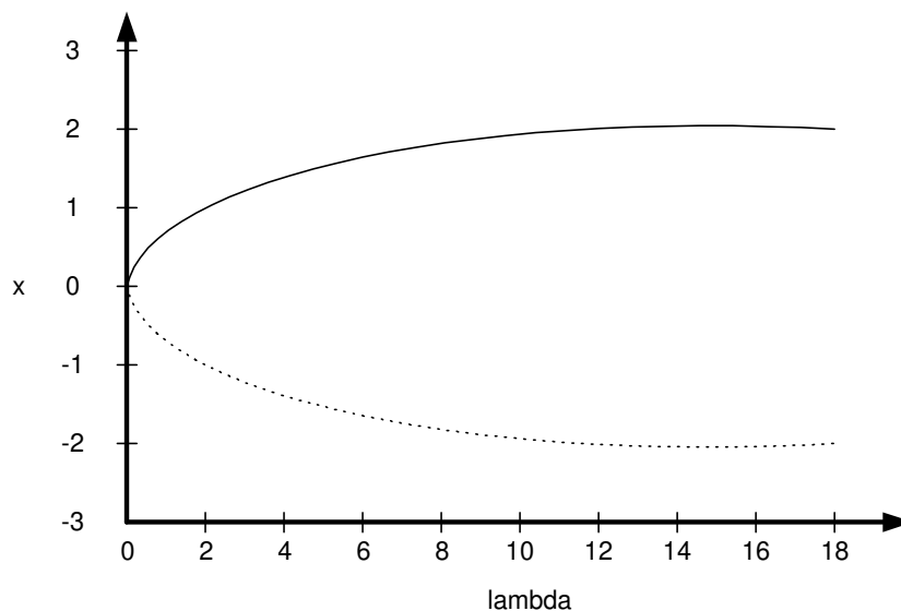
Figura 3.1: Diagrama de bifurcação de uma Sela-nó
