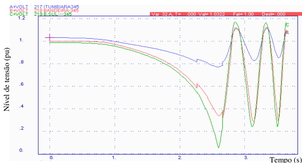
Figura 2.4 : Centro Elétrico em Itumbiara, Bandeirantes e Brasília Sul - 345 kV
