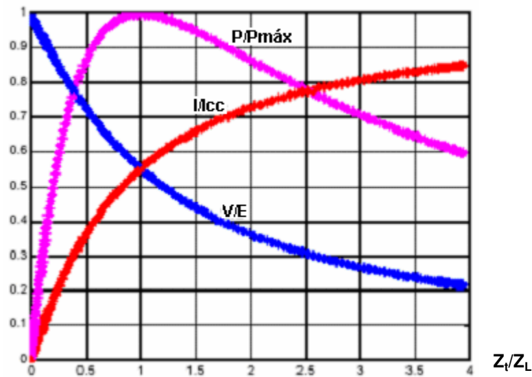
Figura 3.8: Evolução de P/P_{máx} , V/E e I/I_{CC} em função da variação de Z_t/Z_L
