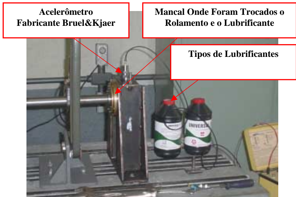
Figura 5.4 – Acelerômetro e mancal onde foram trocados o rolamento e o lubrificante
