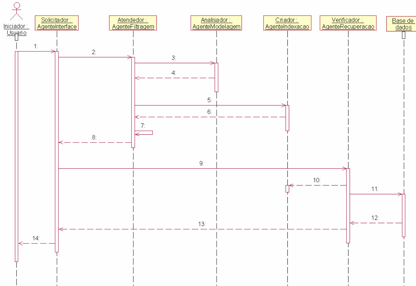
Figura 25 - Diagrama de Interação da Fase de Identificação de Papéis. Cenário: Filtragem Baseada em Conteúdo.
