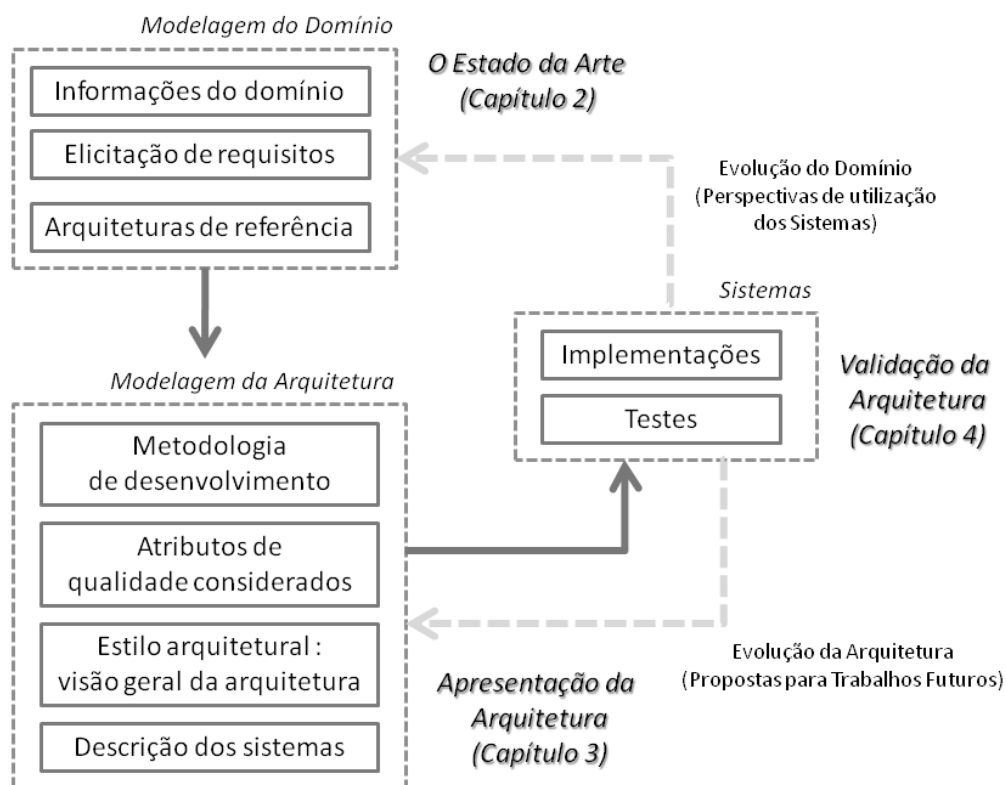
Figura 1.4 – Metodologia utilizada para o desenvolvimento do trabalho.
