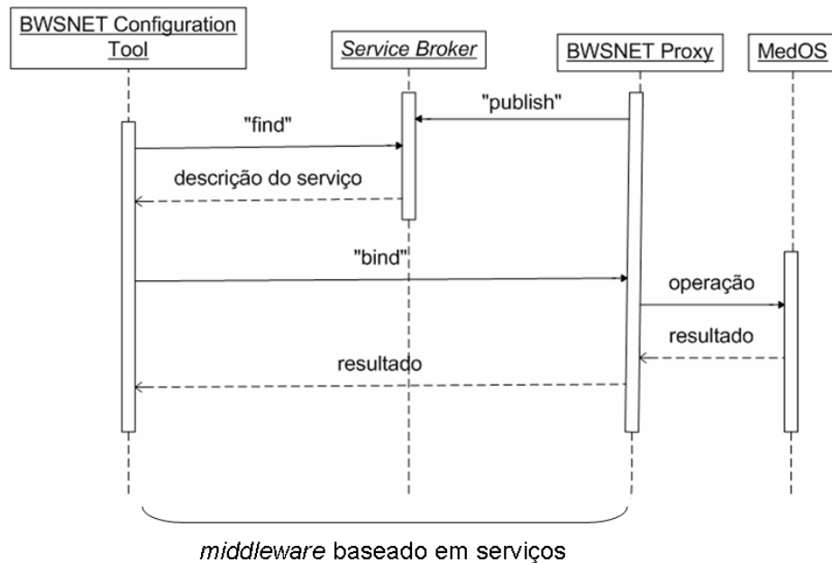
Figura 3.9 – Operações da SOAB segundo padrão SOA.
