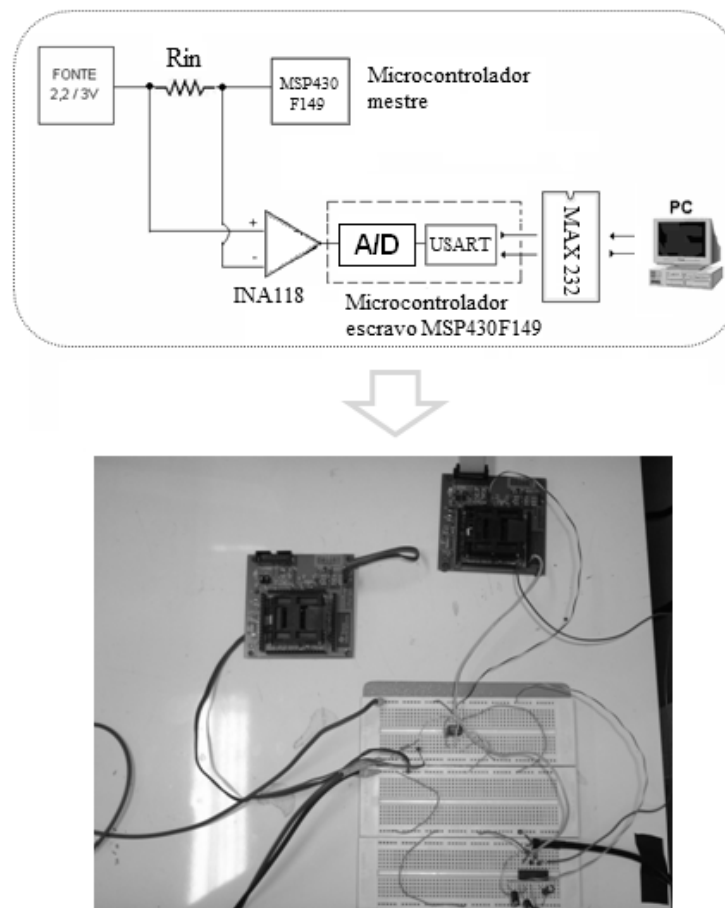
Figura 4.36 – Circuito de testes e protótipo utilizado para avaliar PowerManager .
