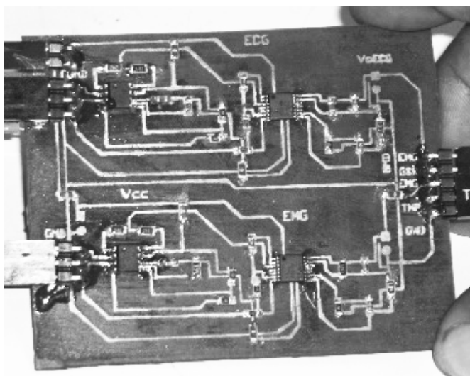
Figura 4.29 – Protótipo em placa de circuito impresso (GUTIÉRREZ et al. , 2006).
