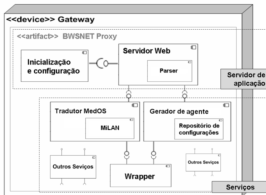
Figura 3.10 – Principais componentes do BWSNET Proxy.
