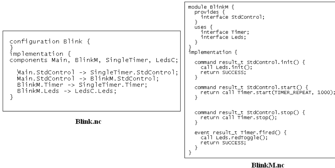
Figura 2.14 – Exemplo de aplicação desenvolvida utilizando NesC e componentes do TinyOS.
