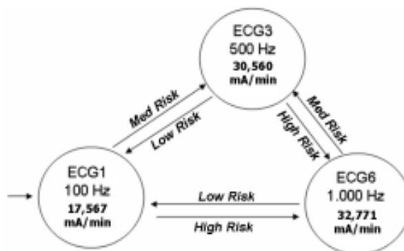
Figura 3.13 – Uma implementação do EPSM para um nó sensor de ECG multifuncional (BARBOSA et al. , 2006).
