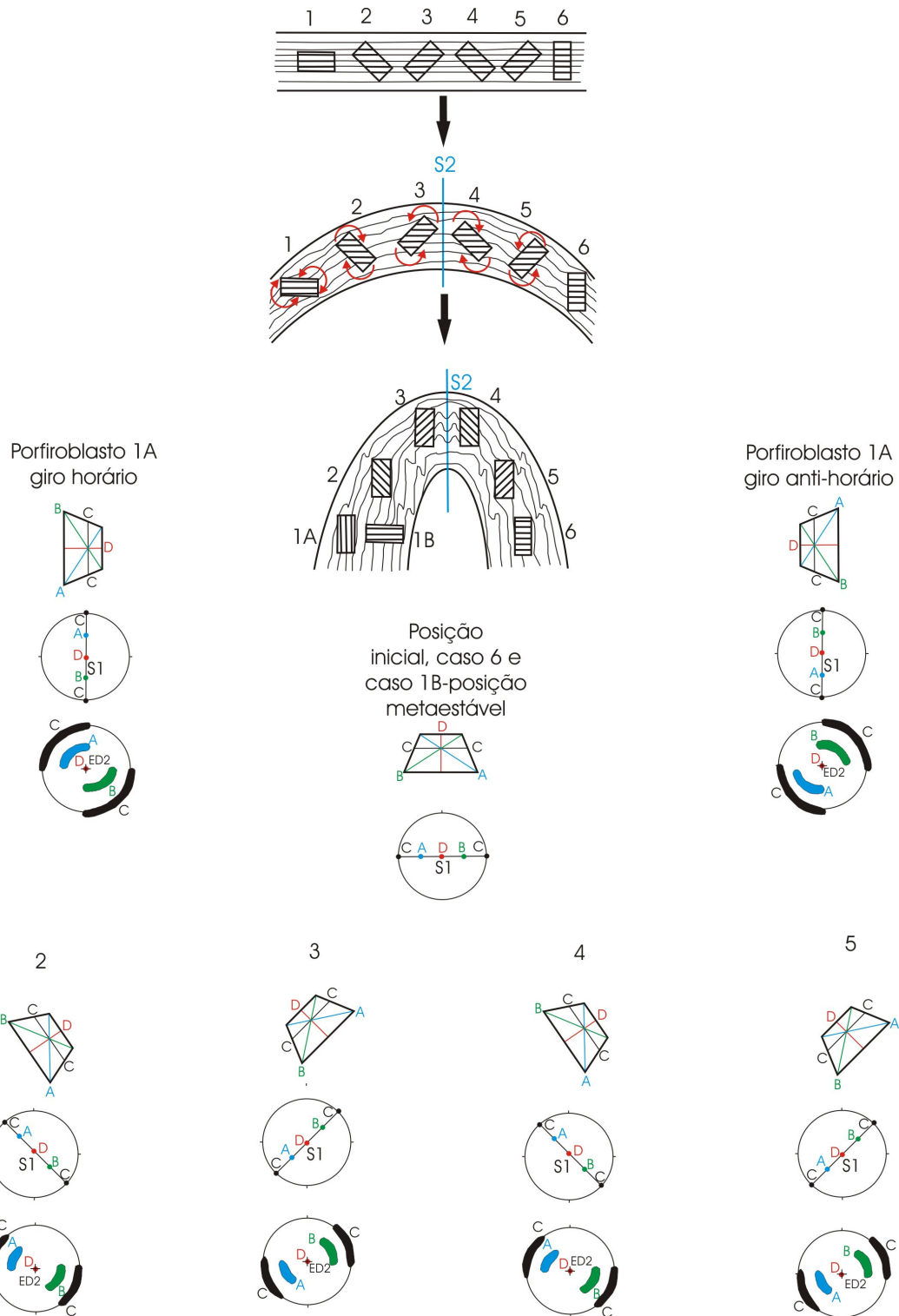
Figura 2.8 - Exemplo teórico do comportamento de porfiroblastos inequidimensionais em dobramento por cisalhamento puro.
