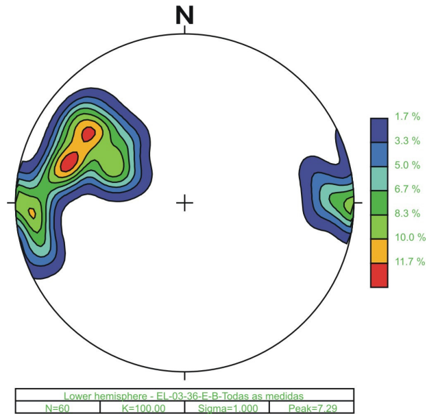
Figura 5.2 – Dispersão dos dados de L1 no espaço, medidos na lâmina EL-03-36-E-B.
