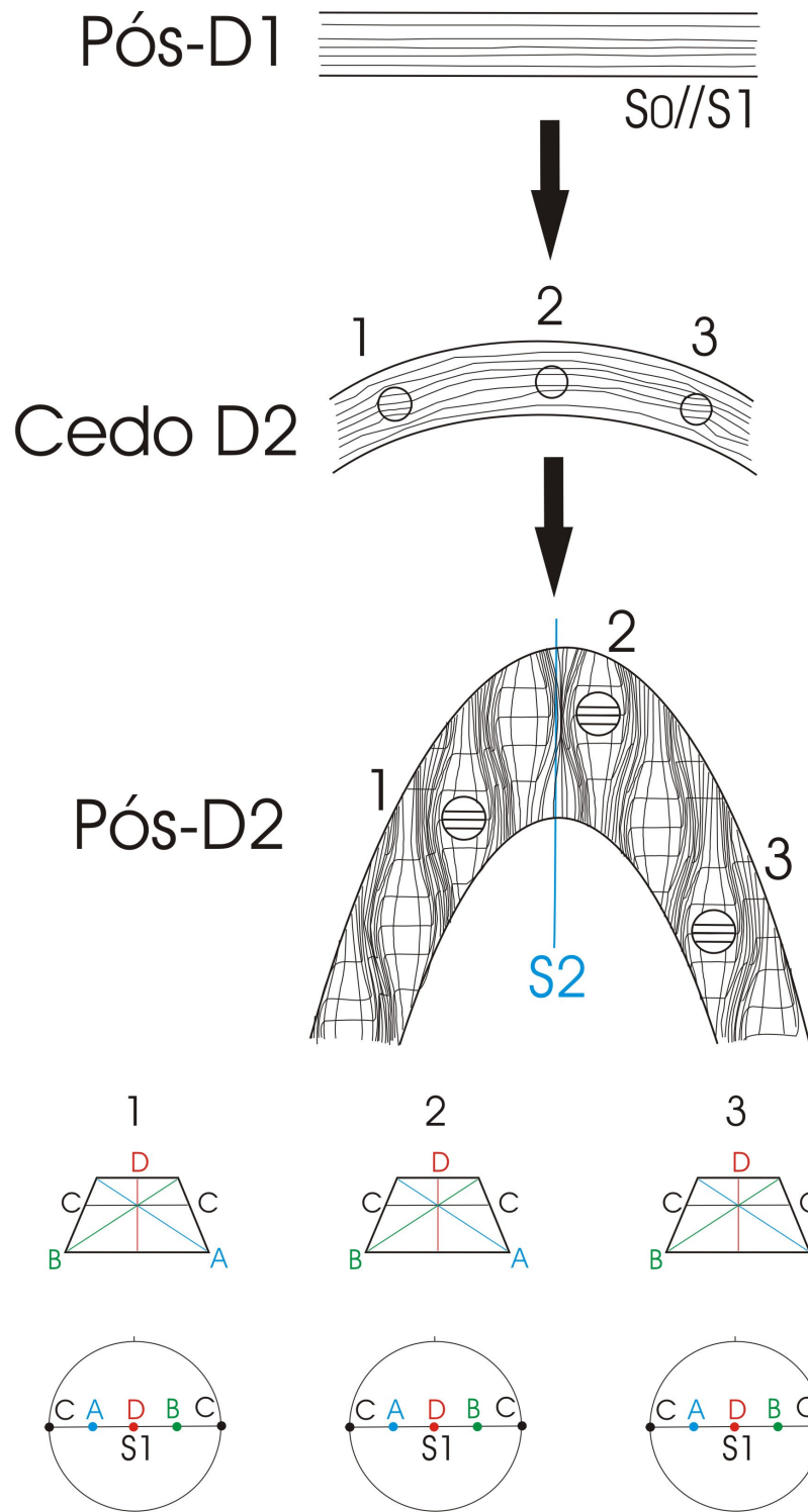
Figura 2.19 - Geometria de inclusões de porfiroblastos esféricos sin D2. O mecanismo de dobramento considerado é o da partição da deformação nos planos de S_2 .
