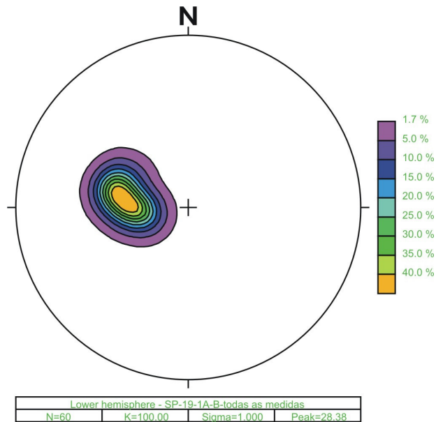
Figura 5.12 - Dispersão dos dados de L1 no espaço, medidos na lâmina SP-19-1A-B.
