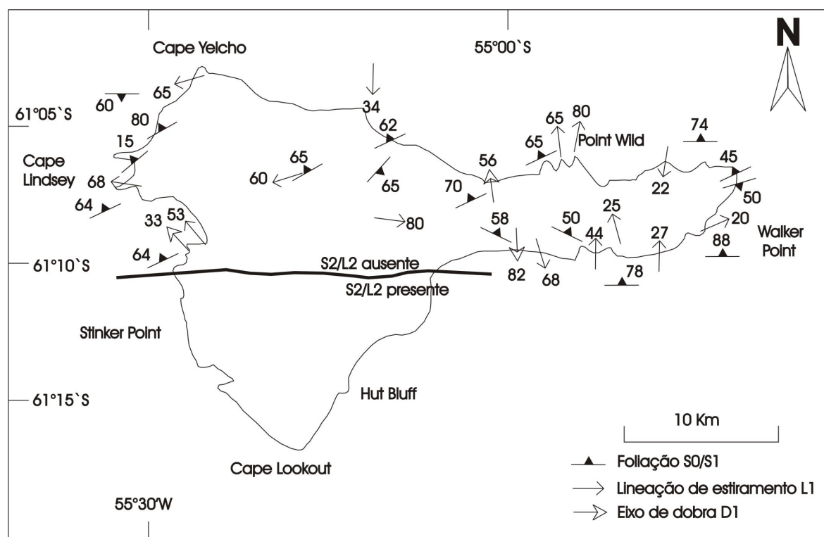
Figura 4.2 – Mapa estrutural da Ilha Elefante, destacando as estruturas D1, dominantes no norte da ilha. Adaptado de TROUW et al. (2000) e GRUNOW et al. (1992).
