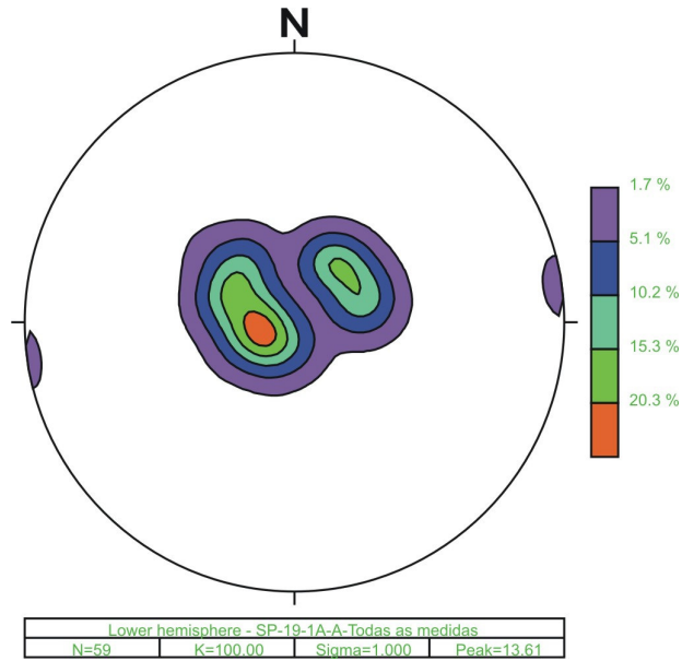
Figura 5.11 - Dispersão dos dados de L1 no espaço, medidos na lâmina SP-19-1A-A.
