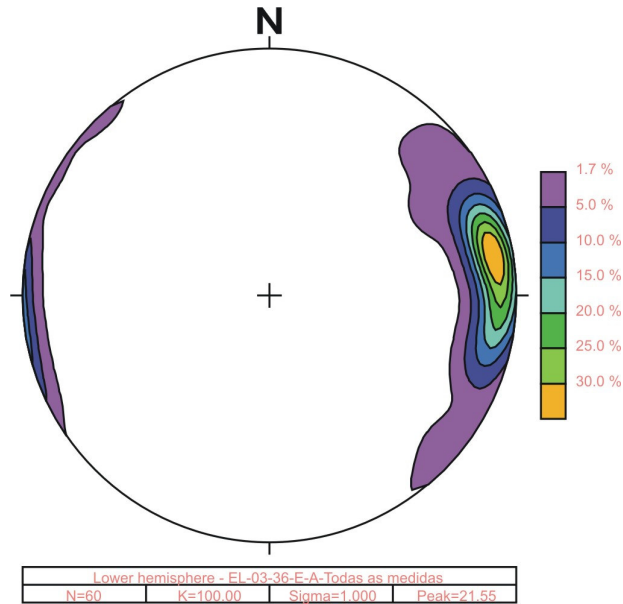
Figura 5.1 – Dispersão dos dados de L1 no espaço, medidos na lâmina EL-03-36-E-A.
