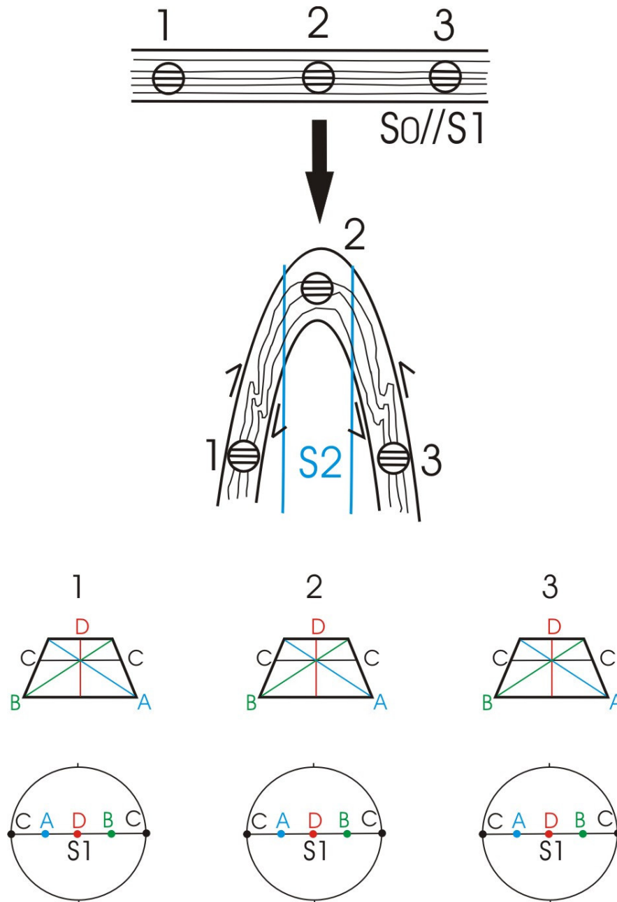
Figura 2.6 – Exemplo teórico do comportamento de porfiroblastos esféricos em dobramento por fluxo flexural. Como neste modelo tais porfiroblastos não se movimentam em relação a S2, as lineações inclusas tendem a manter sua orientação original.
