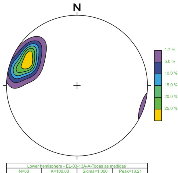
Figura 5.3 – Dispersão dos dados de L1 no espaço, medidos na lâmina EL-03-13A-A.
