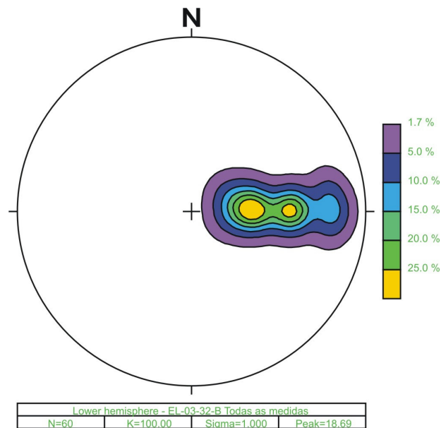
Figura 5.8 - Dispersão dos dados de L1 no espaço, medidos na lâmina EL-03-32-B.
