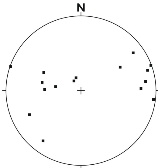
Figura 5.17 – Estereograma das medidas de lineações inclusas em Stinker Point.
