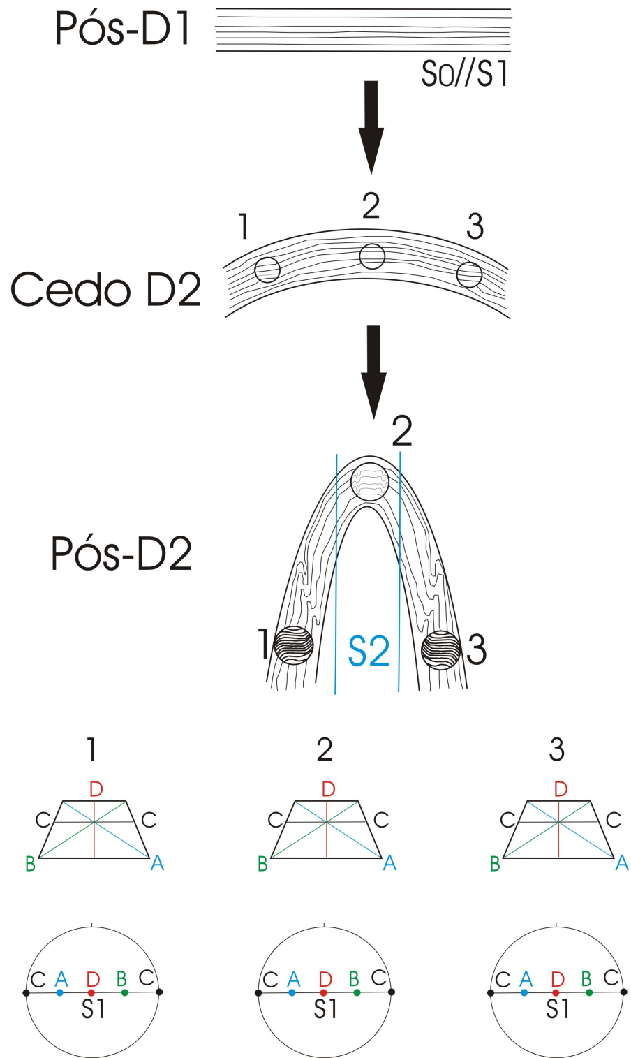
Figura 2.17 - Geometria de inclusões de porfiroblastos esféricos inter a sin D2. O mecanismo de dobramento considerado é o de cisalhamento puro.
