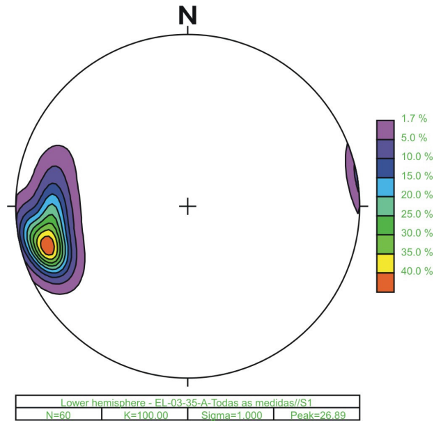
Figura 5.15 - Dispersão dos dados de L1 no espaço, medidos na lâmina EL-03-35A, nos porfiroblastos paralelos a S1.
