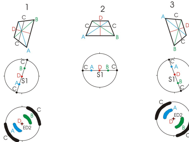
Figura 2.3 – Exemplo de ilustração utilizada para discutir o comportamento de lineações em porfiroblastos com deformações associadas a dobras. Corte idealizado em três porfiroblastos, onde pode ser visualizada a superfície de S_i com quatro possíveis orientações de L_i e os estereogramas representando as posições finais de cada uma das lineações. O porfiroblasto 2, neste caso não rotaciona, e qualquer lineação inclusa irá manter a sua orientação original.
