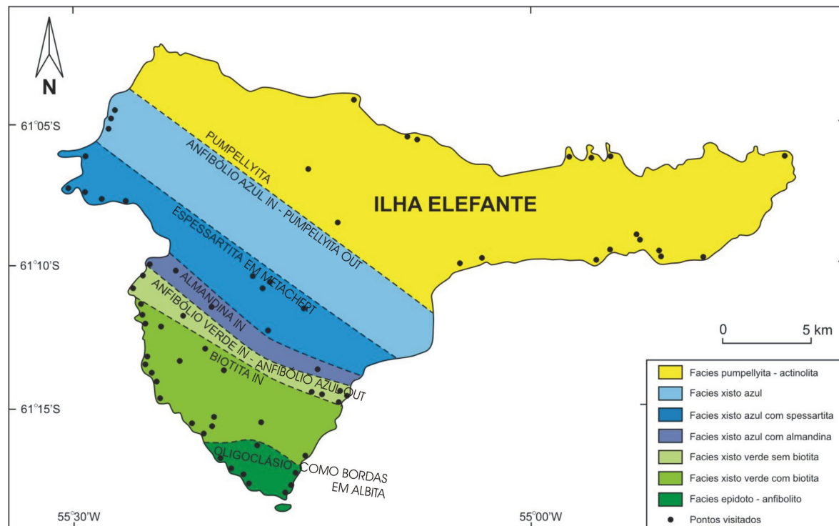
Figura 4.8 – Mapa metamórfico da Ilha Elefante mostrando o aumento das isógradas de nordeste para sudoeste. Extraído de TROUW et al. (1998b).
