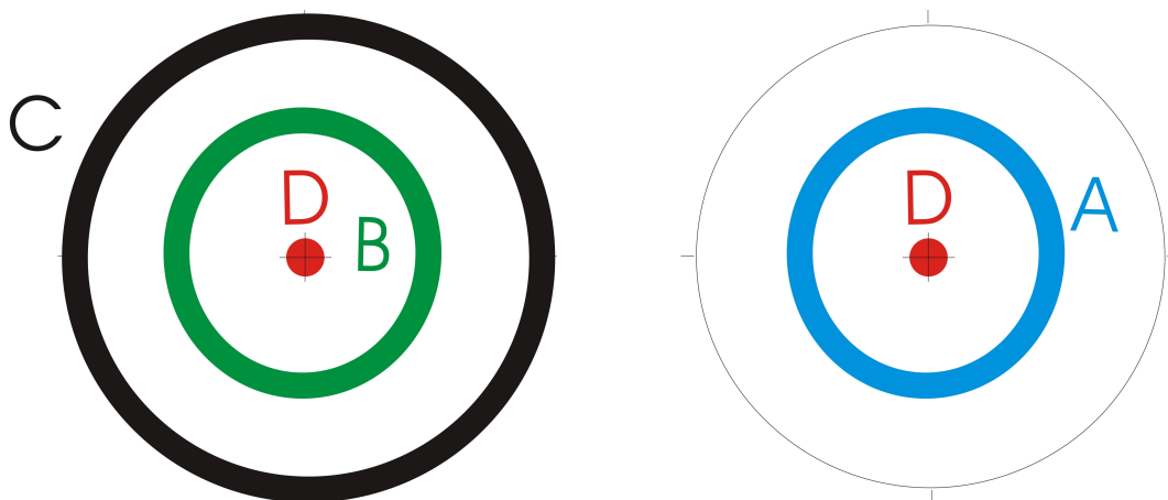
Figura 6.2 - Estereograma ilustrando a rotação das quatro posições iniciais (referidas na figura 2.3) da lineação incluída em um porfiroblasto. Neste caso, cisalhamento não coaxial sem dobra, a única direção que não gera guirlandas é uma paralela ao eixo de rotação, que corresponde ao eixo de vorticidade.
