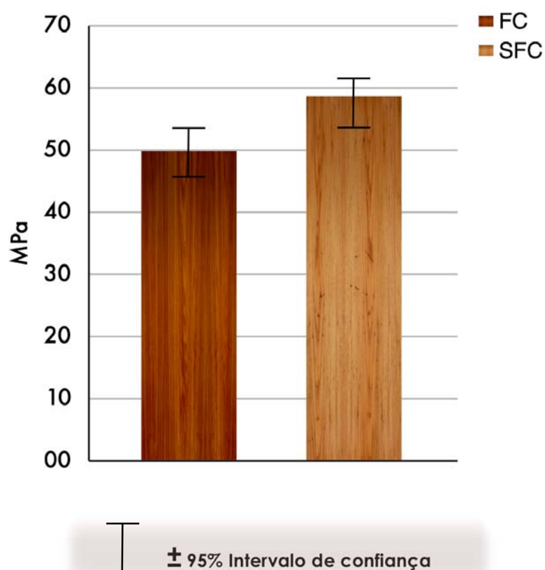
Gráfico 1 - Valores de resistência de união à microtração dos grupos testados.
