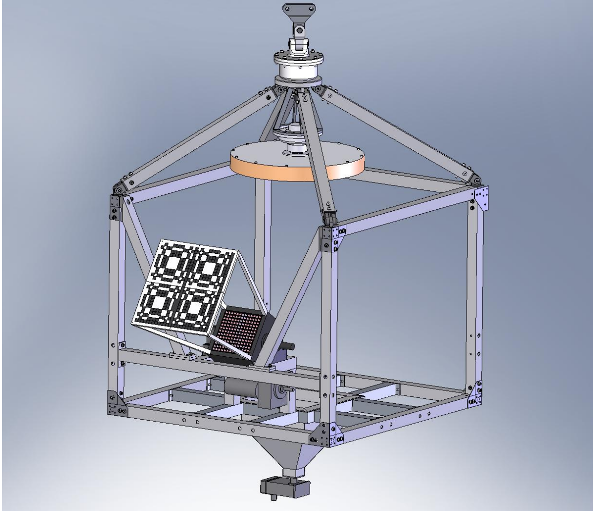
Figura 4.3 - Gôndola de balão.
