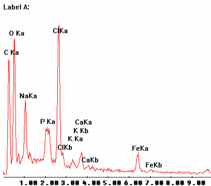
Figura 29- Espectro de espectroscopia de energia dispersiva dos filmes de amido/sorbitol/polipirrol após 3 dias imersão em SBF.
