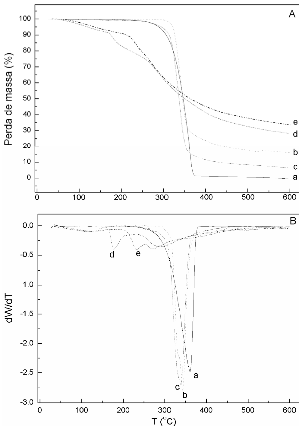
Figura 20- A ) Curvas de TG e B) curvas de DTG de: a) sorbitol; b) filme de amido de milho; c) filme de amido contendo 20% m/v de sorbitol; d) filme de amido contendo 20% m/v de sorbitol e 5% m/v de FeCl 3 .6H 2 O; e) filme de amido contendo 20% m/v de sorbitol e 5% m/v de FeCl 3 .6H 2 O após 24h de exposição aos vapores de pirrol.
