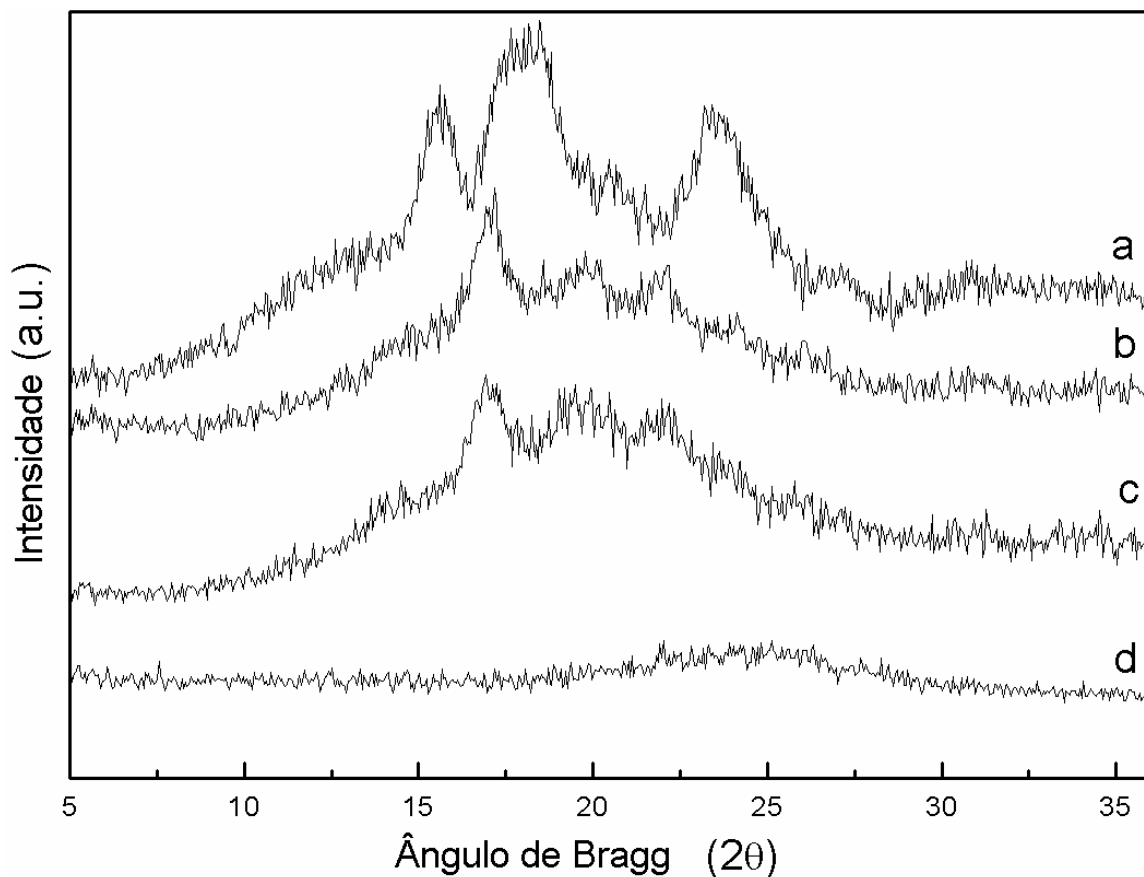
Figura 19- Difratograma de raios-x de: a) amido de milho (pó in natura); b) filme de amido contendo 20% m/v de sorbitol e 5% m/v de FeCl 3 .6H 2 O; c) filme de amido contendo 20% m/v de sorbitol e 5% m/v de FeCl 3 .6H 2 O após 24h de exposição aos vapores de pirrol; d) polipirrol (pó).
