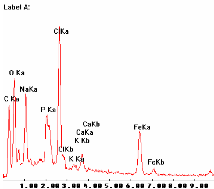
Figura 28- Espectro de espectroscopia de energia dispersiva dos filmes de amido/sorbitol/polipirrol após 1 dia imersão em SBF.
